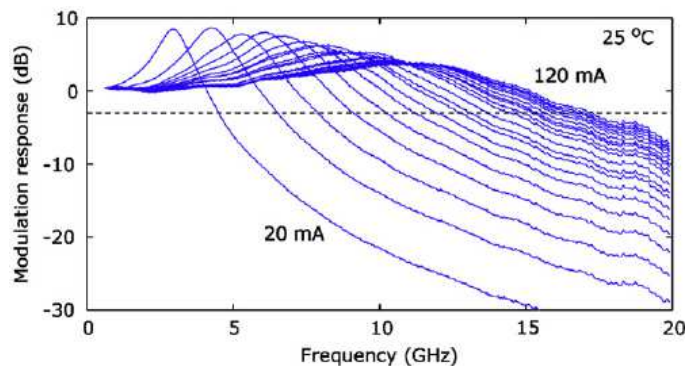
Figure 2.5 : Exemple de réponse en modulation pour plusieurs courants d'injection à température ambiante d'une diode laser à 1,3 \mu\text{m} [Wan09]
