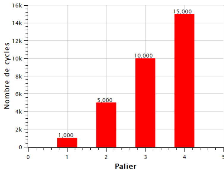
Figure 111 : Conditions des surcharge en courant par palier. Chaque palier présente une crête de courant demi-sinusoidale à 7 \times I_N .
