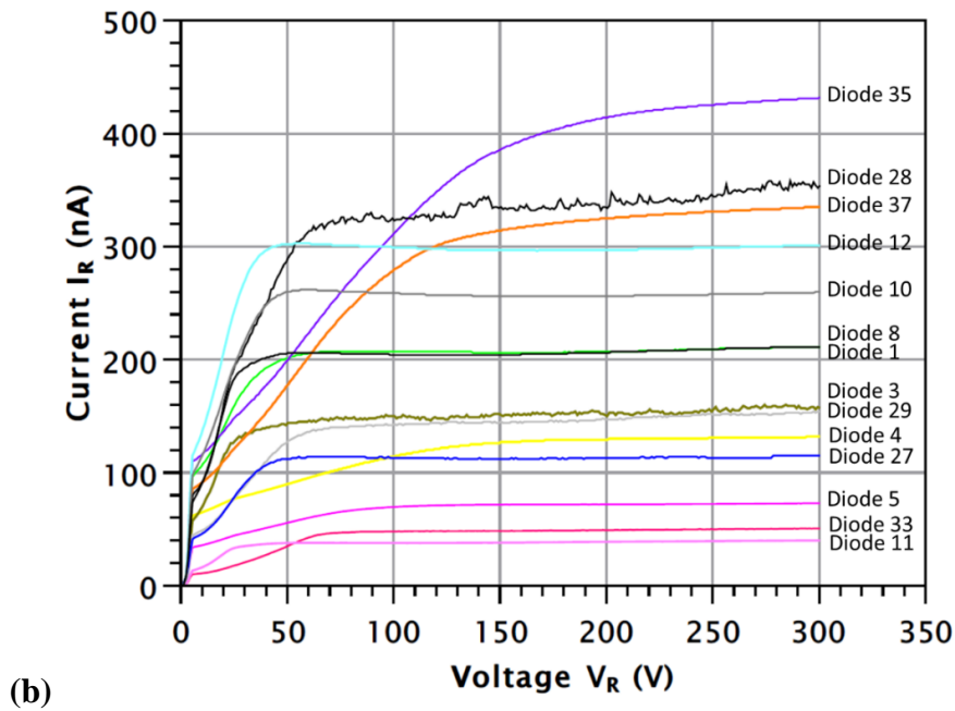
Figure 72 : Mesures en inverse pour les diodes (a) 2,6,7 et 9, (b) diodes restantes de 1 à 35 (B1505A).
