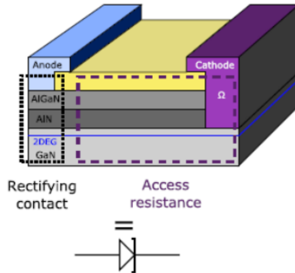
Figure 23 : Coupe verticale d'une diode Schottky AlGaN/GaN telle que l'anode est un contact Schottky et le contact ohmique est la cathode [43].
