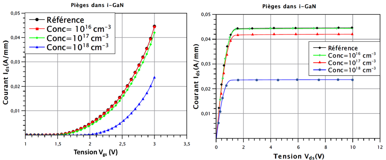
Figure 59 : Caractéristiques de transfert et de sortie du GIT en fonction de la concentration des pièges.
