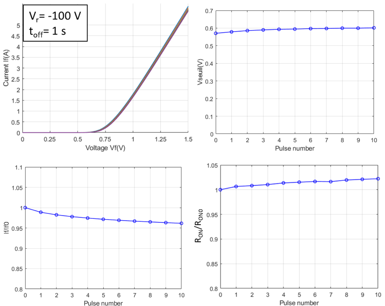
Figure 80 : Application de 10 impulsions de stress quasi-statique pour V_{D-off} = -100 V et t_{off} = 1 s.
