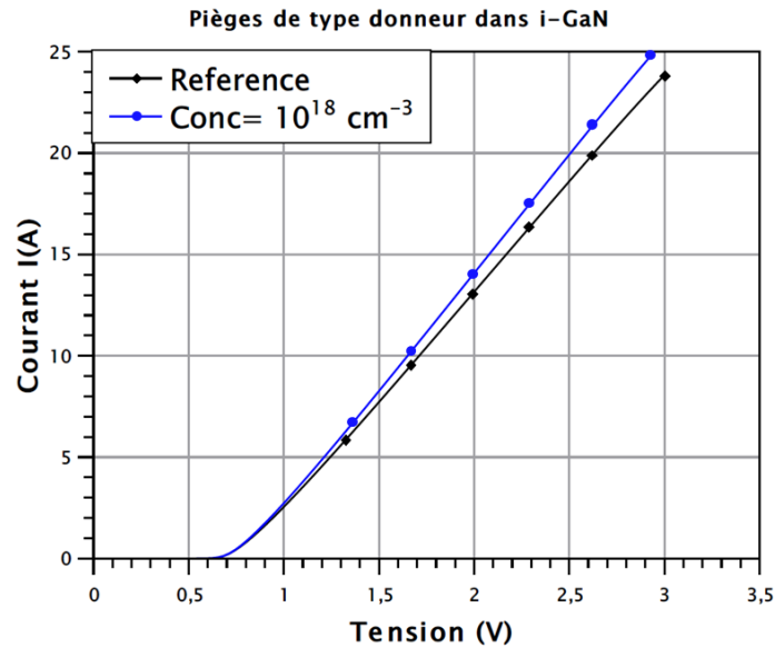
Figure 58 : Influence des pièges de type n localisés dans i-GaN sur les caractéristiques en direct de la diode.
