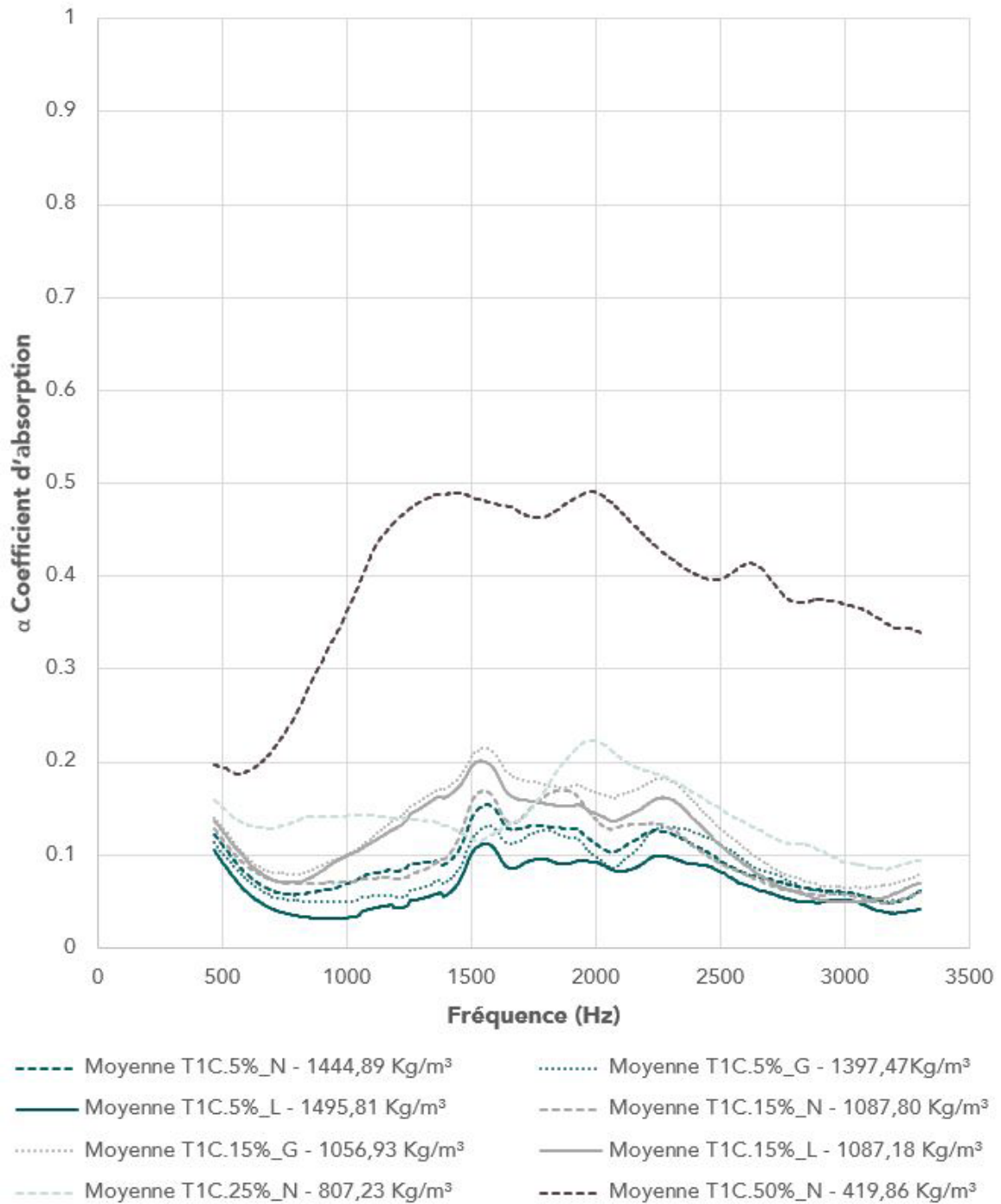
Figure 329 Coefficient d'absorption - Terre 1 - Chanvre
