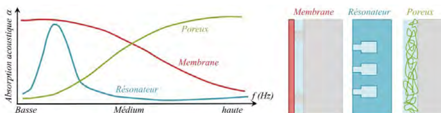
Figure 39 Game d'efficacité - trois types de matériaux absorbants (DE SA et Horsin Molinaro, 2017).
