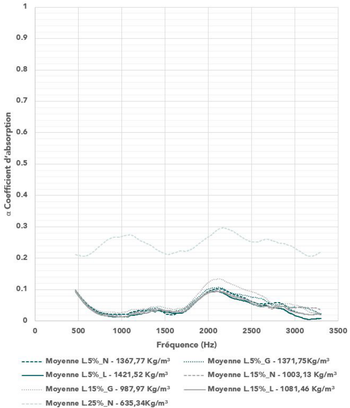
Figure 333 Coefficient d'absorption - Terre 1- Lin
