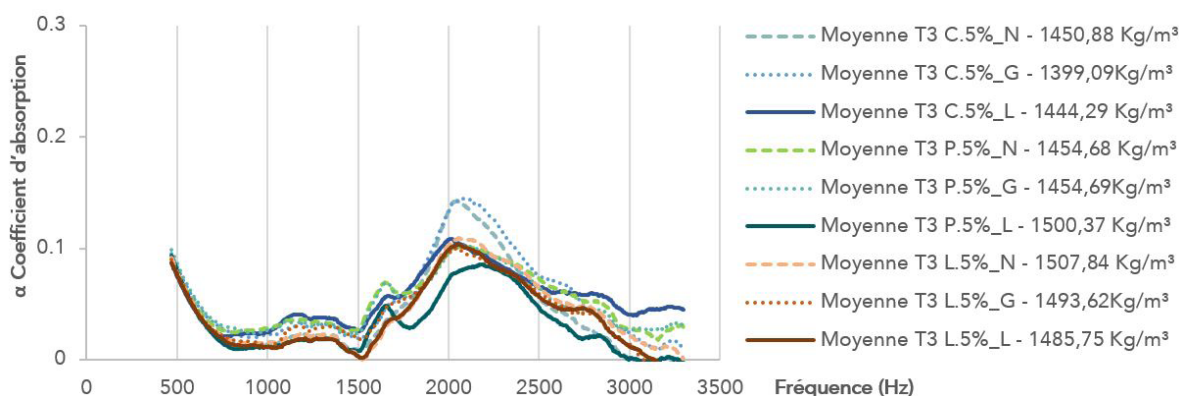
Figure 128 Valeurs d'absorption acoustique des échantillons avec la terre 3 et 5% de fibres.
