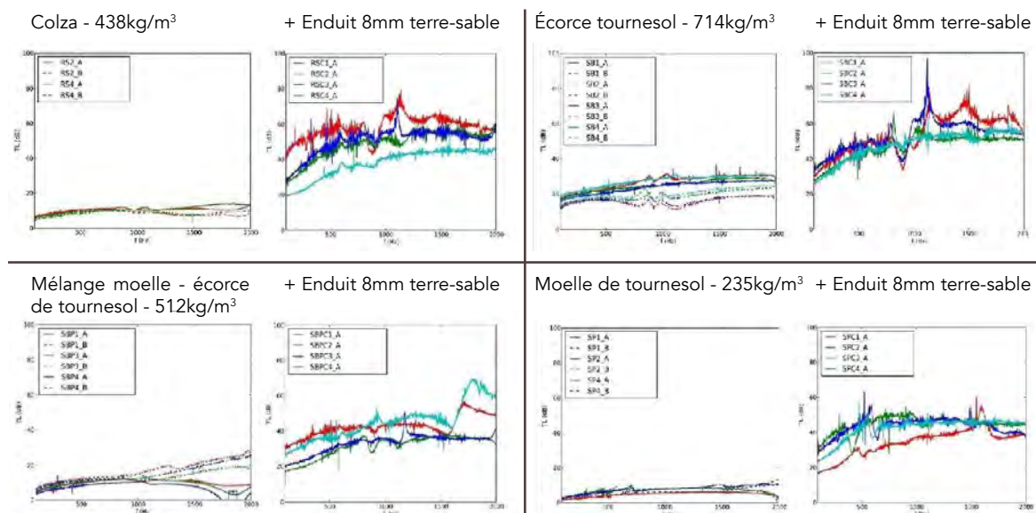
Figure 6 Perte de transmission TL (en tube de Kundt) de quatre composites de terre allégée différentes sans et avec enduit en terre crue (Brouard, 2018).
