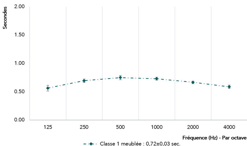
Figure 101 Moyenne du temps de réverbération (calculée à partir du T_{30} ) de la classe mesurée – Treffieux. Les barres d'erreur représentent l'écart type standard entre les différents points de mesure.
