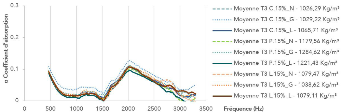
Figure 130 Valeurs d'absorption acoustique des éprouvettes avec la terre 3 et 15% de fibres.
