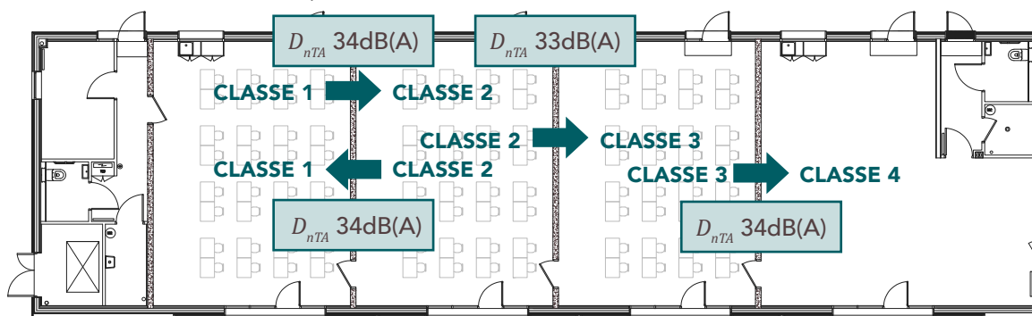
Figure 88 Isolation entre pièces à Baulon - Salles de classes non meublées.
