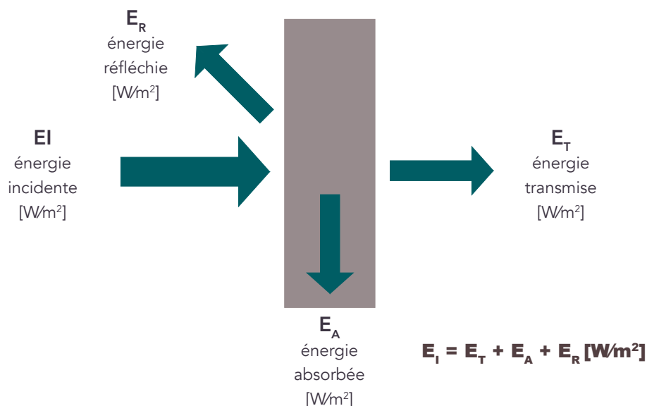
Figure 28 Distribution de l'énergie (Avilés López et Perera Martín, 2017).
