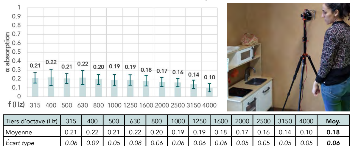
Figure 113 Mesures in situ du coefficient d'absorption acoustique (moyenne) par tiers d'octave. Enduit terre sur botte de paille
