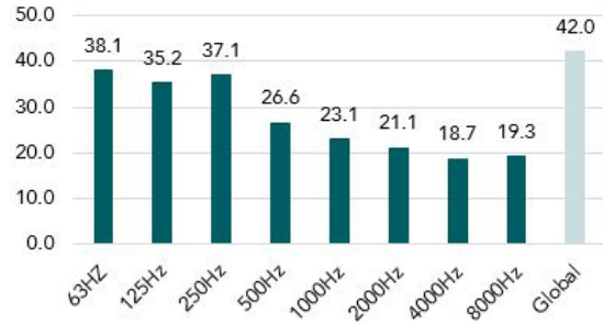
Classe 2 Meublée - Niveaux par bande et niveau global en dB(A).
