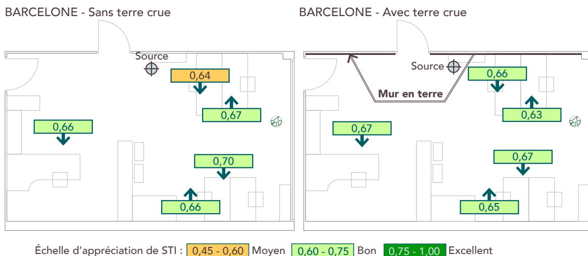
Figure 208 Valeurs d'intelligibilité à la parole - Speech transmission Index (STI) – Barcelone
