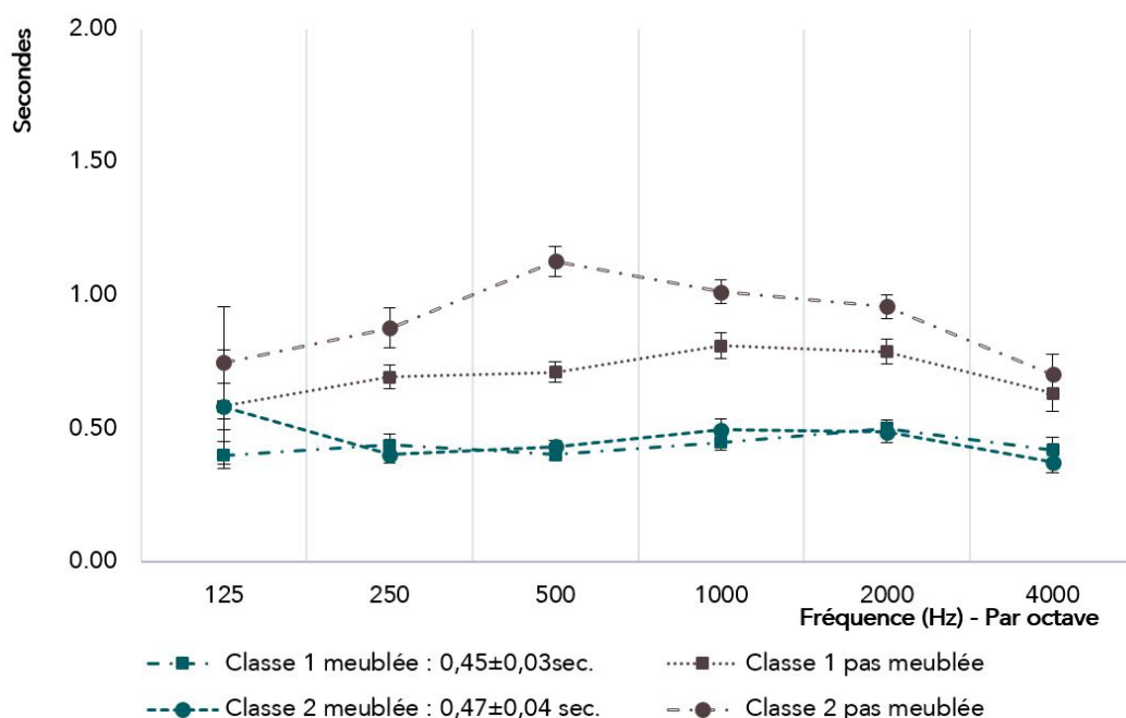
Figure 99 Moyennes des temps de réverbération (calculées à partir du T30) des différentes classes mesurées – Mouais. Les barres d'erreur représentent l'écart type standard entre les différents points de mesure.
