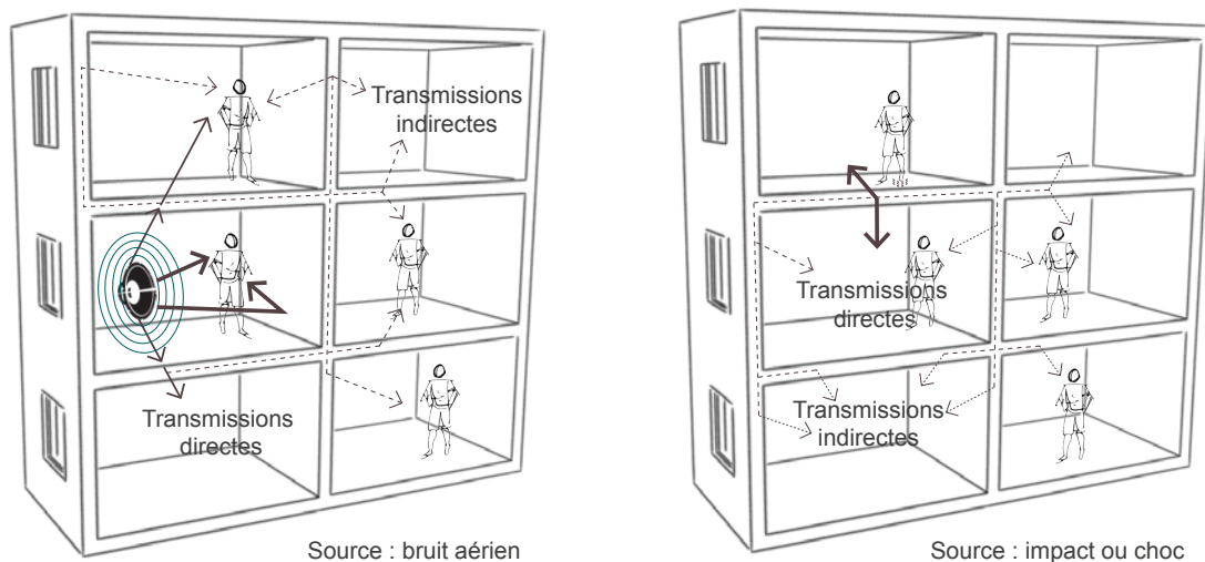
Figure 30 Génération et distribution des bruits dans les bâtiments (Saint-Gobain 2016).
