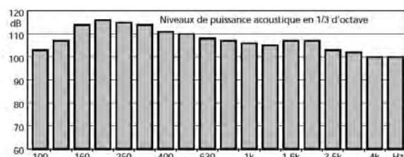
Figure 235 Niveaux de puissance acoustique maximum sur 1/3 d'octave pour l'OmniPower avec un générateur de puissance de type 2716.
