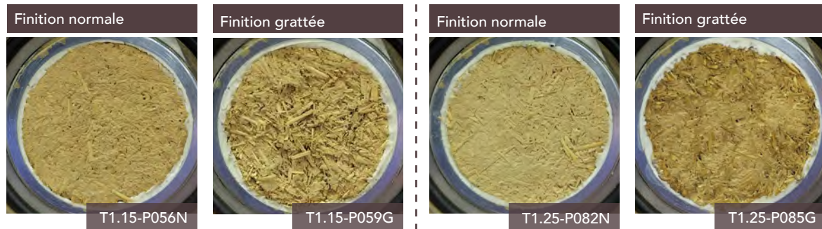
Figure 132 Aspect de surfaces des éprouvettes de la terre 1 avec 25% de paille et 15% de paille.
