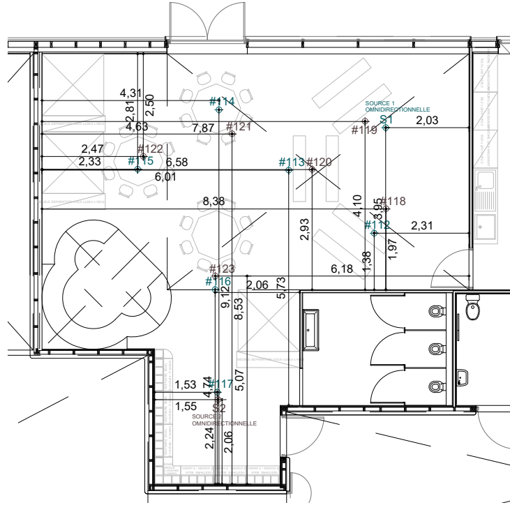
Figure 298 Positions des sources et des points de mesure – Méthode du bruit interrompu - CLASSE 3
