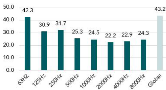
Classe 3 Pas meublée - Niveaux par bande et niveau global en dB(A).
