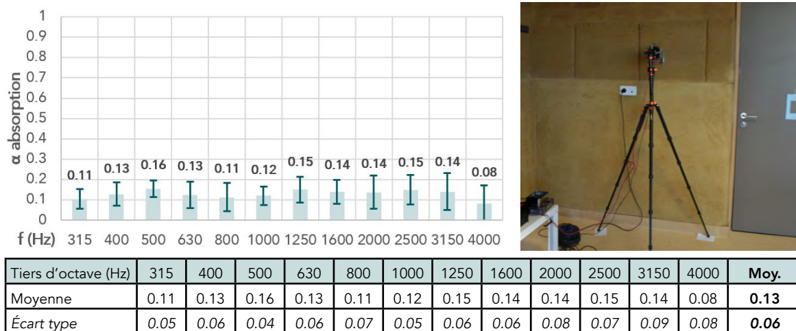
Figure 108 Mesures in situ du coefficient d'absorption acoustique (moyenne) par tiers d'octave. Mur en terre (bauge) – Partie haute du mur sans finition.
