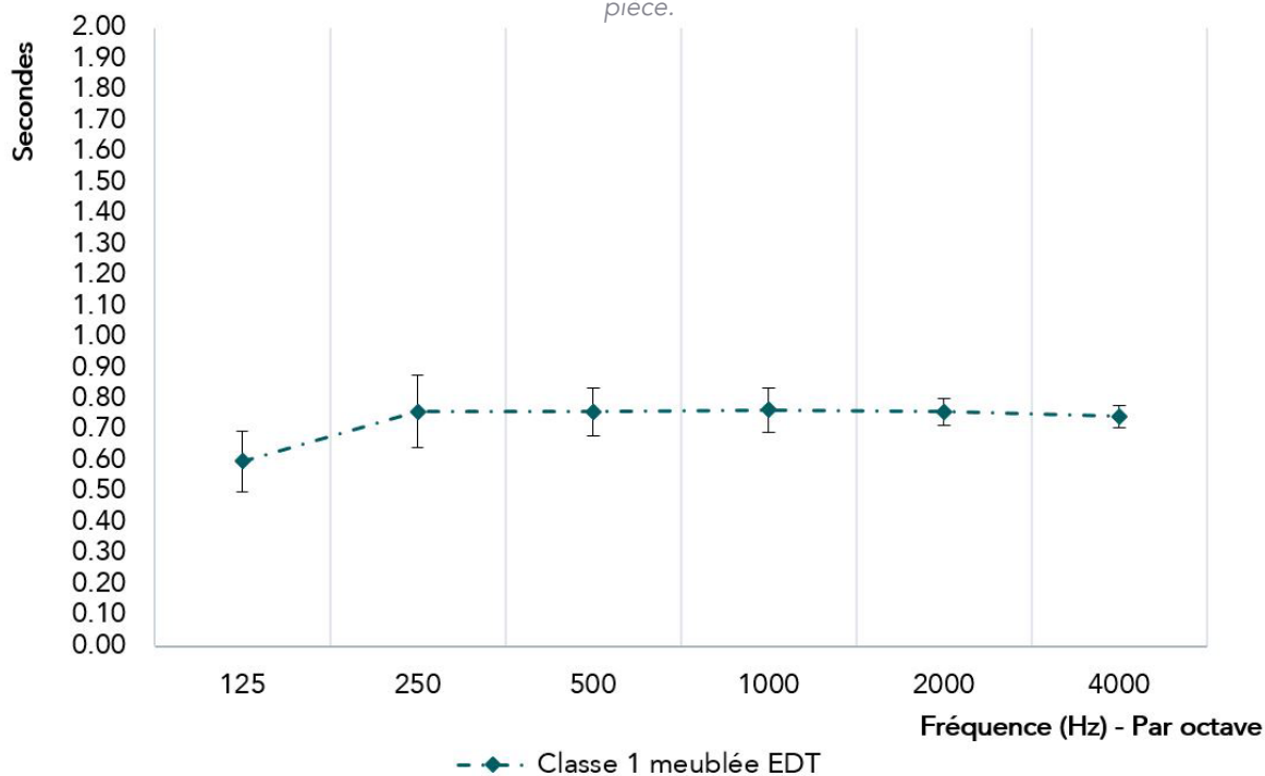
Figure 304 EDT Treffieux – Moyennes. Les barres d'erreur représentent l'écart type standard entre les différents points de mesure.
