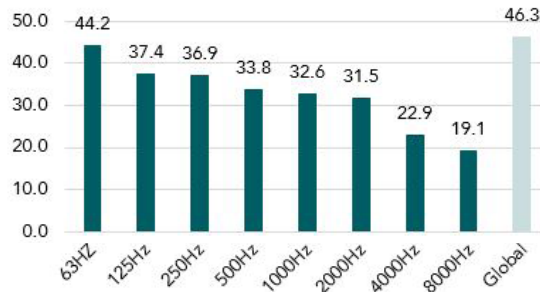
Biblio Meublée - Niveaux par bande et niveau global en dB(A).
