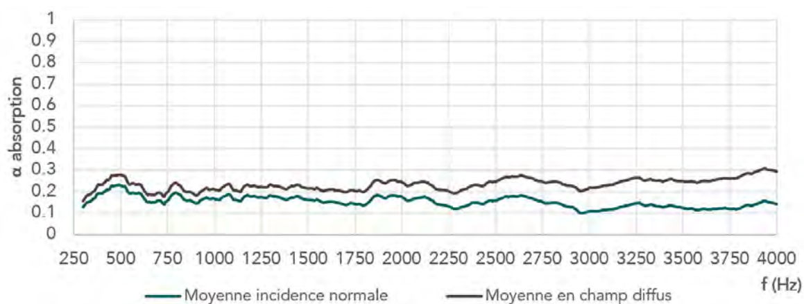
Figure 322 Comparatif entre la valeur moyenne d'absorption en incidence normale et en champs diffus. Enduit terre sur support terre-paille – Mouais.
