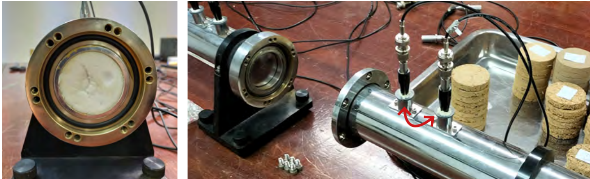
Figure 52 Calibration des microphones de mesure avec la mousse de référence.
