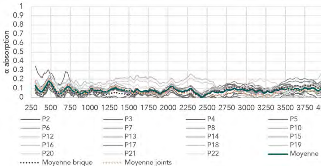
Figure 318 Mesures in situ du coefficient d'absorption acoustique en champ diffus par fréquence. Mur en brique de terre crue stabilisé à la chaux (BTC) - Fégréac.
