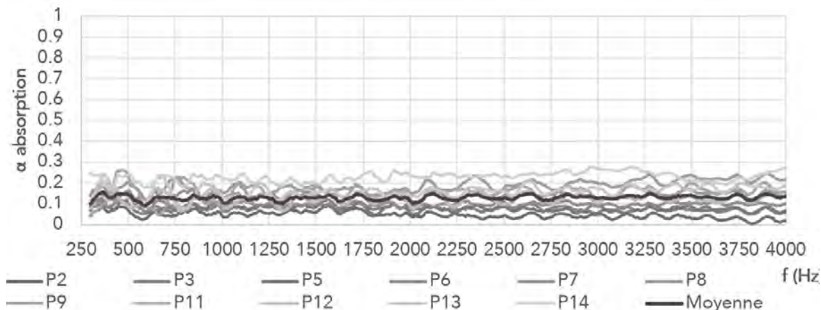
Figure 306 Mesures in situ du coefficient d'absorption acoustique en champ diffus par fréquence. Mur bauge (partie basse) – Bouvron.
