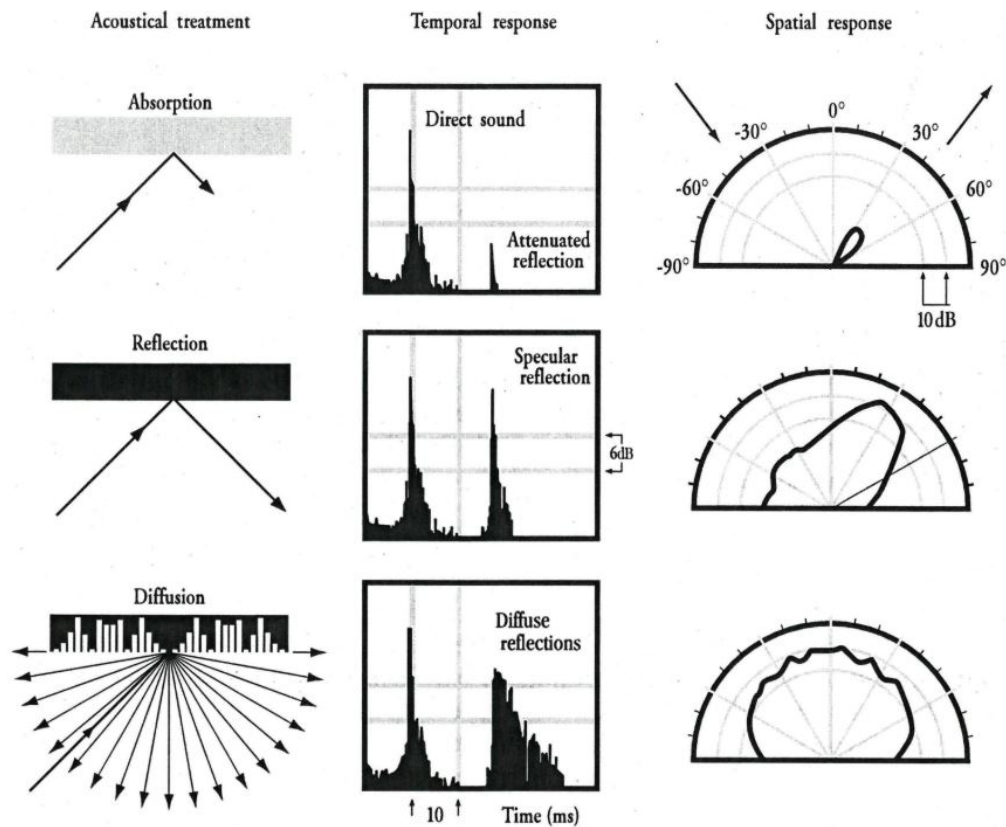
Figure 38 Phénomènes associés à la propagation du son (Cox and D'Antonio, 2009).
