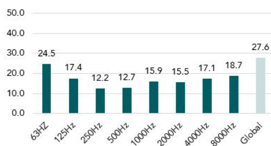
Classe 2- Niveaux par bande et niveau global en dB(A).
