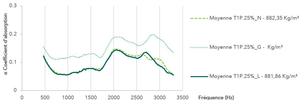
Figure 131 Valeurs d'absorption acoustique des éprouvettes avec la terre 1 et 25% de fibres.
