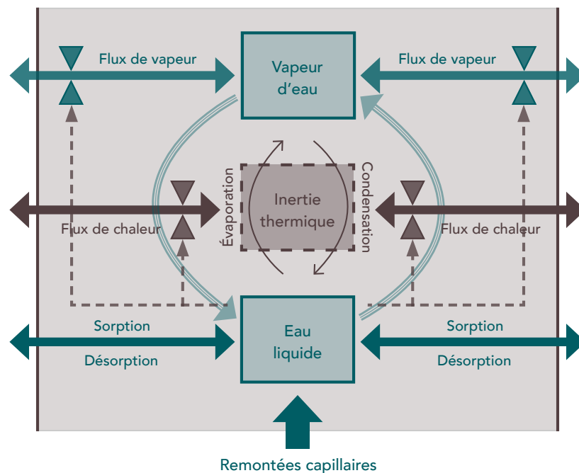
Figure 5 Couplage hygrothermique de la terre crue (Chabriac, 2014).
