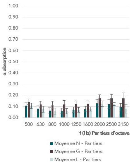
Terre 1 – 25% Paille : Par tiers d'octave
