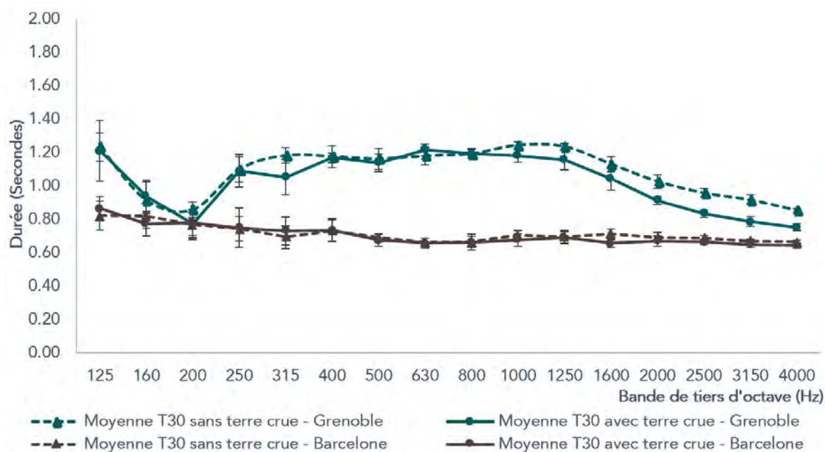
Figure 206 T30 de salles d'expérimentation de Grenoble et Barcelona avec et sans terre crue. Les barres d'erreur représentent l'écart type standard entre les différents points de mesure.
