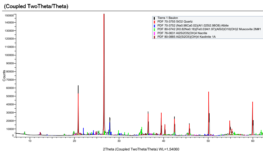
Figure 326 Diffraction des rayons X. Terre 1 - Baulon
