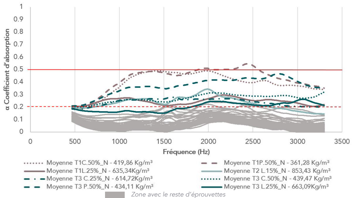
Figure 119 Valeurs d'absorption du tube de Kundt.
