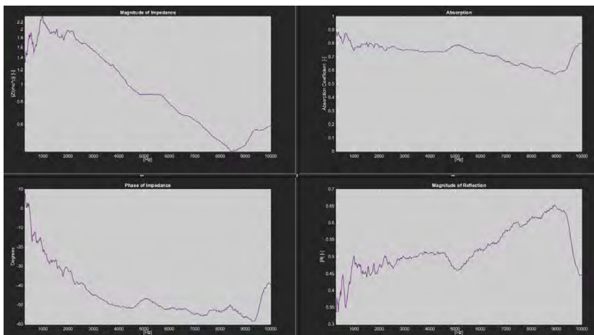
Figure 50 Exemple de mesure réalisée d'une paroi terre-chanvre. Programme : Microflown Velo 5.
