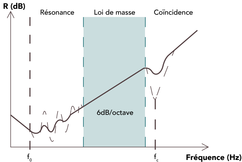
Figure 33 Indice de réduction acoustique d'une paroi simple (Avilés López et Perera Martín, 2017).
