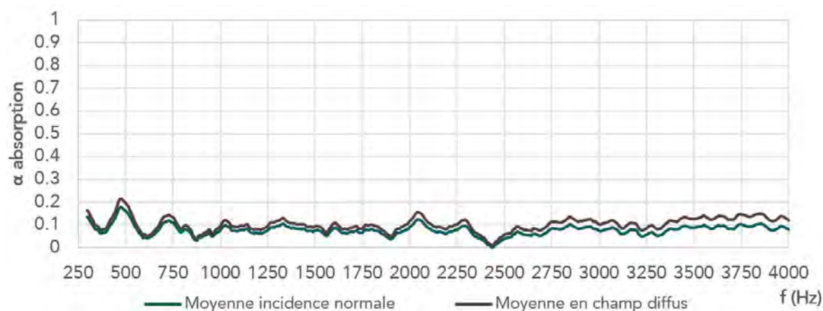
Figure 319 Comparatif entre la valeur moyenne d'absorption en incidence normale et en champs diffus Mur en brique de terre crue stabilisé à la chaux (BTC) - Fégréac.
