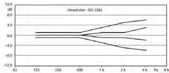
Figure 238 Directivité pour OmniPower selon la norme ISO3382 : déviation maximale de la moyenne pour un arc de 30° «glissant». Les courbes supérieures et inférieures sont les tolérances ISO3382.
