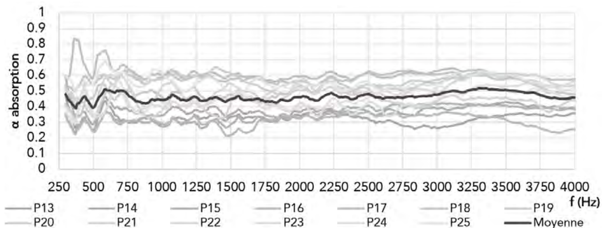
Figure 312 Mesures in situ du coefficient d'absorption acoustique en champ diffus par fréquence. Mur en terre et chanvre (torchis) – Baulon.
