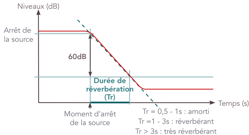
Figure 37 Durée de réverbération (Saint-Gobain 2016).
