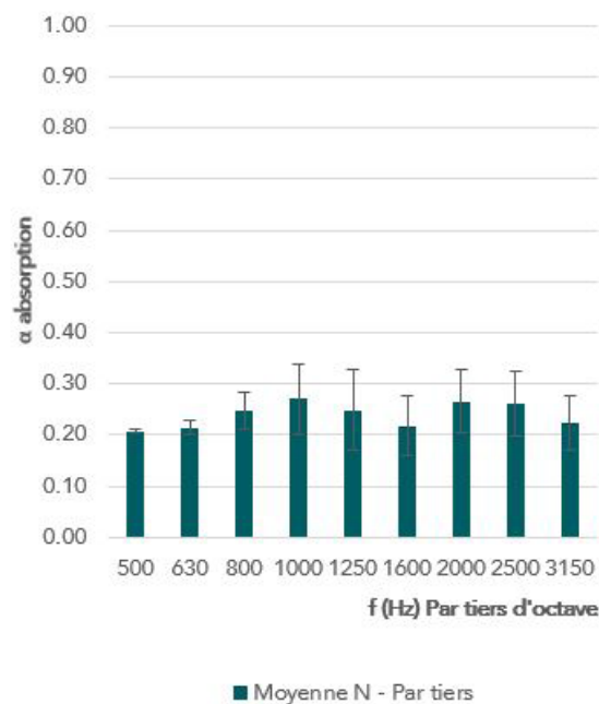
Terre 1 – 25% Lin : Par tiers d’octave
