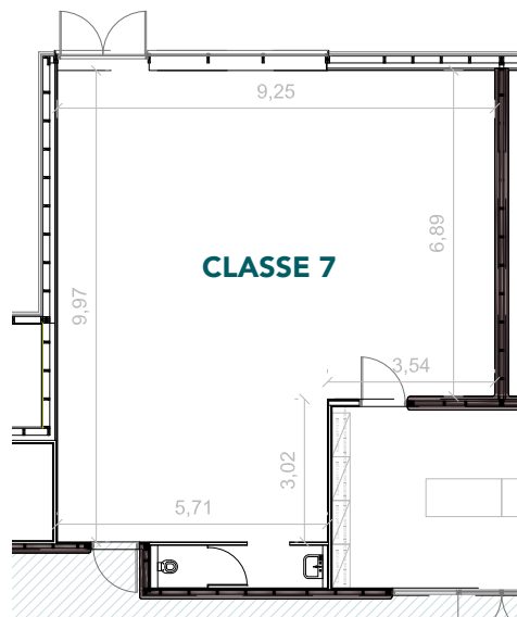
Figure 55 Plan courant de la salle de classe et vue 3D – Bouvron.
