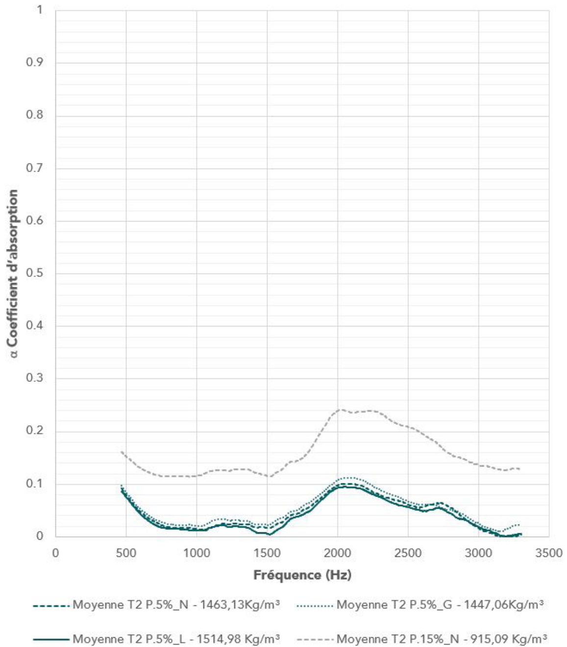
Figure 337 Coefficient d'absorption - Terre 2 – Paille
