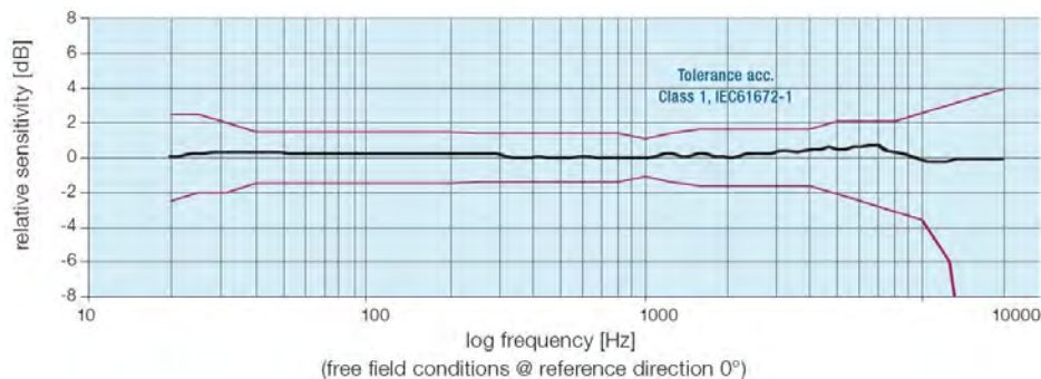
Figure 240 Réponse en fréquence typique du microphone.
