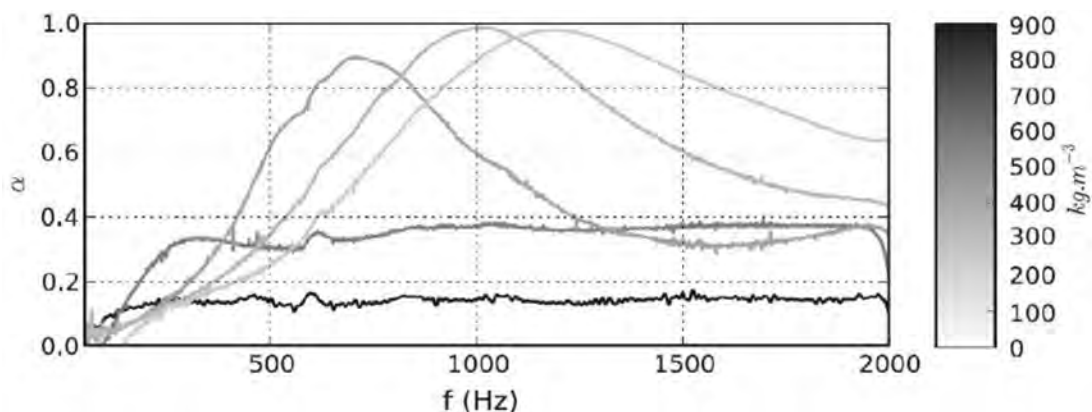
Figure 9 Coefficients d'absorption (en tube de Kundt) de terre-chanvre avec densités de 229, 306, 386, 517 et 821 \text{kg}\cdot\text{m}^{-3} (Degrave-Lemeurs, Glé and Hellouin de Menibus, 2018).
