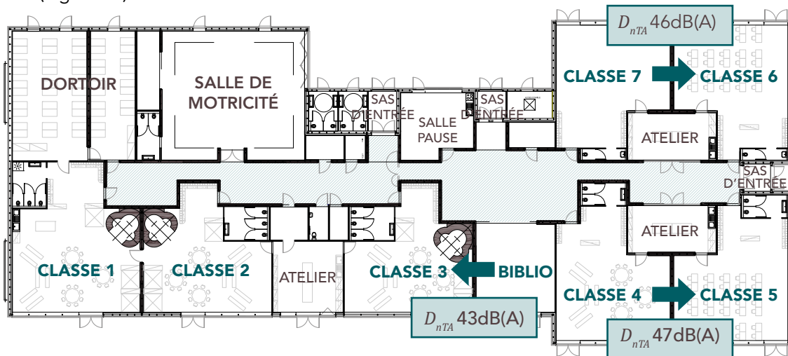
Figure 86 Isolation entre pièces à Bouvron.
