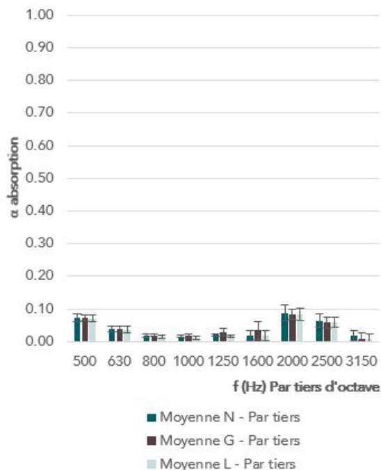
Terre 3 – 25% Lin : Par tiers d'octave
