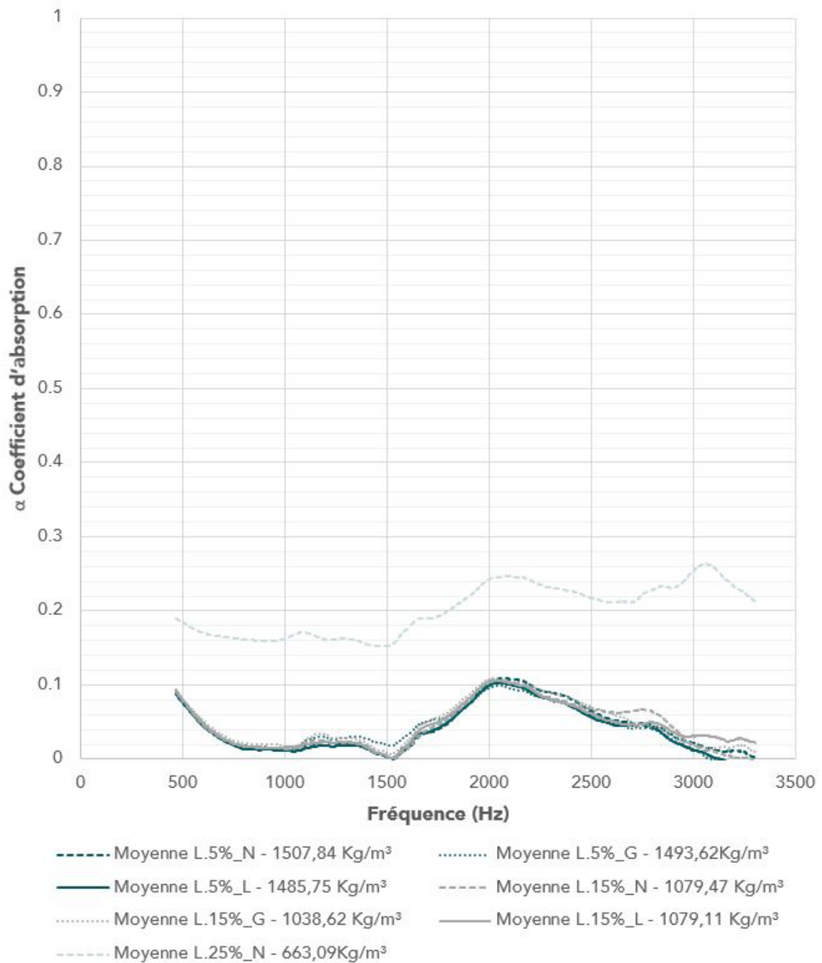
Figure 345 Coefficient d'absorption - Terre 3 - Lin
