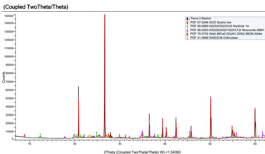
Figure 327 Diffraction des rayons X. Terre 3 - Baulon
