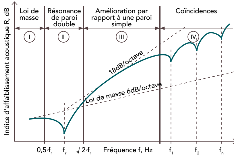
Figure 34 Tracé qualitatif de l'isolement d'une double paroi en fonction de la f_r (Zürcher et Thomas, 2014).
