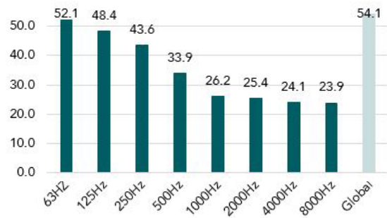
Classe 4 Pas meublée - Niveaux par bande et niveau global en dB(A).
