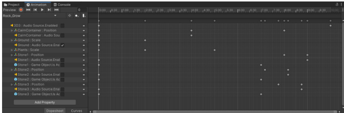
Figure 260 Fenêtre Animation.
