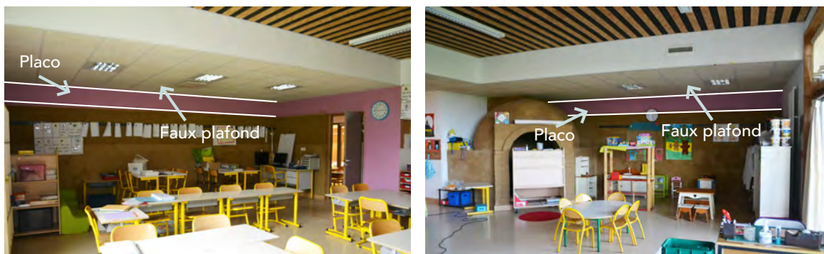
Figure 87 Points du passage du son principalement remarquables.
