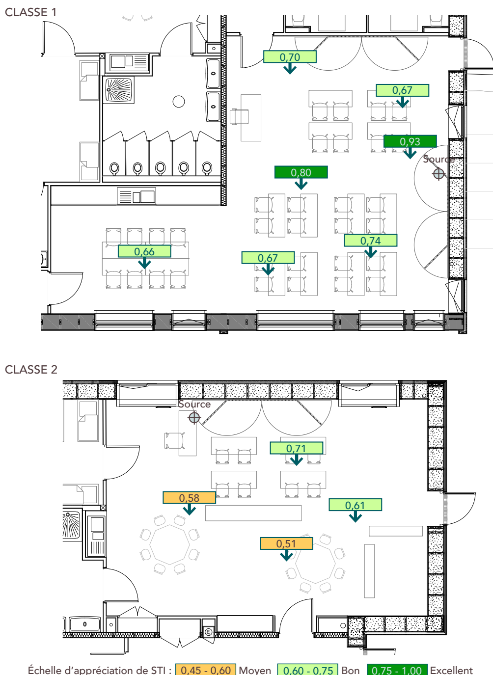
Figure 105 Valeurs d'intelligibilité à la parole - Speech transmission Index (STI) – Salles de classe de Mouais.
