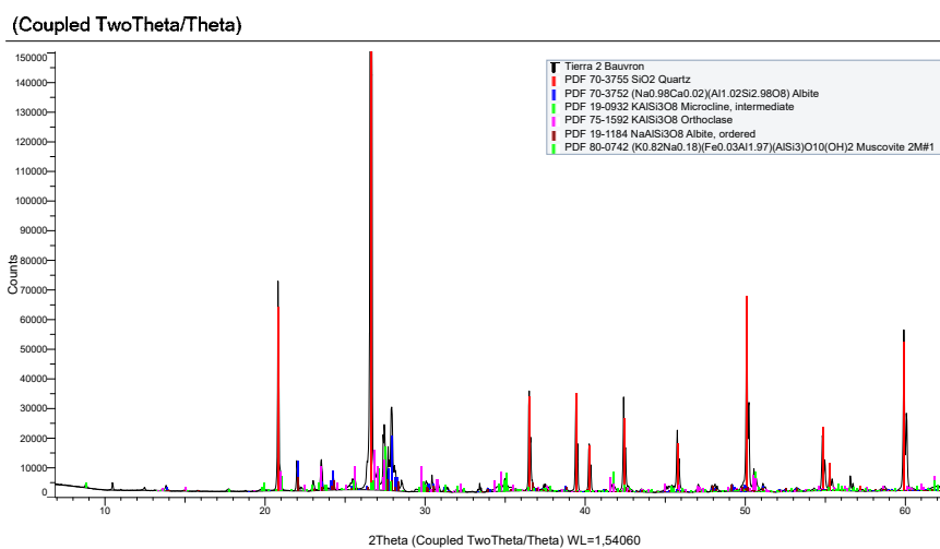
Figure 328 Diffraction des rayons X. Terre 2 - Bouvron
