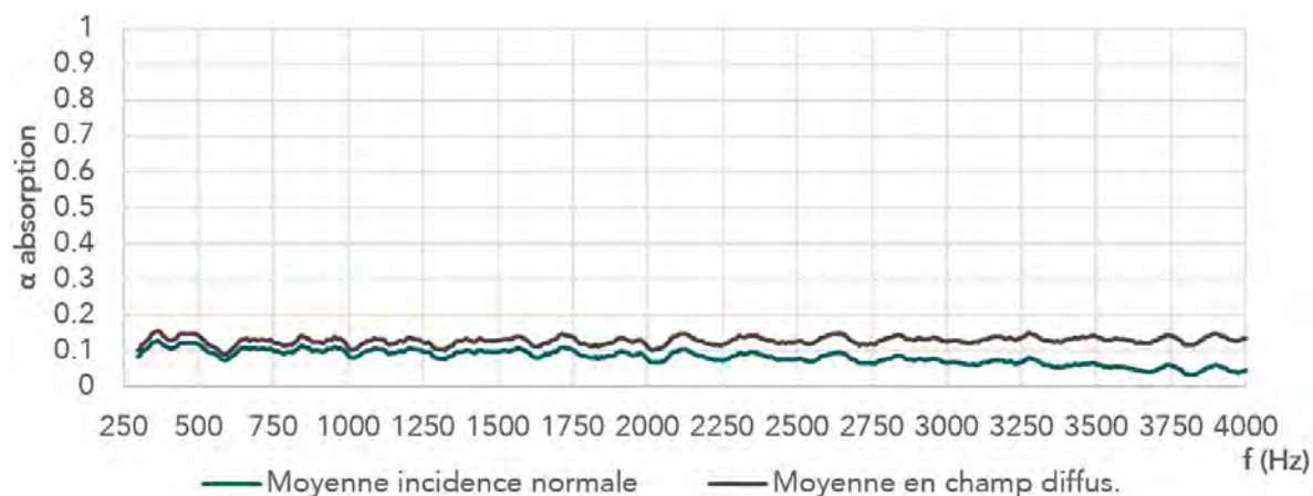
Figure 307 Comparatif entre la valeur moyenne d'absorption en incidence normale et en champs diffus. Mur en bauge (partie basse) – Bouvron.
