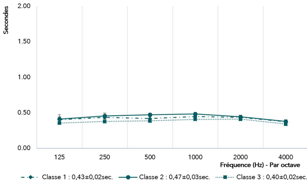
Figure 97 Moyennes des temps de réverbération (calculées à partir du T30) des différentes classes mesurées – Fégréac. Les barres d'erreur représentent l'écart type standard entre les différents points de mesure.
