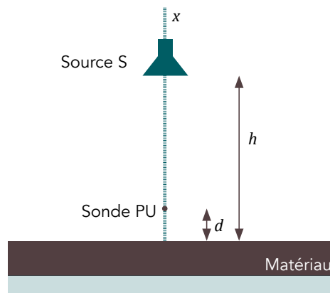
Figure 47 Schéma de la configuration de mesure avec la méthode impulsionnelle sous incidence normale (Benoit, 2013).
