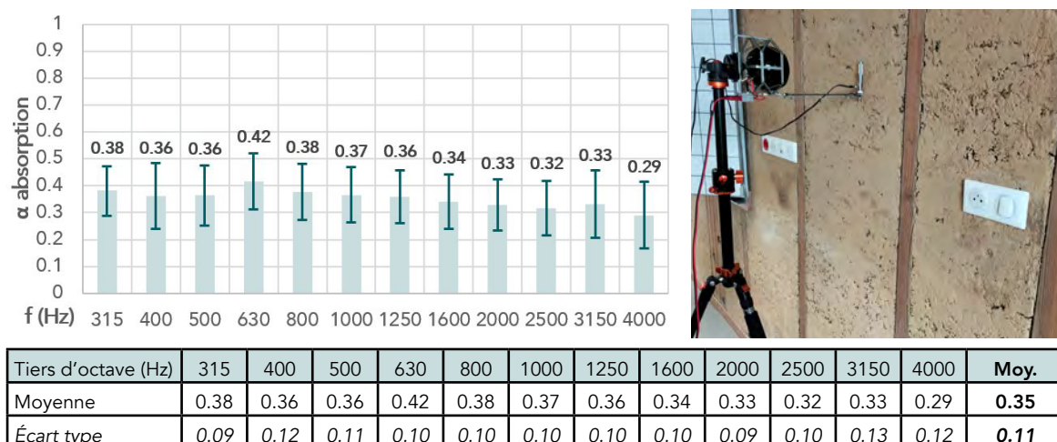
Figure 109 Mesures in situ du coefficient d'absorption acoustique (moyenne) par tiers d'octave. Mur en terre et chanvre (torchis).
