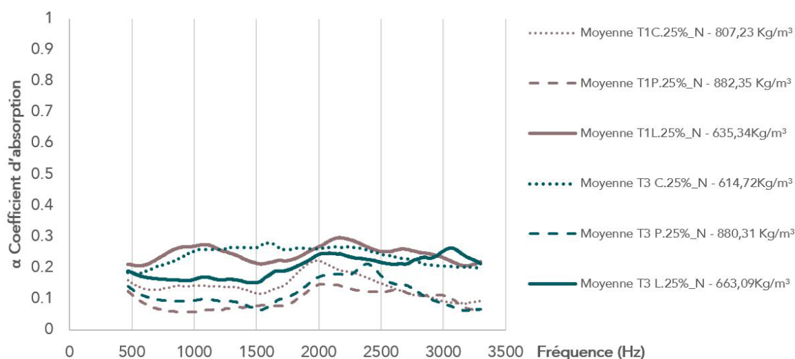
Figure 120 Valeurs d'absorption du tube de Kundt avec 25% de fibres.
