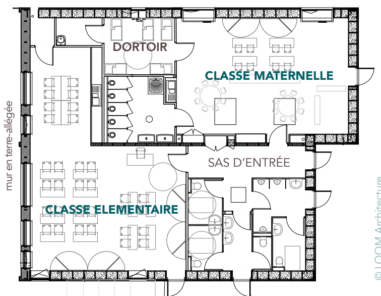
Figure 18 Plan du nouveau bâtiment de l'école de Mouais.
