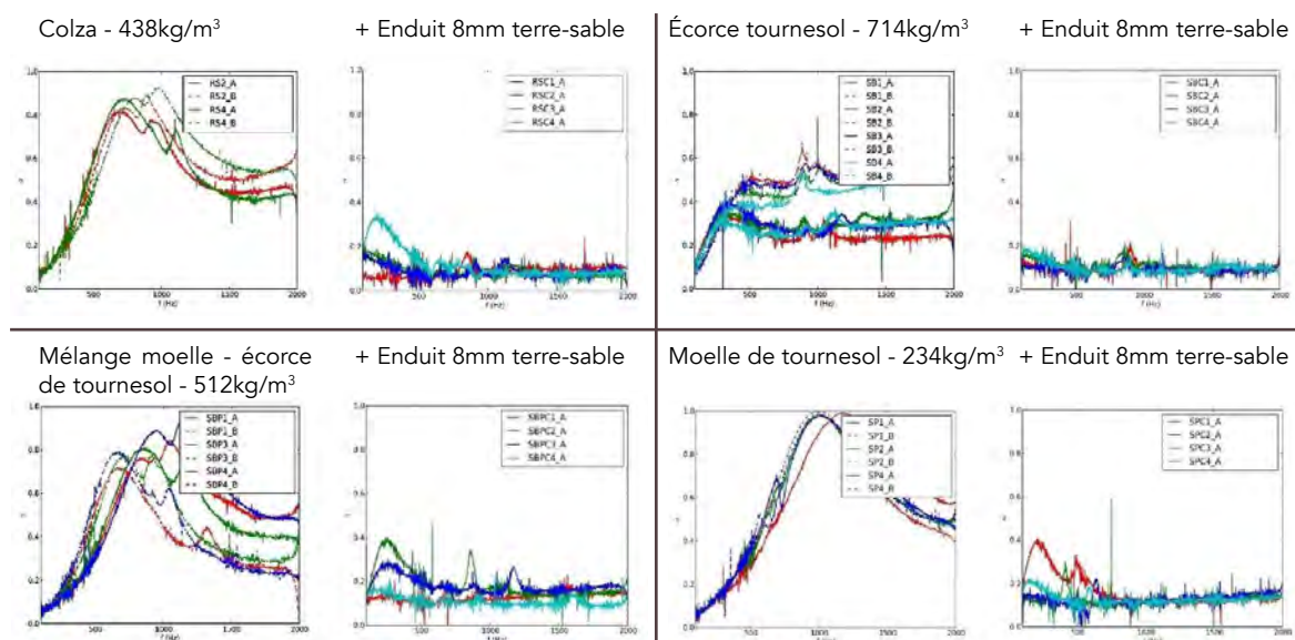
Figure 8 Coefficients d'absorption Sabine (en tube de Kundt) de quatre composites de terre allégée différentes sans et avec enduit en terre crue. Fréquences entre 0Hz et 2000Hz (Brouard, 2018).
