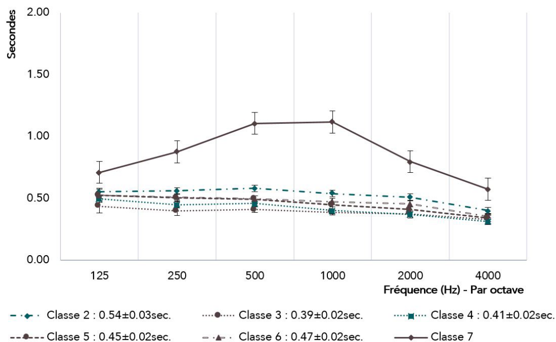
Figure 93 Moyennes des temps de réverbération (calculées à partir du T30) des différentes classes mesurées – Bouvron. Les barres d'erreur représentent l'écart type standard entre les différents points de mesure.
