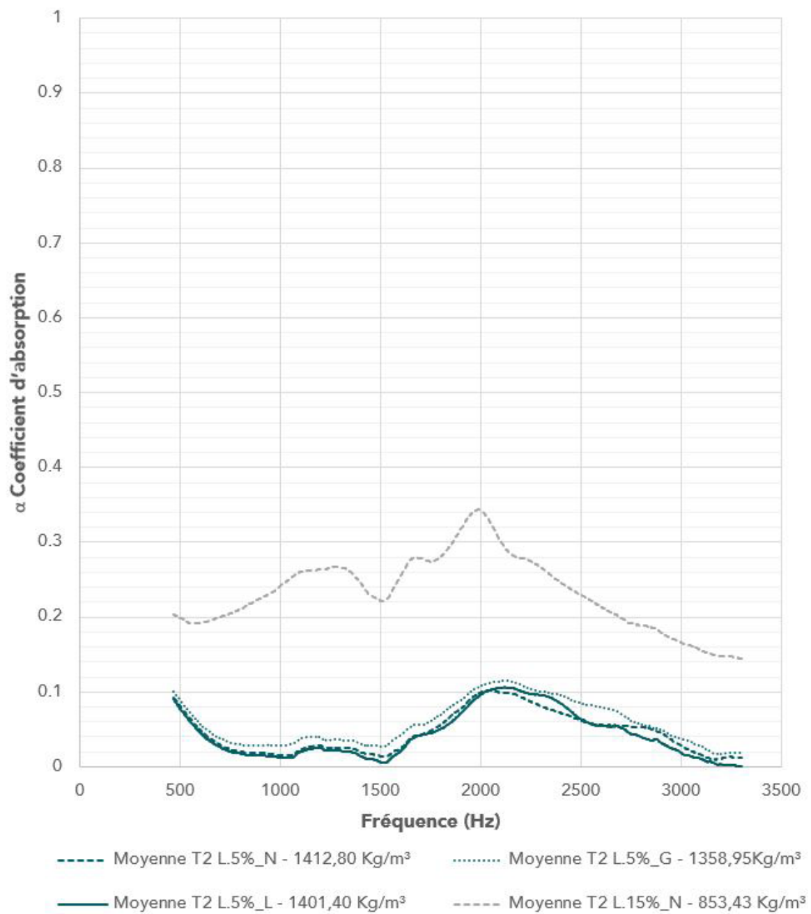
Figure 339 Coefficient d'absorption - Terre 2 - Lin
