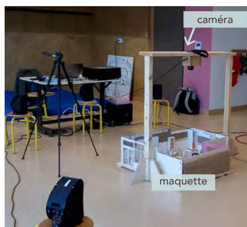
Figure 194 Installation de l'interface d'utilisateur tangible avec caméra pour identification des cibles.
