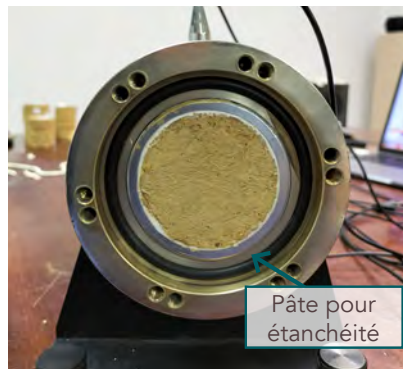
Figure 53 Incorporation de pâte dans le périmètre de l'éprouvette pour assurer l'étanchéité (exemple).
