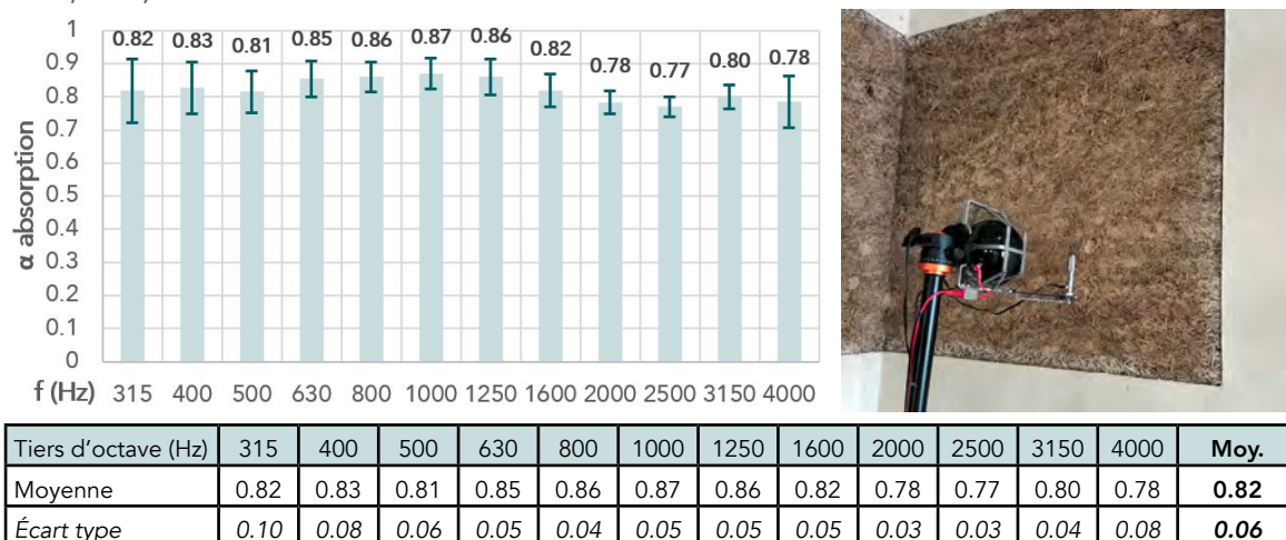
Figure 110 Mesures in situ du coefficient d'absorption acoustique (moyenne) par tiers d'octave. Mur en terre-chanvre (terre allégée).
