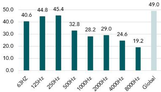
Classe 1 Meublée - Niveaux par bande et niveau global en dB(A).
