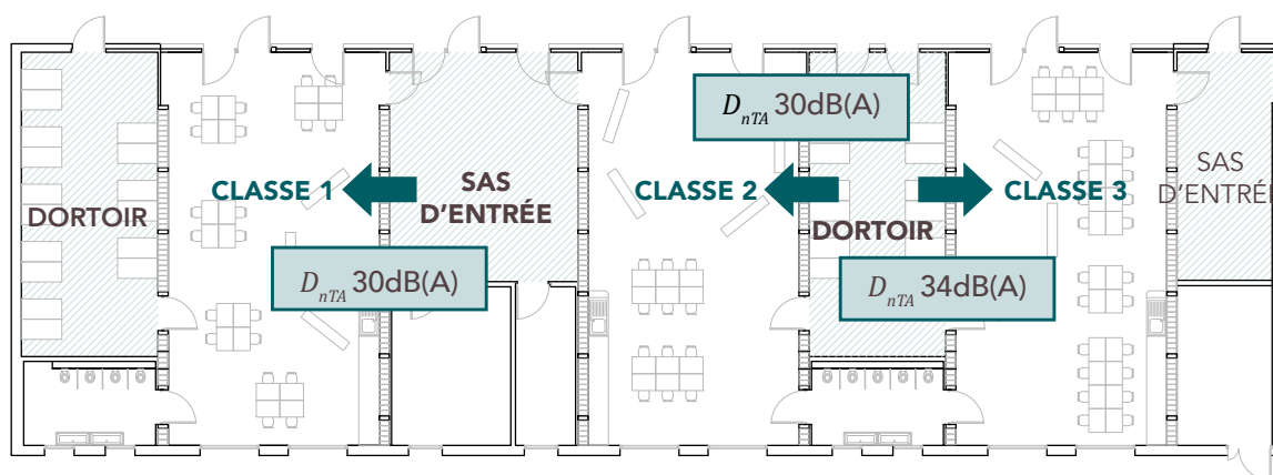
Figure 90 Isolation entre pièces à Fégréac.
