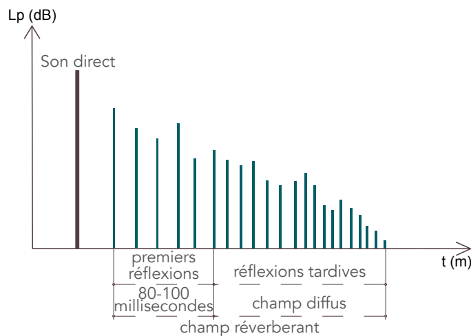
Figure 36 Champ réverbérant (Avilés López et Perera Martín, 2017).
