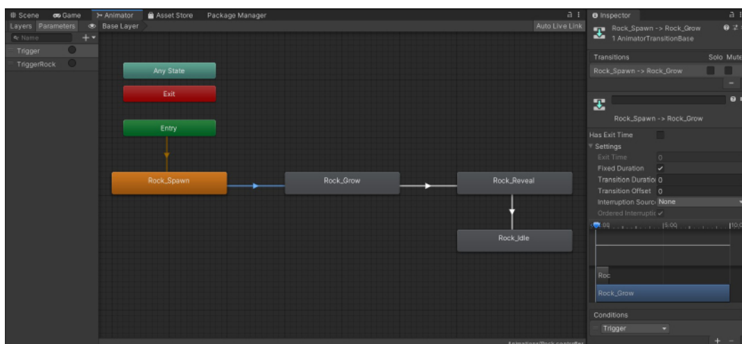
Figure 261 Fenêtre Animator.
