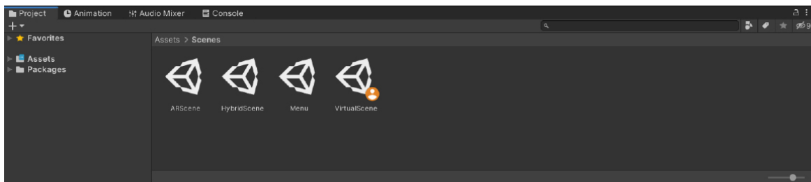
Figure 255 Dossier Scènes.
