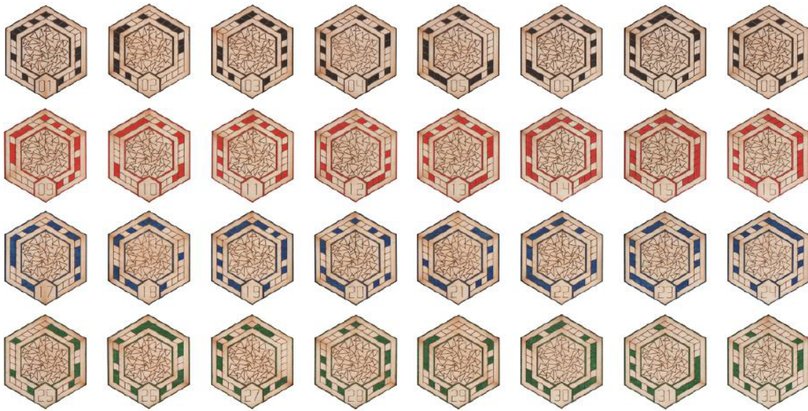
Figure 284 Cibles utilisés.
