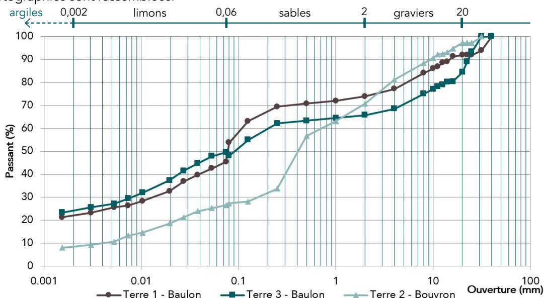
Figure 115 Graphique de la distribution granulométrique des terres étudiées.
