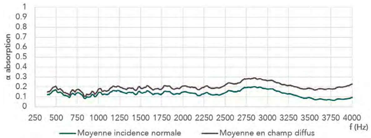
Figure 310 Comparatif entre la valeur moyenne d'absorption en incidence normale et en champs diffus. Mur en bauge (partie haute) – Bouvron.
