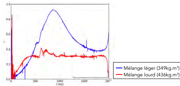
Figure 7 Coefficient d'absorption (en tube de Kundt) de deux échantillons terre-chanvre avec la même formulation mais de masses volumiques différentes (compactage différent) (Lemeurs et al., 2016).
