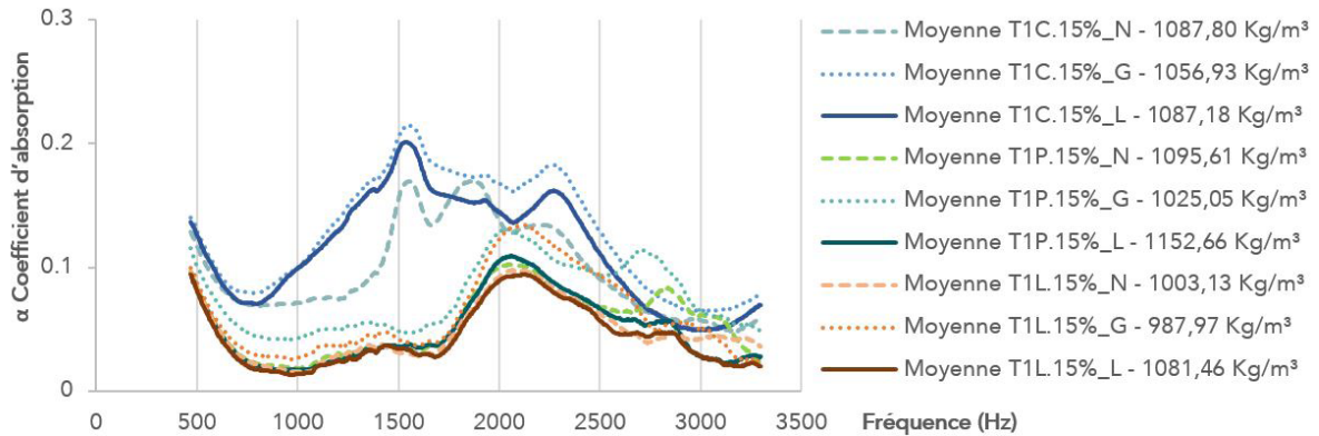
Figure 129 Valeurs d'absorption acoustique des éprouvettes avec la terre 1 et 15% de fibres.
