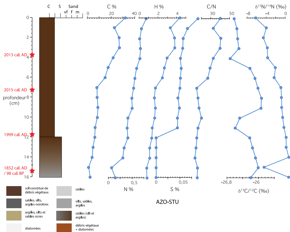
Figure 6-6 : Données de géochimie organique et isotopique, % de carbone (C), azote (N), hydrogène (H), et soufre (S), ratio C/N, \delta^{13}\text{C} et \delta^{15}\text{N} mesurées sur la carotte AZO-STU.
