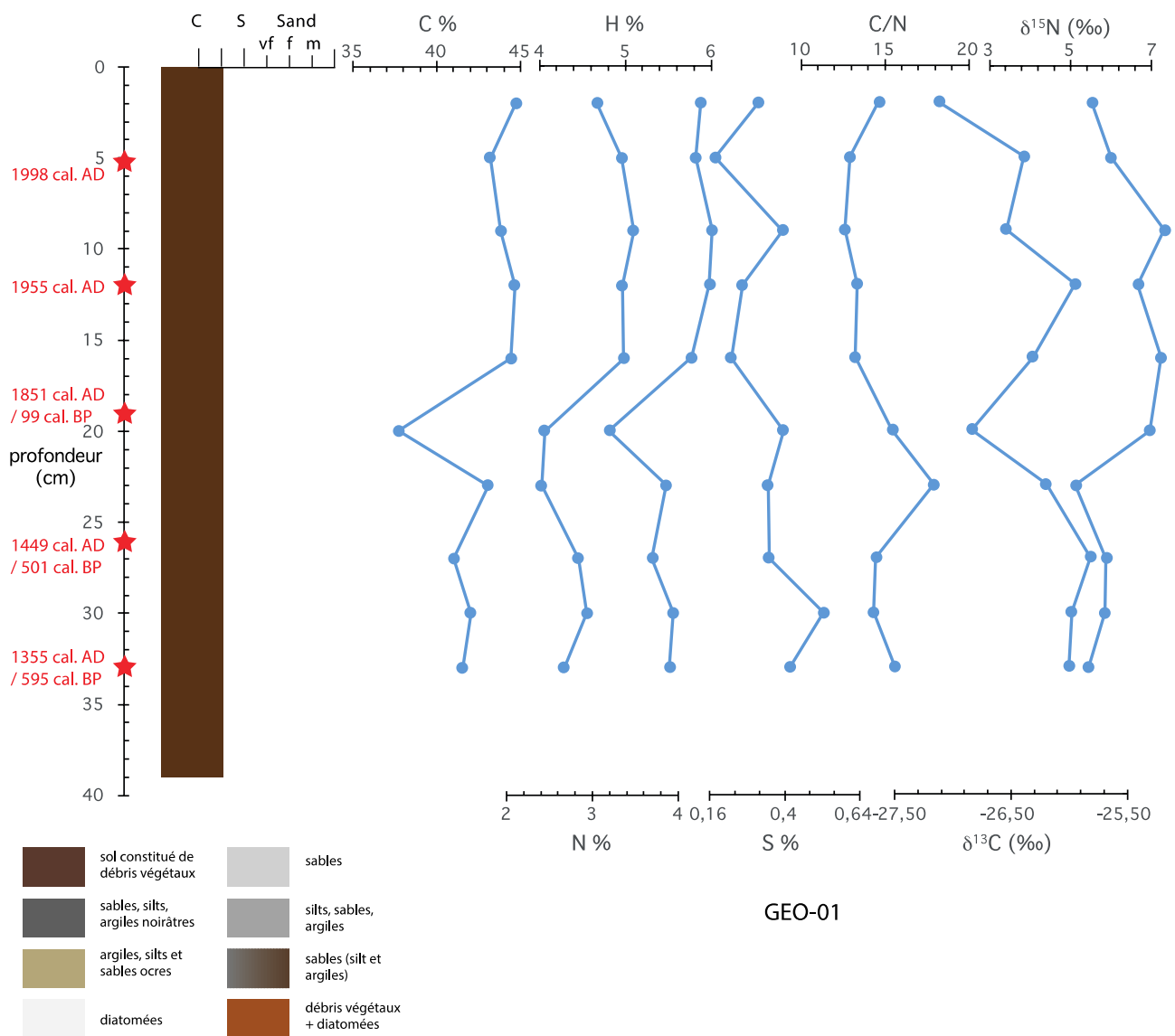
Figure 6-8 : Données de géochimie organique et isotopique, % de carbone (C), azote (N), ratio C/N, δ 13 C et δ 15 N mesurées sur la carotte GEO-01.
