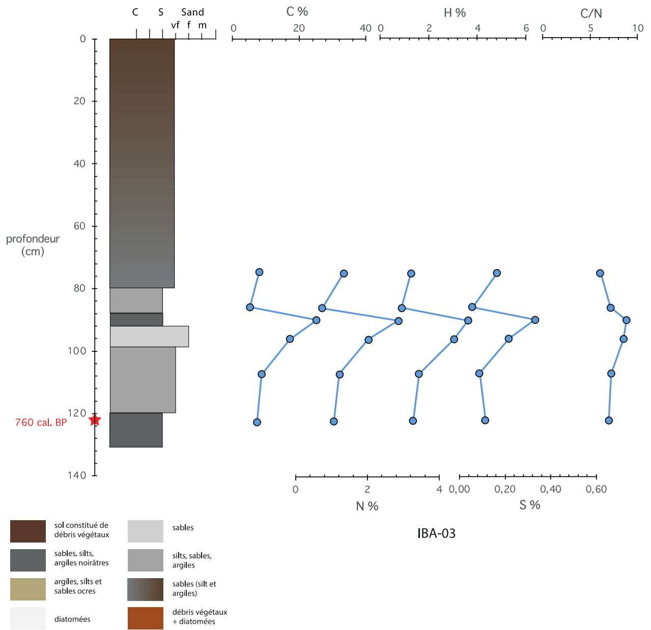
Figure 6-12 : Données de géochimie organique et isotopique, % de carbone (C), azote (N), ratio C/N, \delta^{13}\text{C} et \delta^{15}\text{N} mesurées sur la carotte IBA-03.
