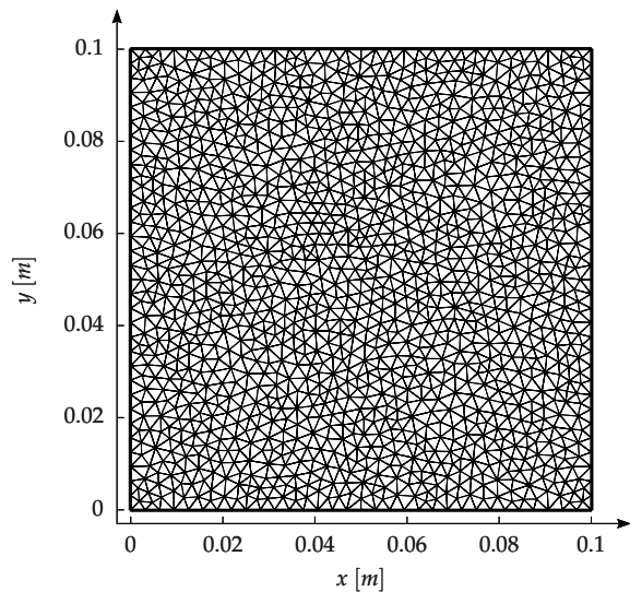
(d) UUU/TF mesh.
