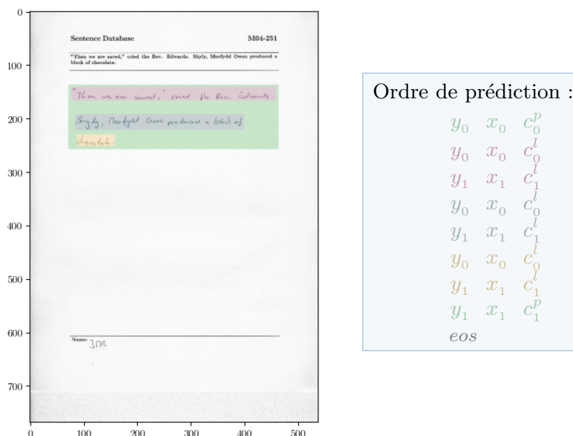
Figure 7.2 – Exemple de séquence à deux classes : paragraphe et ligne de texte. L’ordre de prédiction préserve la hiérarchie des objets : point supérieur gauche du paragraphe, point supérieur gauche de la première ligne de texte, point inférieur droit de la première ligne de texte, ..., point inférieur droit du paragraphe, fin de séquence ( eos ).
