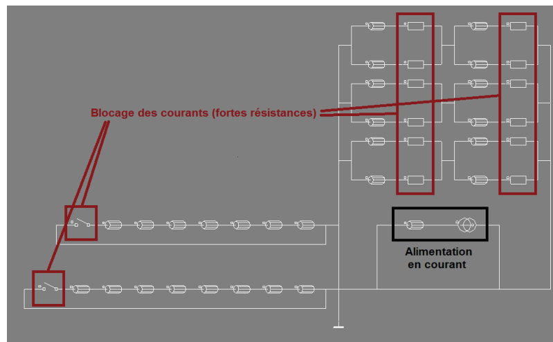
Figure 2. 21. Schéma électrique modifié pour l'identification des inductances de l'alternateur principal sous Flux2D.
