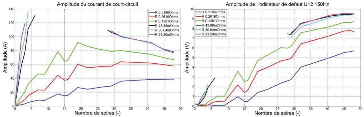
Figure 3. 48. Évolutions expérimentales des amplitudes de la composante à 150Hz de la tension composée U12 et du courant de court-circuit en fonction du nombre de spires impliquées dans le défaut et des valeurs des résistances insérées dans la boucle de court-circuit (alternateur à vide, niveau d'excitation de 0.8A).
