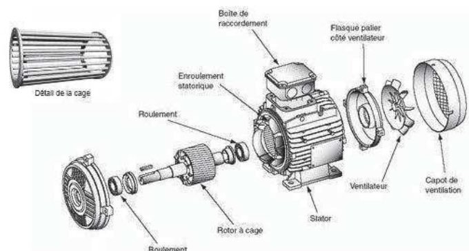
Figure 1. 5. Vue éclatée d'une machine asynchrone à cage [5].
