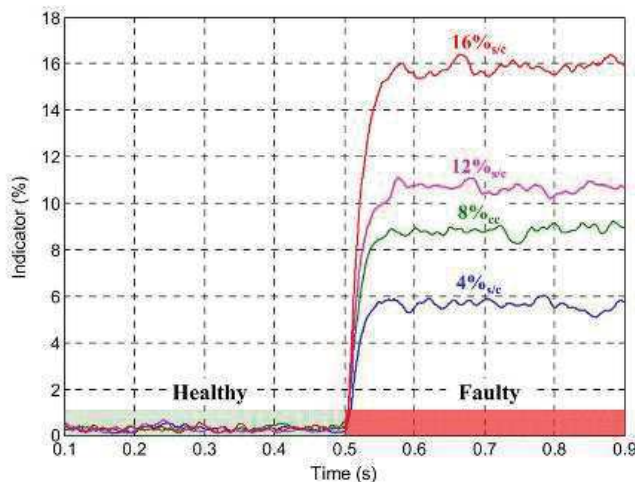
Figure 1. 30. Évolution d'un indicateur paramétrique lors de l'apparition d'un défaut de type court-circuit inter-spires avec modèle défaillant [33].
