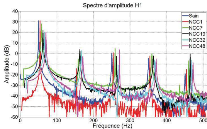
Figure 3. 44. Spectre d'amplitude expérimental de la force électromotrice H1 en fonction du nombre de spires court-circuit (alternateur à vide, excitation 0.4A, t_{FFT} = 1s , f_{ech} = 100kHz ).
