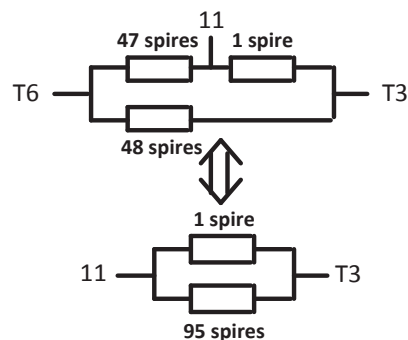
Figure 3. 13. Schéma électrique équivalent pour la mesure de la résistance d'une spire de la bobine 2-1 de la phase 3.
