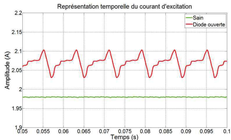
Figure 3. 49. Simulation de l'impact de la mise en circuit ouvert d'une diode du pont redresseur tournant sur le courant d'excitation pour un fonctionnement au point de fonctionnement nominal (27kVA, 400V en sortie et \cos\phi 0.8).
