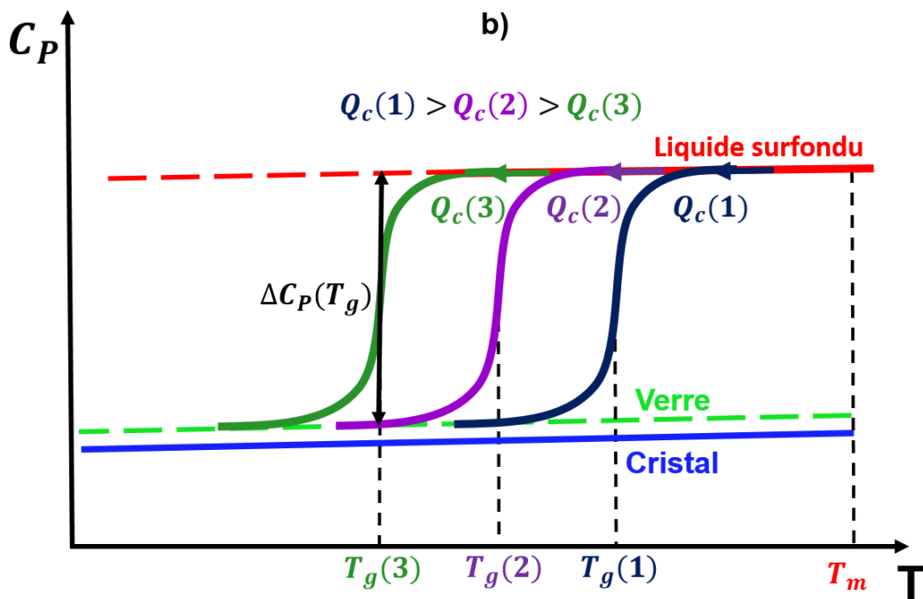
Figure 7 : Évolution schématique en fonction de la température et pour différentes vitesses de refroidissement Q_c(1) , Q_c(2) , Q_c(3) :
