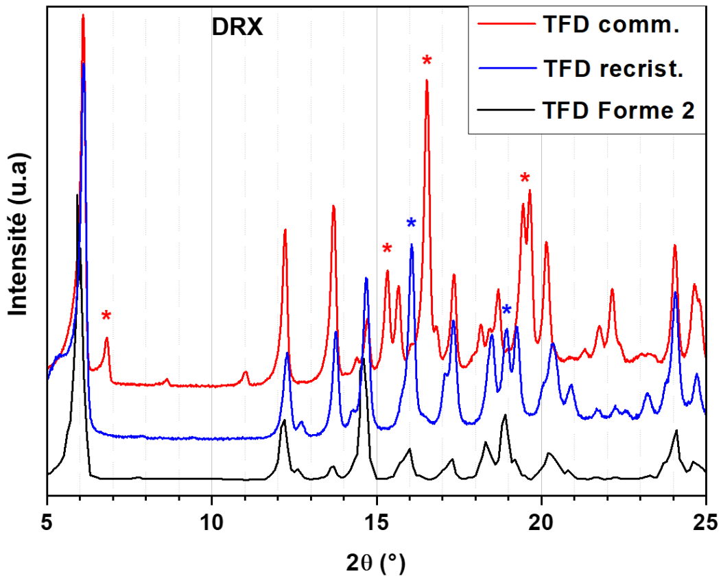
Figure 7: Diffractogrammes de rayons X enregistrés à température ambiante l'échantillon obtenu par reprécipitation dans le méthanol après recristallisation à 100°C (en bleu). Pour comparaison, le diffractogramme de la forme 2 reporté dans [15] est également représenté (en noir). Les * indiquent les raies caractéristiques de chaque forme.
