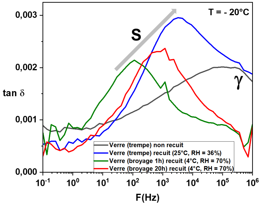
Figure 45 : Enregistrements à -20^\circ\text{C} de \tan \delta = \varepsilon'' / \varepsilon' en fonction de la fréquence F , montrant les relaxations S et \gamma dans le cas du verre de Terfenadine obtenu par fusion/trempe, non recuit (courbe noire) et recuit 17 jours à température ambiante ( \text{RH} = 36\% ) (courbe rouge), et du verre obtenu par broyage d'1h (courbe bleue) ou 20h (courbe verte) et conservé environ un an au réfrigérateur ( T = 4^\circ\text{C} , \text{RH} = 70\% ).
