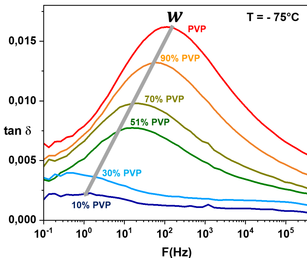
Figure 18 : Evolution fréquentielle de \tan \delta pour les mélanges Terfénaire/PVP de compositions variables obtenus par co-broyage de 10h à température ambiante.
