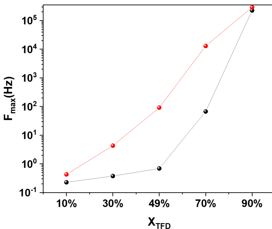
Figure 34 : Comparaison à 110°C de la position du maximum du mode \alpha (ou \alpha_2 ) des différents mélanges Terfénadine/PVP obtenus par co-broyage (en rouge) ou par trempage depuis l'état liquide (en noir).
