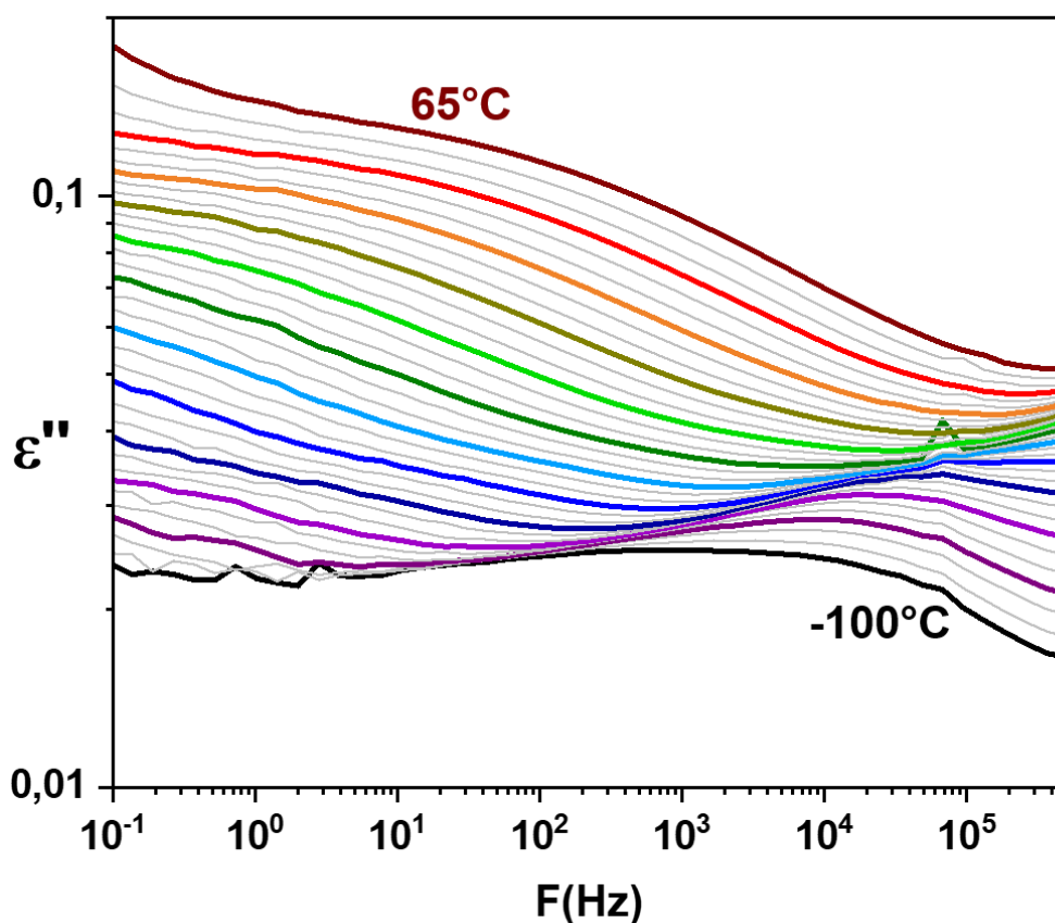
Figure 19 : Enregistrements de \epsilon'' lors d'isothermes comprises entre -100°C et 65°C (par pas de 5°C) réalisés dans le cas d'une DSA contenant 49% w/w de Terfénadine obtenue par trempe depuis l'état liquide.
