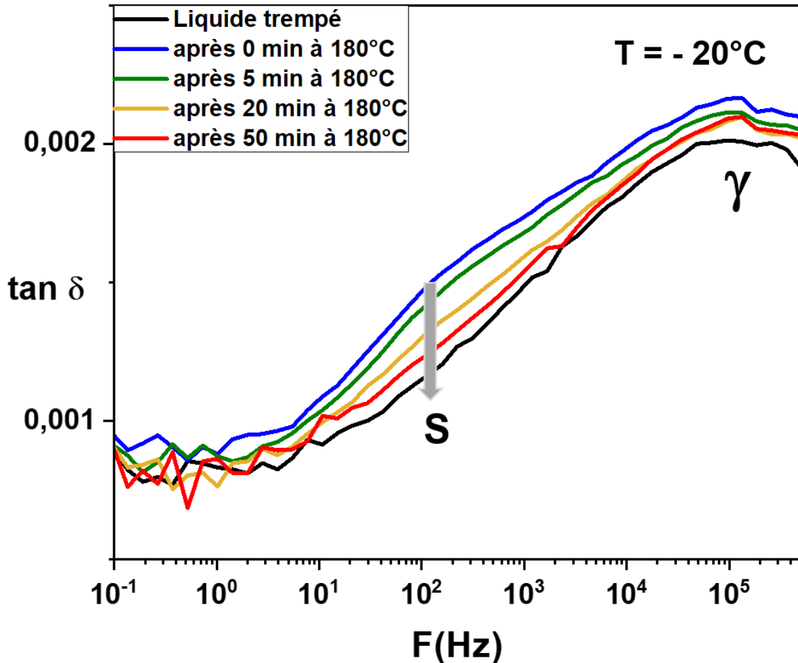
Figure 43 : Enregistrements à -20^\circ\text{C} de \tan \delta = \varepsilon'' / \varepsilon' en fonction de la fréquence, montrant la relaxation \gamma dans le cas du verre de Terféndine obtenu par trempe du liquide et non recuit à température ambiante (courbe noire) et après un recuit de différents temps (0,5,20,50 min) à 180^\circ\text{C} , du verre de Terféndine préalablement stocké 21 jours dans un dessiccateur contenant une solution saturée de chlorure de sodium (76% d'humidité relative à température ambiante).
