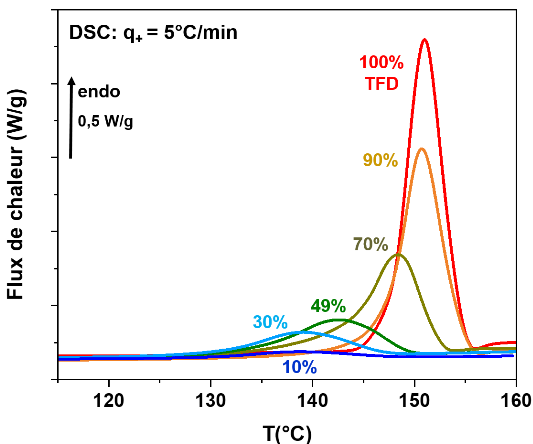
Figure 1 : Thermogrammes DSC enregistrés au chauffage à 5°C/min des différents mélanges physiques Terfénadine/PVP de compositions variables (10%, 30%, 49%, 70%, et 90% w/w de Terfénadine).
