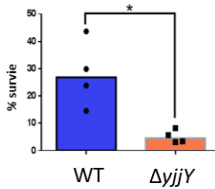
Figure 44 : Etude de l'impact de la délétion du gène yjjY la survie en présence de loméfloxacine
