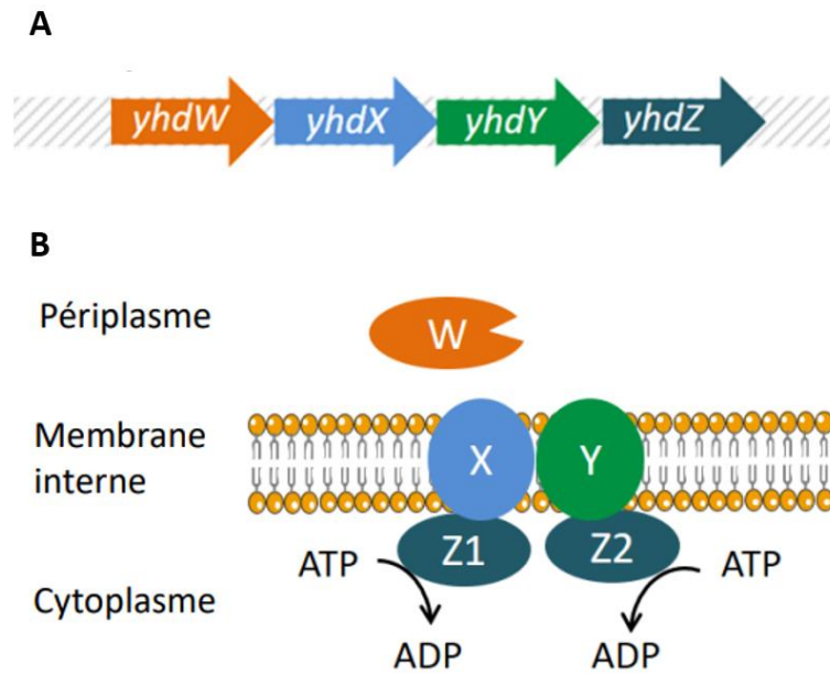
Figure 45 : Schématisation de l'organisation de l'opéron yhd et du transporteur Yhd
