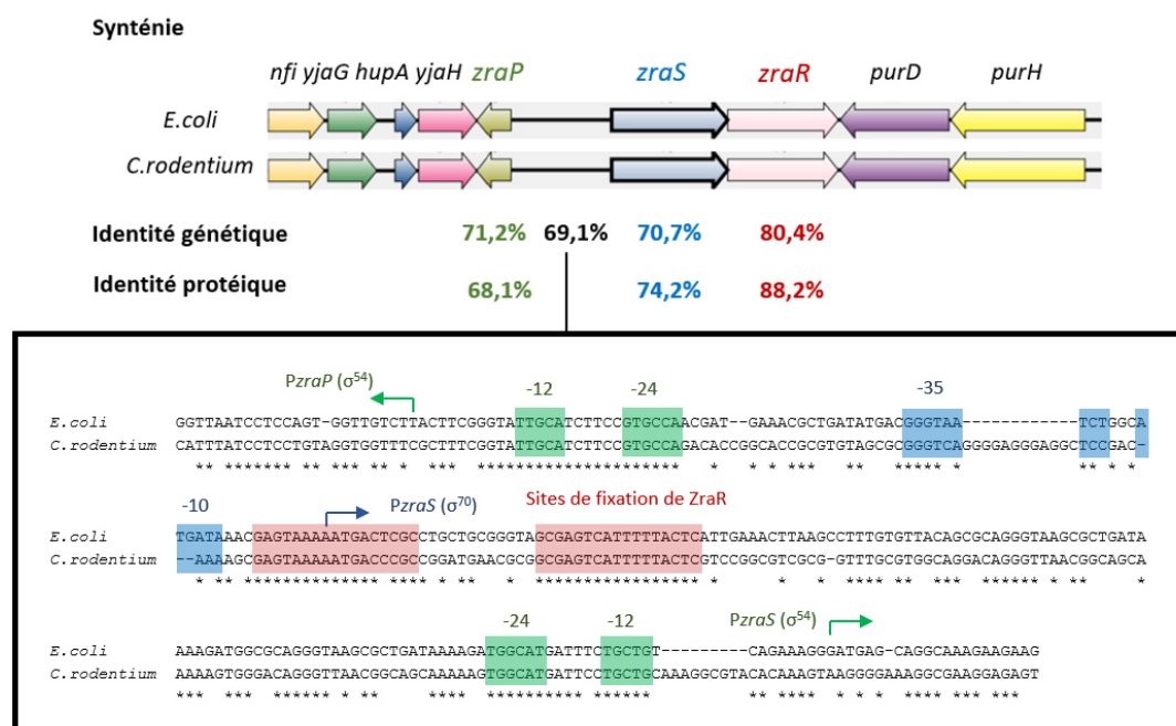
Figure 30 : Comparaison du système ZraPSR chez E. coli et C. rodentium au niveau génétique et protéique
