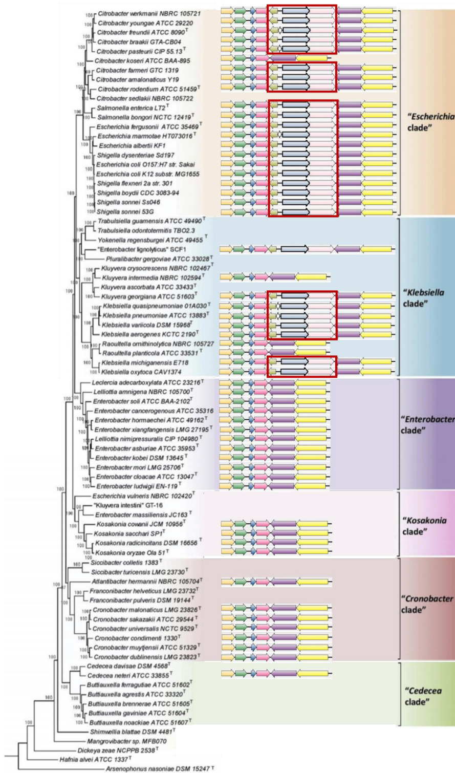
Figure 29 : Présence des éléments du système Zra dans la famille des Enterobacteriaceae
