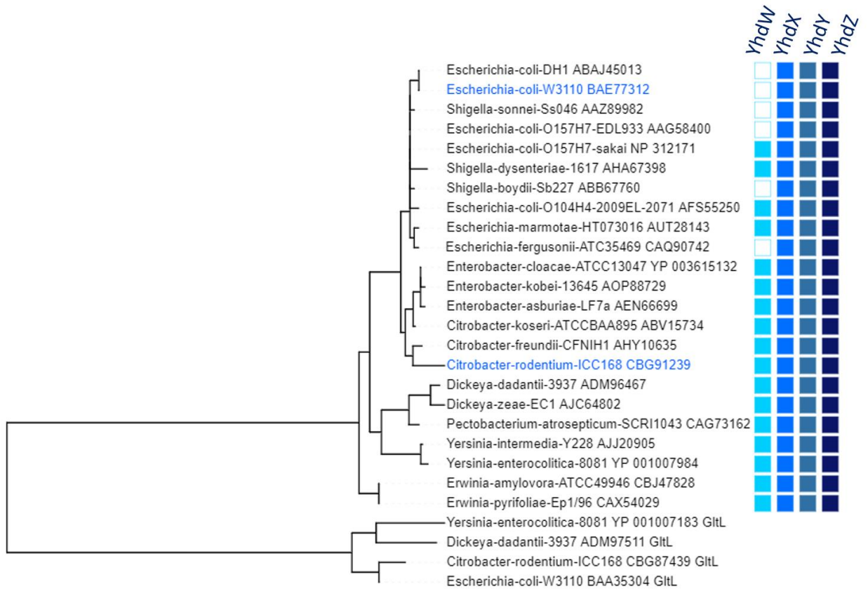
Figure 46 : Arbre phylogénétique de l'ATPase, YhdZ, et présence des autres éléments du transporteur chez les entérobactéries
