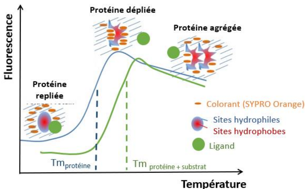
Figure 23 : Principe du Fluorescence-based thermal shift assay
