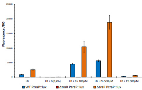
Fig 3 profil d'induction de zraP dans des mutants ΔzraP or ΔzraR et en présence de cations divalents (des résultats identiques sont obtenus avec la fusion zraS::lux )
