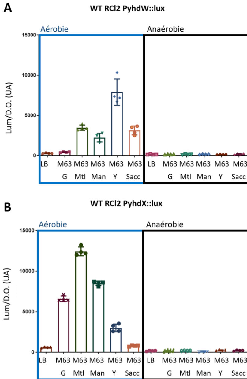
Figure 62 : Profil d'activité des promoteurs de yhdW et yhdX chez la souche sauvage en aérobiose et en anaérobiose
