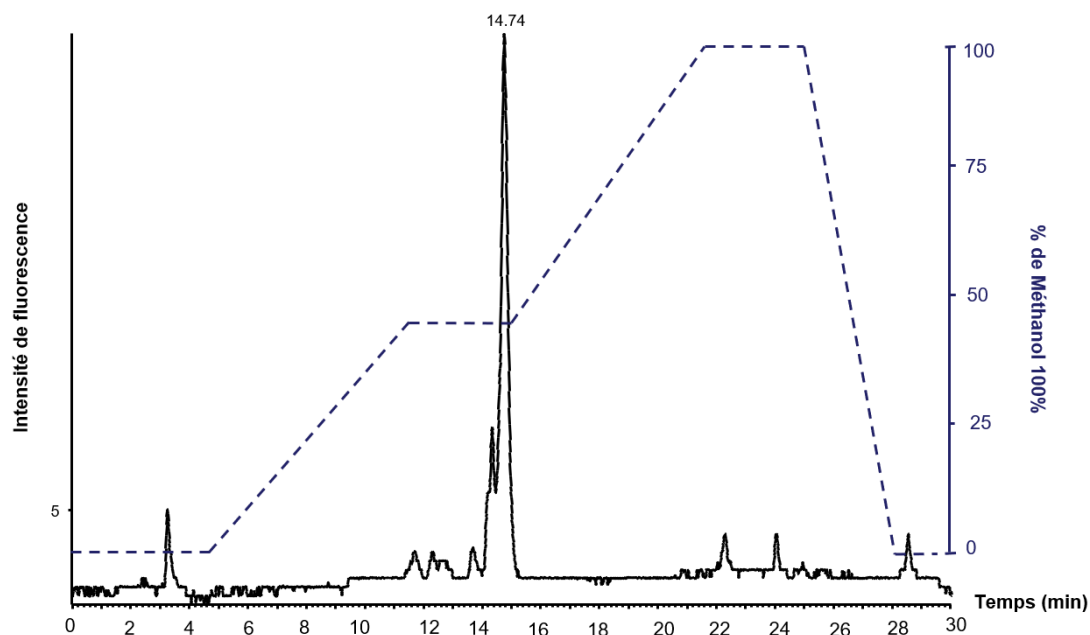
Figure 26 : Chromatogramme pour la détection par fluorescence en HPLC de 5ng de loméfloxacin
