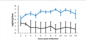
Fig. 6: Suivi du nombre de bactéries au cours de temps post-infection sur milieu Mc Conkey sorbitol
