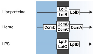
Figure 18 : Les transporteurs ABC chez E. coli K12
