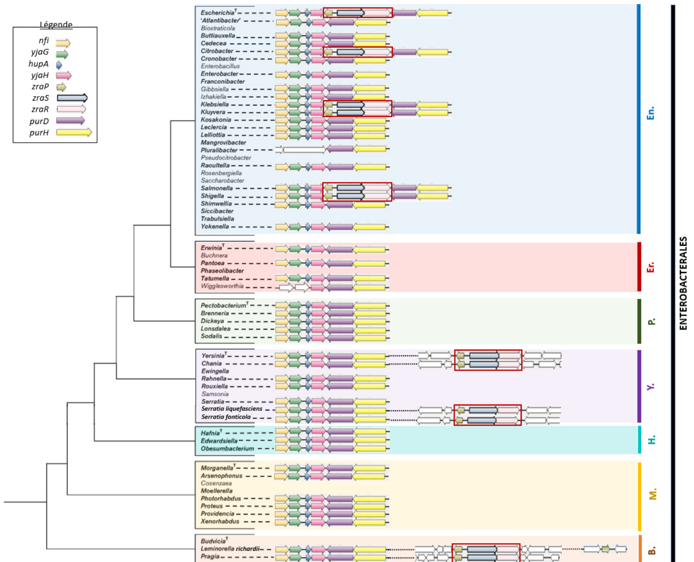
Figure 28 : Présence des éléments du système Zra dans l'ordre des Enterobacterales
