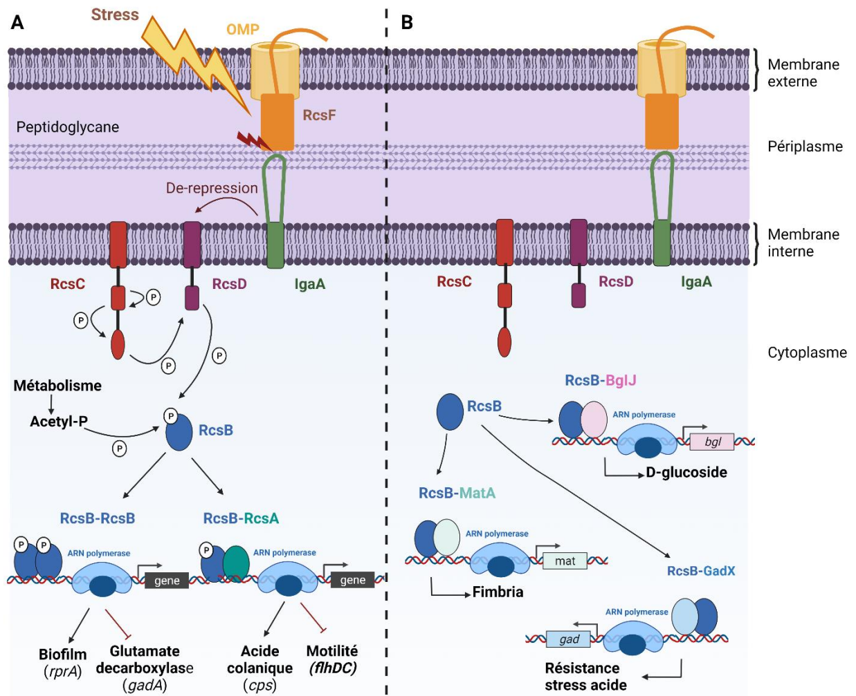
Figure 7 : Représentation schématique du fonctionnement du système Rcs
