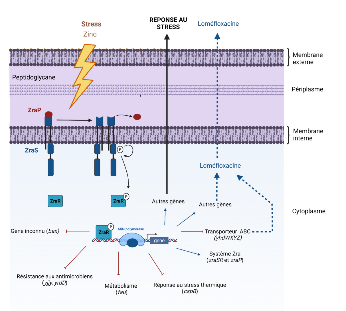
Figure 67 : Schématisation du fonctionnement du système ZraPSR
