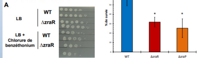
Fig 2 : A-CMI en présence de chlorure de benzéthonium. B-Relative survival rate of the ΔzraP or ΔzraR mutants, compared to the wild type strain. * p ≤ 0,05, Student's t test
