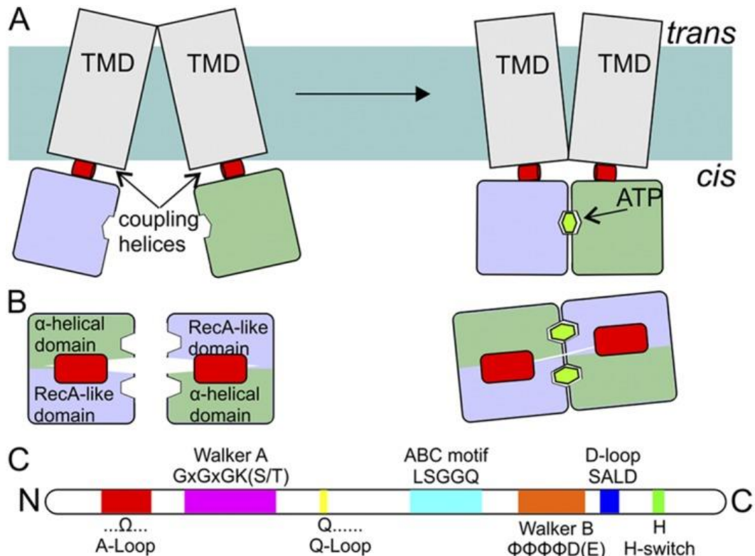
Figure 15 : Représentation schématique des NBDs et des différents motifs conservés
