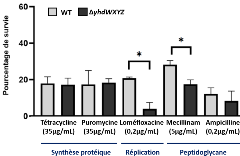
Figure 53 : Pourcentages de survie de E.coli WT et \Delta yhdWXYZ en présence de différents antibiotiques
