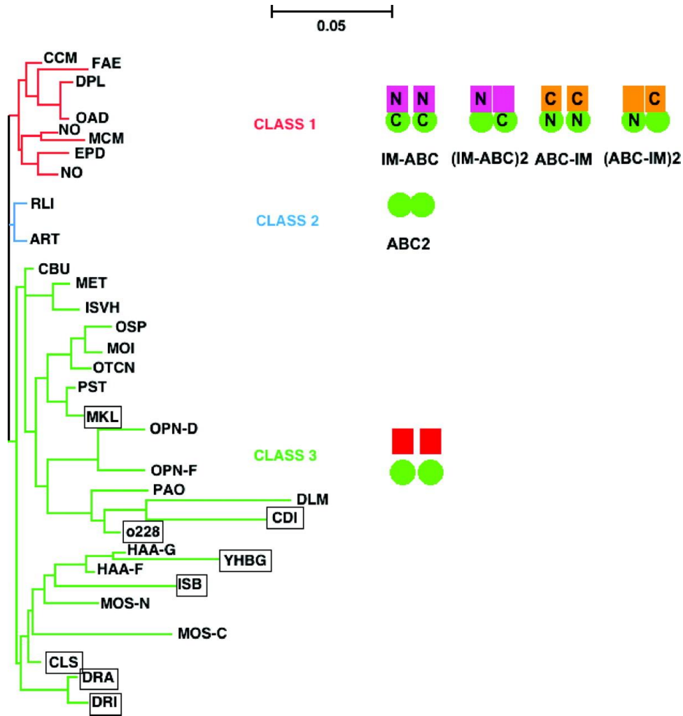
Figure 14 : Arbre phylogénétique simplifié des transporteurs ABC du vivant
