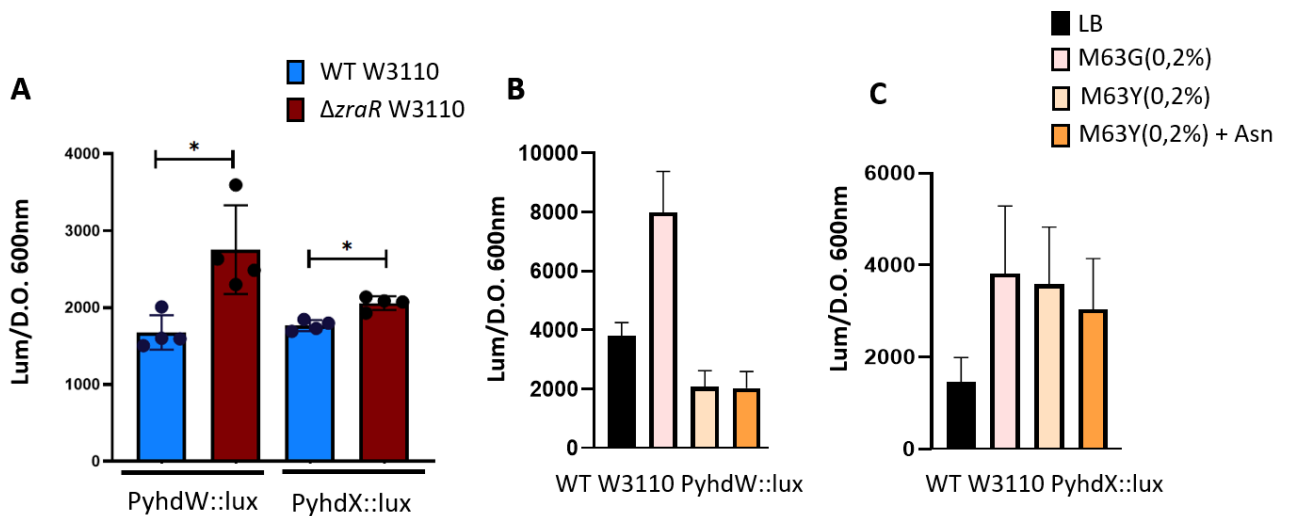
Figure 49 : Profil d'induction de la fusion yhdW::lux et yhdX::lux de E. coli
