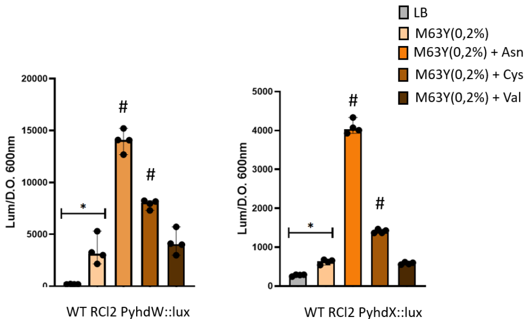
Figure 61 : Profil d’activité des promoteurs de yhdW et yhdX chez la souche sauvage
