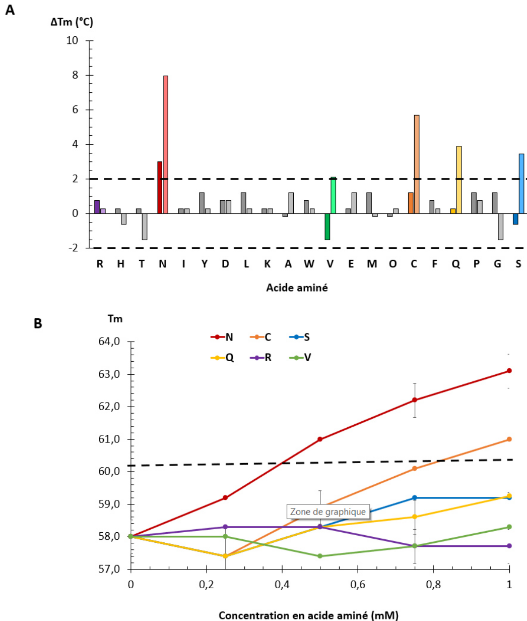
Figure 57 : Etude de l'interaction de YhdW avec les acides aminés par fluorescent thermal shift assay
