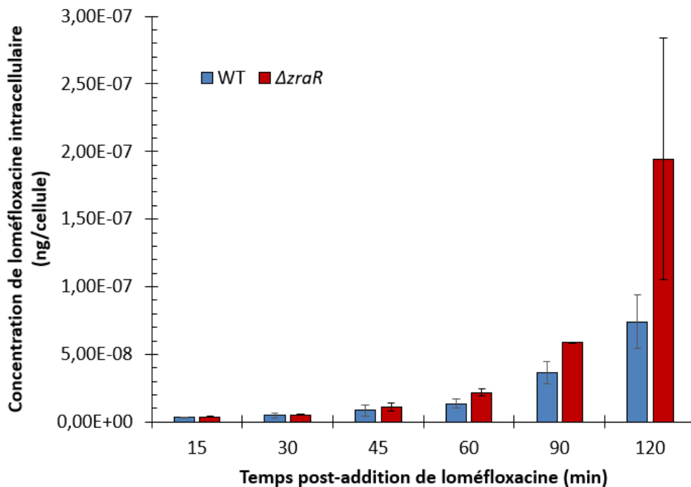
Figure 40 : Quantification de l’accumulation de la loméfloxacin à l’intérieur de la cellule
