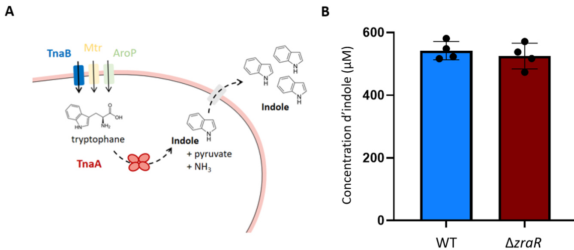
Figure 38 : Effet de la mutation de zraR sur la production d'indole
