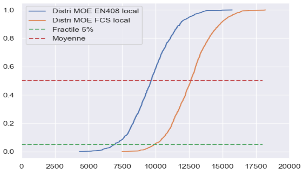
Figure n° 100 : Distributions des MOE' apparents de 1020 poutres BLC générées sur la base des lois expérimentales EN408 local et FCS local
