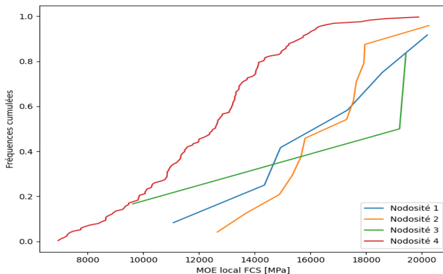
Figure n° 69 : Fréquences cumulées des MOE local en fonction de la nodosité : configuration sur chant (FCS)
