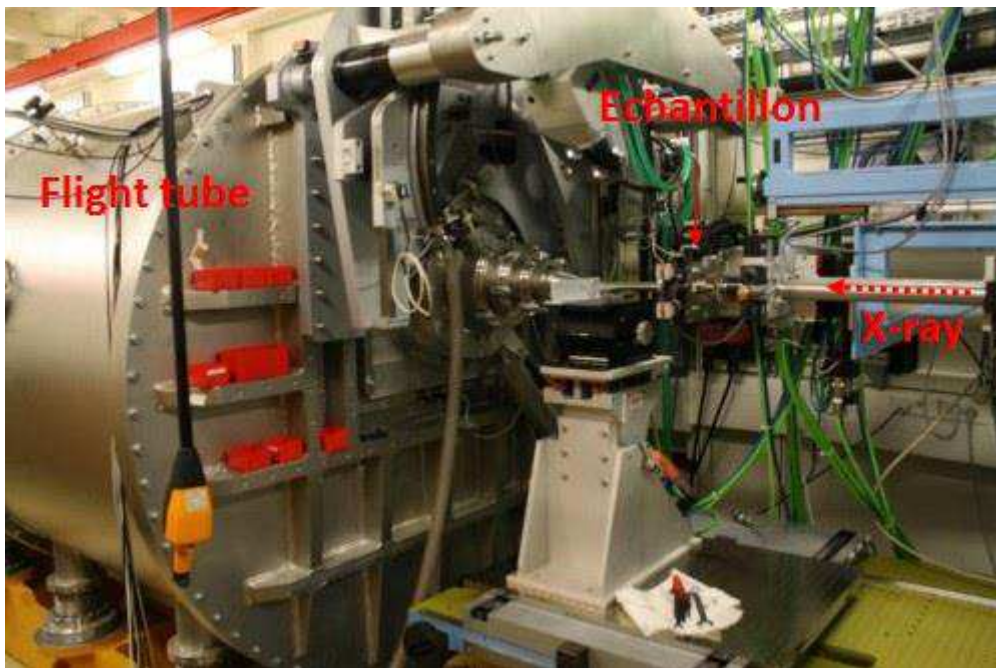
Figure IV.5. Photographie de la cabine expérimentale de la ligne SWING
