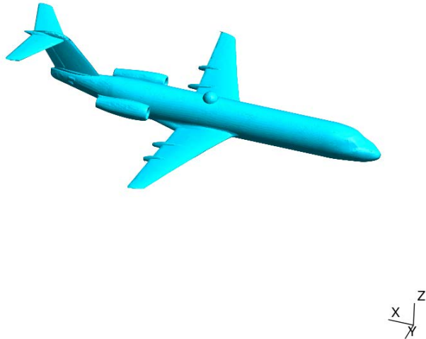
FIGURE 4.1.3 – Avion discrétisé en surface avec 77 190 DDLs.
