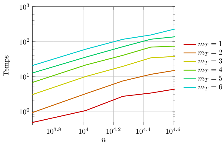
FIGURE 3.2.6 – Temps moyen de réalisation de l'étape de compression par ACA du noyau en fonction de m_T ( \epsilon_{HCA} = 10^{-4} ).
