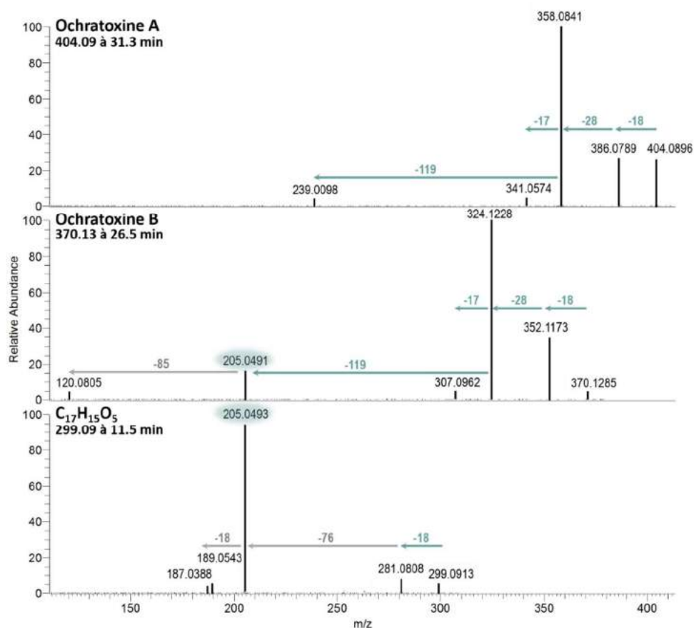
Figure 35. Comparaison des spectres MS/MS de l'ochratoxine A, de l'ochratoxine B et du métabolite C 17 H 14 O 5 détecté à 11,5 min.
