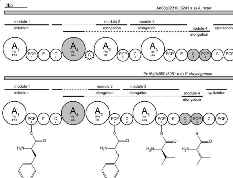
Figure 11. Schématisation des gènes hcpA d' A. niger (haut) et de P. chrysogenum (bas) responsables notamment de la synthèse de fungisporines chez ces champignons. Extrait de Ali et al. 2014 40
