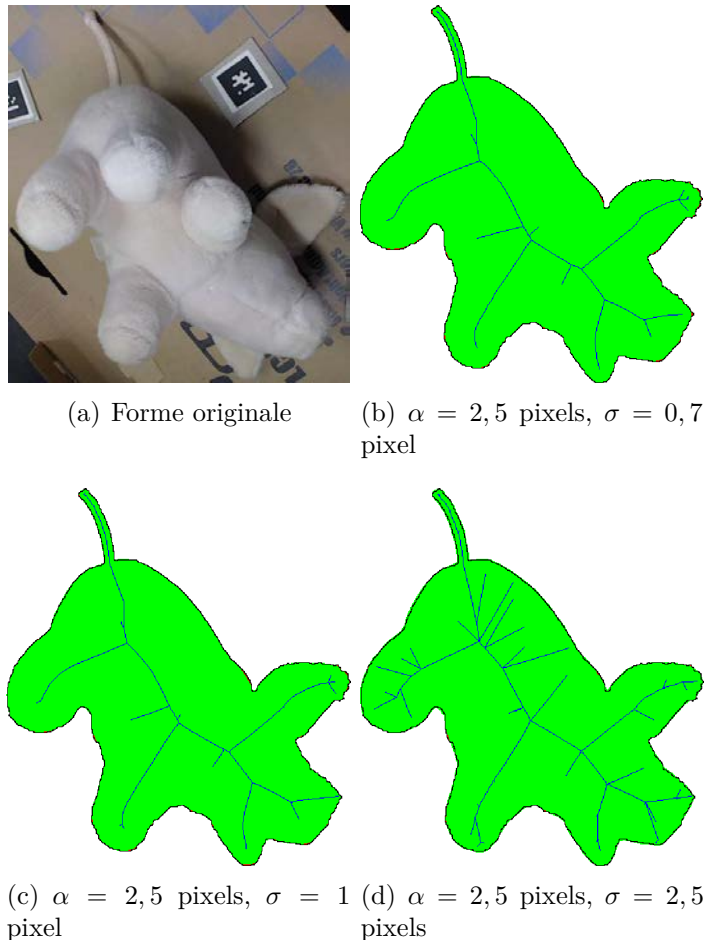
FIGURE 4.34 – Pour \alpha = 2,5 pixels, effet de valeurs extrêmes de \sigma sur le squelette estimé. Pour une valeur élevée de \sigma , on constate ici que le squelette possède un grand nombre de branches peu informatives. Quand ce paramètre prend des valeurs faibles, le nombre de branches est peu élevé.
