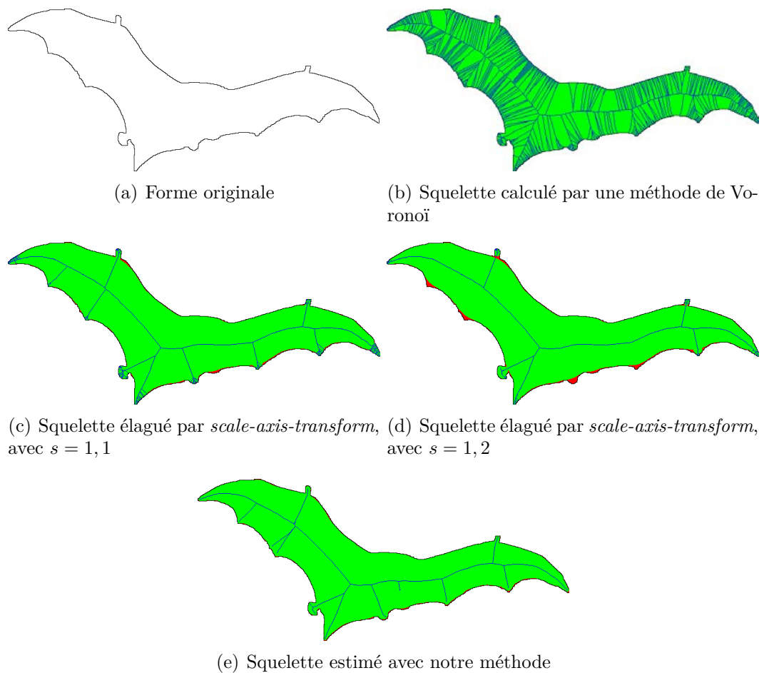
FIGURE 4.10 – Illustration des différentes techniques d'élagage. L'élagage d'un squelette ne donne pas toujours des résultats adaptés à la forme initiale ((b), image issue de la base de données MPEG-7 [65]). Le résultat d'une squelettisation par l'algorithme de Voronoï est présenté en (b). Comme ce squelette est fortement bruité, du fait de la rasterisation, un élagage permet d'éliminer une grande partie des branches. Le résultat d'un élagage par le scale-axis-transform est exposé en (c) et (d). On constate cependant que certaines parties de la forme initiale (en rouge), ne sont plus prises en compte par la forme engendrée par le nouveau squelette (en vert), tandis que du bruit subsiste (visible par exemple au bout des ailes, sous la forme de branches multiples, surtout en (c)). La méthode de squelettisation que nous proposons, en (e), restitue la forme squelettisée en minimisant le bruit sur le squelette.
