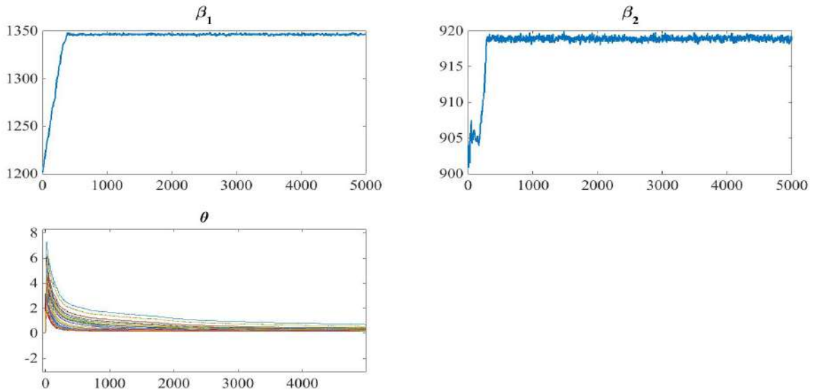
Figure F.5: Evolution de la convergence des chaînes de Markov pour les différents paramètres \hat{\beta}_1, \hat{\beta}_2, \hat{\theta} estimés pour des images MCR réelles.
