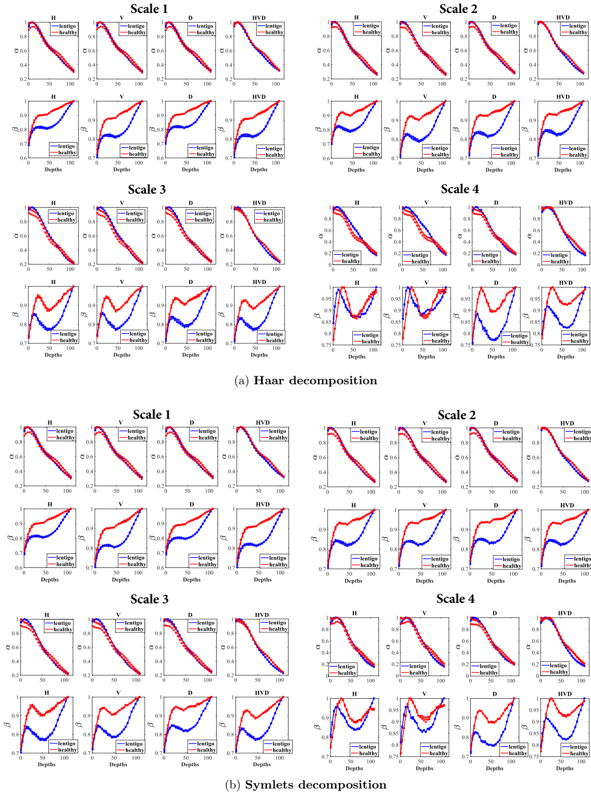
Figure 2.11: Évolution des paramètres moyens \hat{\alpha} et \hat{\beta} en fonction de la profondeur, pour les différentes bandes à toutes les échelles. Les valeurs de \alpha sont très similaires pour les patients sains et lentigo et ne peuvent être utilisées pour la discrimination. Le paramètre \beta montre une différence significative pour les profondeurs entre 31 \mu m et 76 \mu m , avec une différence maximale aux environs de 50 \mu m . Notre conclusion est que ce paramètre \beta peut discriminer les tissus sains et lentigo de la peau.
