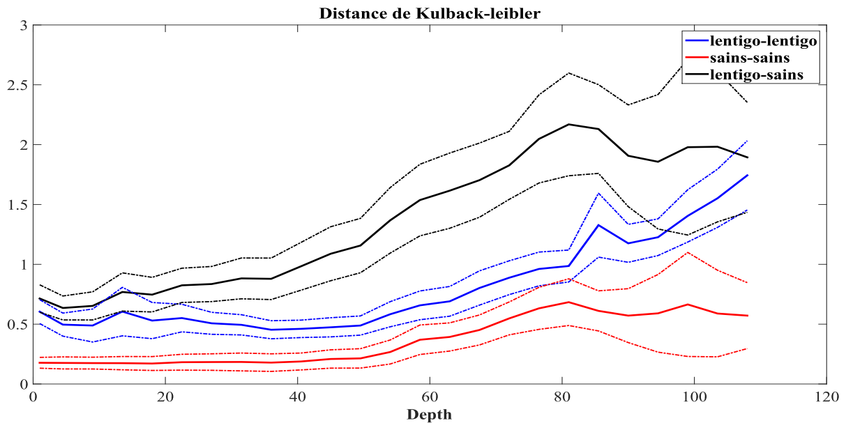
Figure 3.13: Évolution des distances Kulback-Leibler moyennes tout au long de la profondeur. Les distances montrent une différence significative pour les profondeurs entre 30 \mu m et 76 \mu m , avec une différence maximale aux environs de 50 \mu m .
