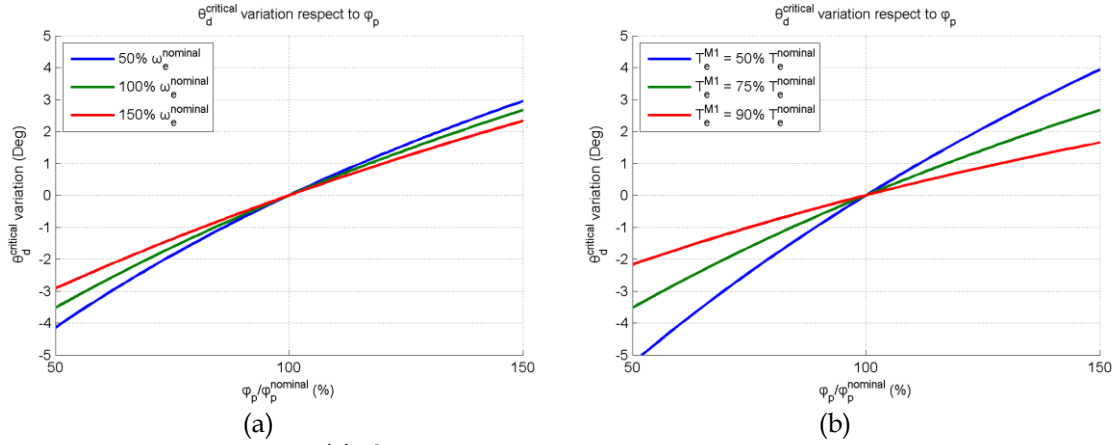
Figure 1.17 \theta_d^{critical} en fonction de (a) \varphi_p et \omega . (b) \varphi_p et le Couple.
