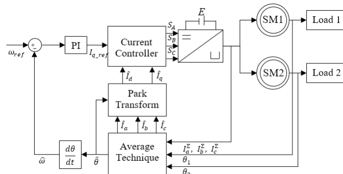
Figure 1.6 Schéma du contrôleur de la stratégie basée sur les valeurs de algébrique moyennes
