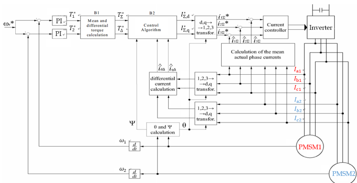
Figure 1.7 Schéma du contrôleur de \Sigma - \Delta
