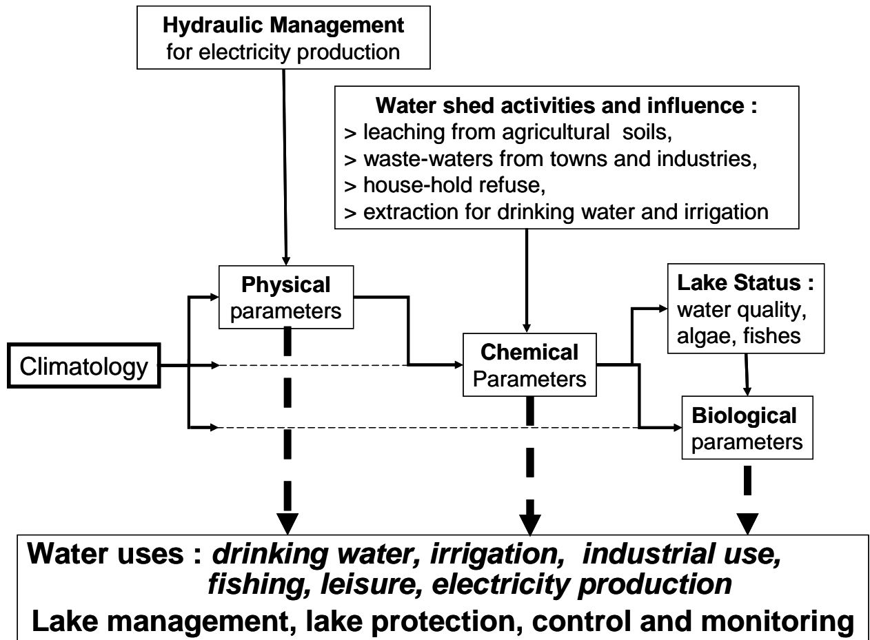
Figure 2. Les principaux facteurs influençant le volume d'eau dans le lac Taabo. (Groga et al ; sous presse)
