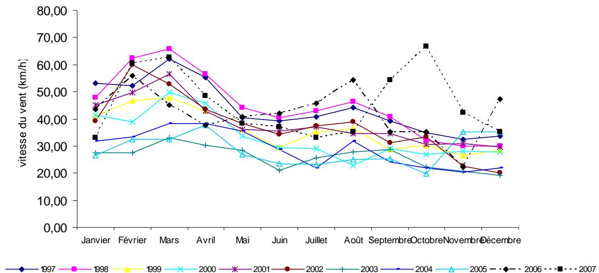
Figure 18. Variation pluri-annuelle moyenne du vent dans la région de Taabo entre 1997 et 2007.
