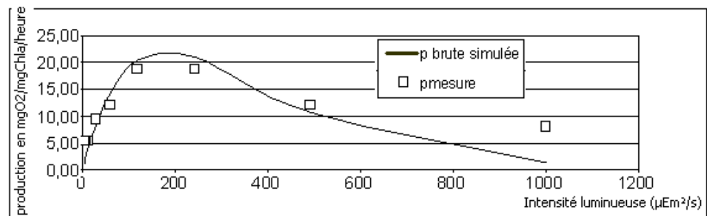
Figure 31. Exemple de calcul à partir des mesures de terrain : le modèle de Steele (1962) est calé (Pmax, Iopt) sur les valeurs expérimentales.
