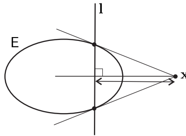
FIGURE 6.3: La relation pôle-polaire : la droite l = E\mathbf{x} est la polaire du point \mathbf{x} respectivement à la conique E [Hartley 2004b, p. 58].
