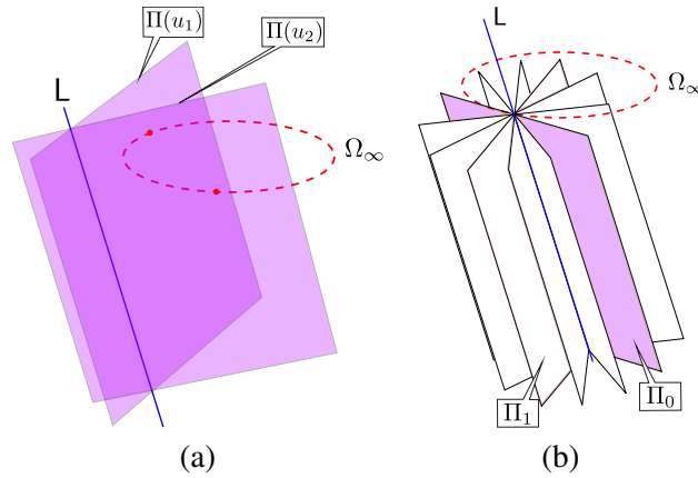
FIGURE 4.3: Preuve de la proposition 29. (a) Par une droite L, il passe deux plans \Pi(u_1) et \Pi(u_2) (combinaisons linéaires de \Pi_0 et \Pi_1 ), qui sont tangents à la conique absolue \Omega_\infty . (b) Lorsque L intersecte \Omega_\infty , u_1 = u_2 et \Pi(u_1) et \Pi(u_2) sont confondus.
