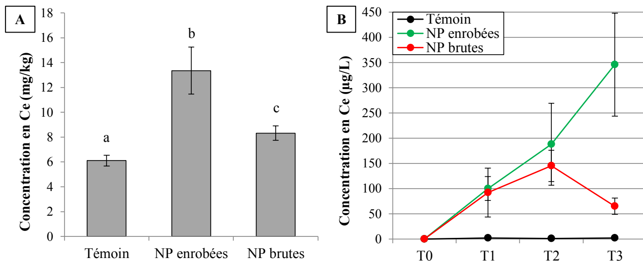
Figure 4 : Accumulation des NP de CeO 2 dans les compartiments abiotiques. (A) dans le sédiment. Les concentrations (valeurs moyennes ± erreur standard) sont mesurées en fin d'expérience. Les lettres (a,b,c) indiquent des groupes statistiques différents. (B) dans la colonne d'eau. Les concentrations (valeurs moyennes ± erreur standard) sont mesurées plusieurs fois durant l'expérience. T0 : première introduction de NP. T1 : introduction des chironomes. T2 : introduction des pleurodèles. T3 : fin de l'expérience.
