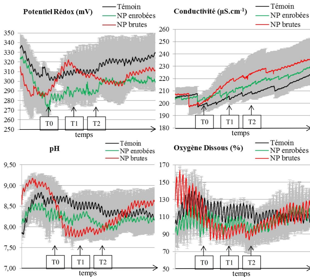
Figure 3 : Courbes de variation de potentiel rédox, conductivité, pH et oxygène dissous (valeurs moyennes) en fonction du temps. Les zones grisées représentent les valeurs d'écart-type. T0 : première addition de NP ; T1 : introduction des larves de chironome ; T2 : introduction des larves de pleurodèle.
