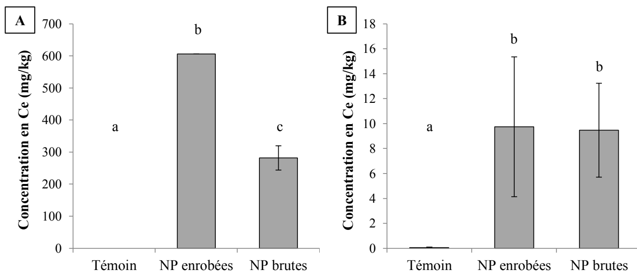
Figure 5 : Accumulation des NP de CeO 2 dans les organismes. (A) chez C. riparius et (B) chez P. waltl. . Les concentrations (valeurs moyennes ± erreur standard) sont mesurées en fin d'expérience. Les lettres (a,b,c) indiquent des groupes statistiques différents.
