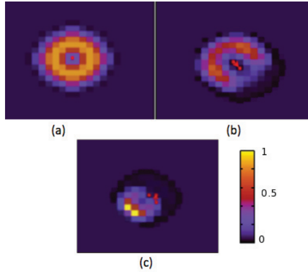
Figure A.5 – Représente l'évolution de la probabilité de contenir la cible pour chaque cellule de la grille, en utilisant trois mesures sur une même profondeur. Les trois emplacements du véhicule sont représentés par des croix.
