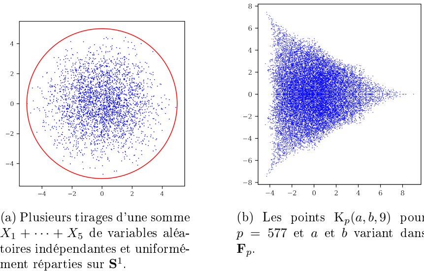
Figure 3: Deux comportements différents de sommes exponentielles dont le module est borné respectivement par 5 et par 9.
