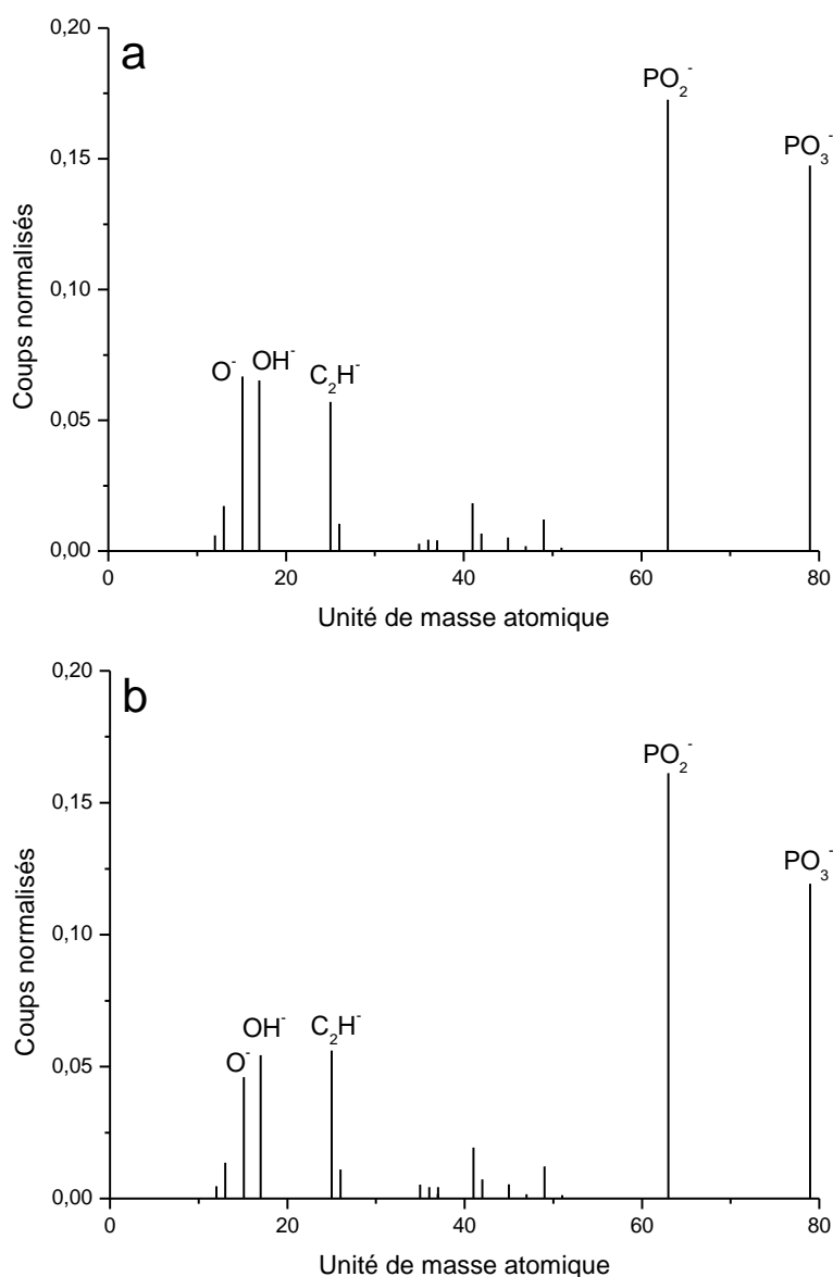
Figure 110: Spectres ToF-SIMS négatifs de HAG vierge (a) et HAG irradié sous UV (b).
