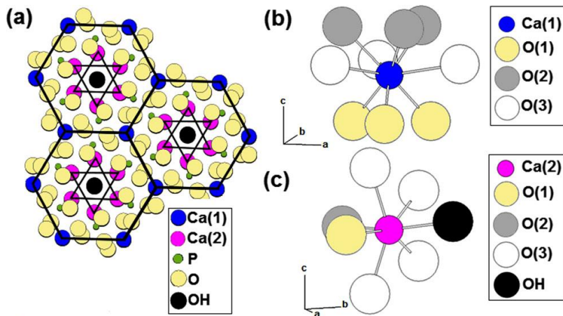
Figure 1: (a) Projection du plan (001) de la maille d'hydroxyapatite sur le plan xy, (b) environnement atomique des sites Ca (1) et (c) environnement atomique des sites Ca (2) (Zougrou et al., 2016).
