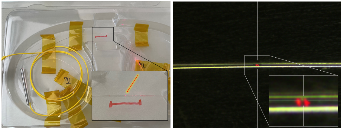
Figure 5.14: Image de gauche : photo avec le miroir semi-réfléchissant mis en valeur par un laser passant dans la fibre. Photo de droite : image faite au microscope du miroir semi-réfléchissant.
