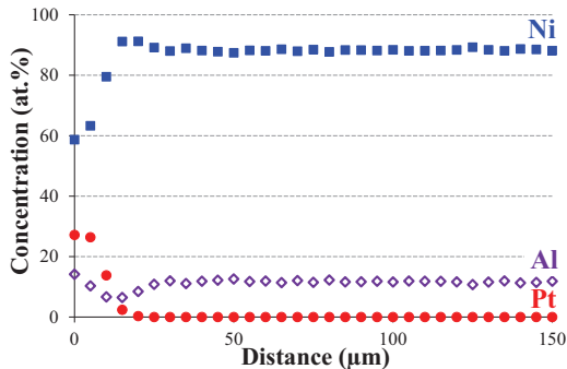
Figure IV-10 : Profils initiaux pour la modélisation c'est-à-dire état diffusé après 15min à 1100°C
