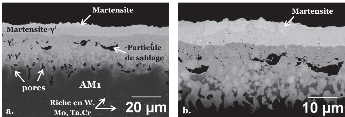
Figure III-4 : Images MEB en coupe transverse du revêtement \gamma\text{-}\gamma' Pt+Al de référence issu de la deuxième série d'élaboration, après 1 cycle à 1100^\circ\text{C} : référence 7/5 (échantillon 6,9/4,3). La figure b. est un agrandissement de la figure a. (mode BSE)
