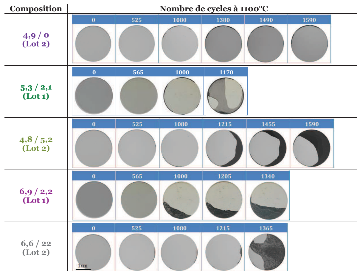
Figure III-42 : Evolution de l'écaillage de la barrière thermique au cours du cyclage pour un système de chaque composition cible
