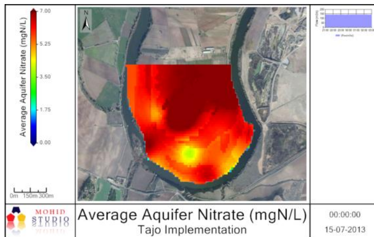
Figure 6-15: Concentrations en nitrates simulées sur le site du Tago après deux mois de simulation
