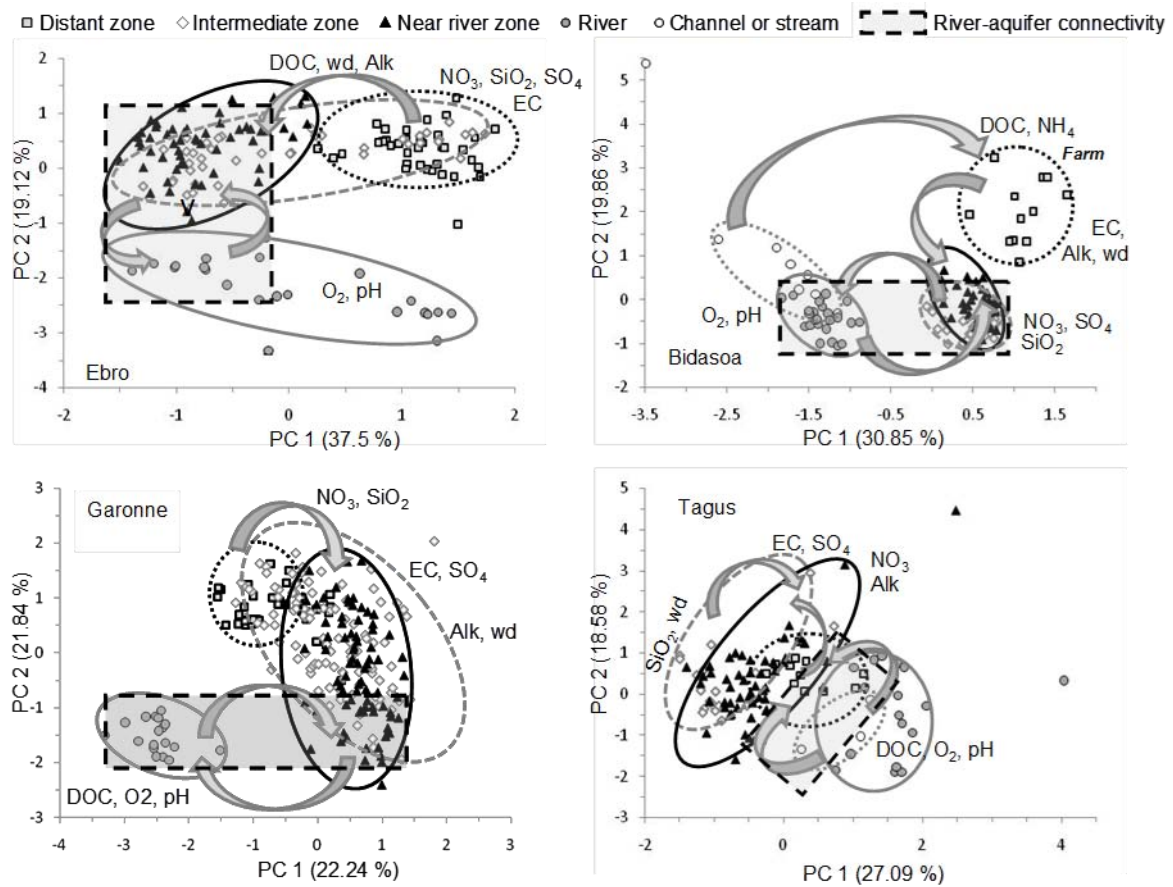
Figure 6-4 : Evolution spatiale des caractéristiques des eaux en fonction de leurs groupes (voir description dans le texte) dans le plan factoriel I-II de l'ACP effectuée pour chaque site. La connectivité entre la rivière et la zone proche de la rivière (NR) est également indiquée (cadre pointillé). Les flèches représentent les échanges entre les différents groupes (extrait de Antiguada et al., submitted).
