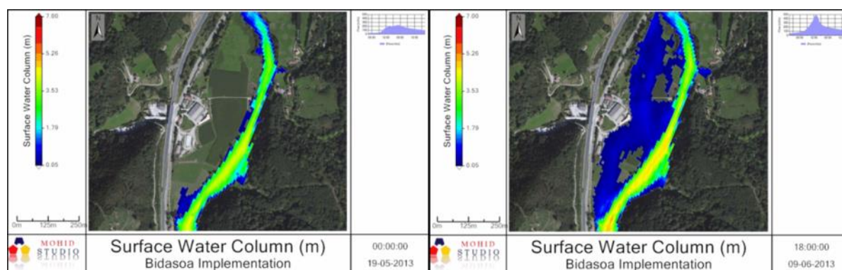
Figure 6-10 : Hauteur d'eau pour des crues correspondant à un débit de 200 \text{ m}^3/\text{s} (gauche) et 500 \text{ m}^3/\text{s} (droite), http://attenagua.actionmodulers.dtdns.net/
