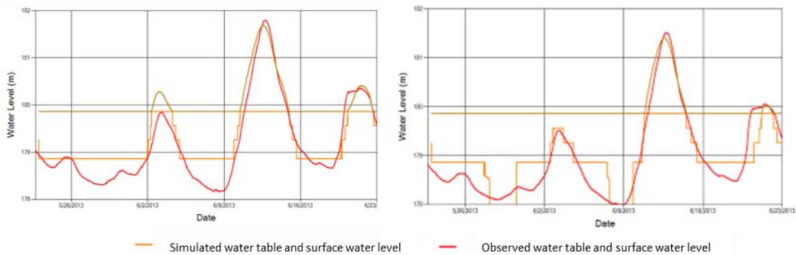
Figure 6-7 : Niveau piézométrique observé et simulé dans deux piézomètres situés dans le site de l'Ebre (Brito, 2014b)
