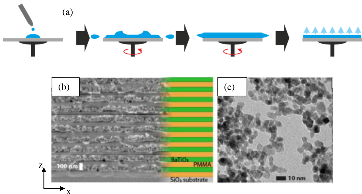
Figure 3.1: (a) Schéma du procédé de dépôt des couches minces par la technique de Spin Coating. (b) Image SEM du super-réseau constitué des couches de PMMA et BaTiO 3 . (c) Image TEM des nanoparticules de BaTiO 3 dans la couche hybride de type BaTiO 3 .
