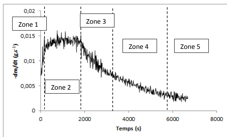
Figure 5.E.3 : Courbe de dérivée de la masse en fonction du temps - Solution de nitrate de fer nonahydraté ( T = 60\text{ °C} ).
