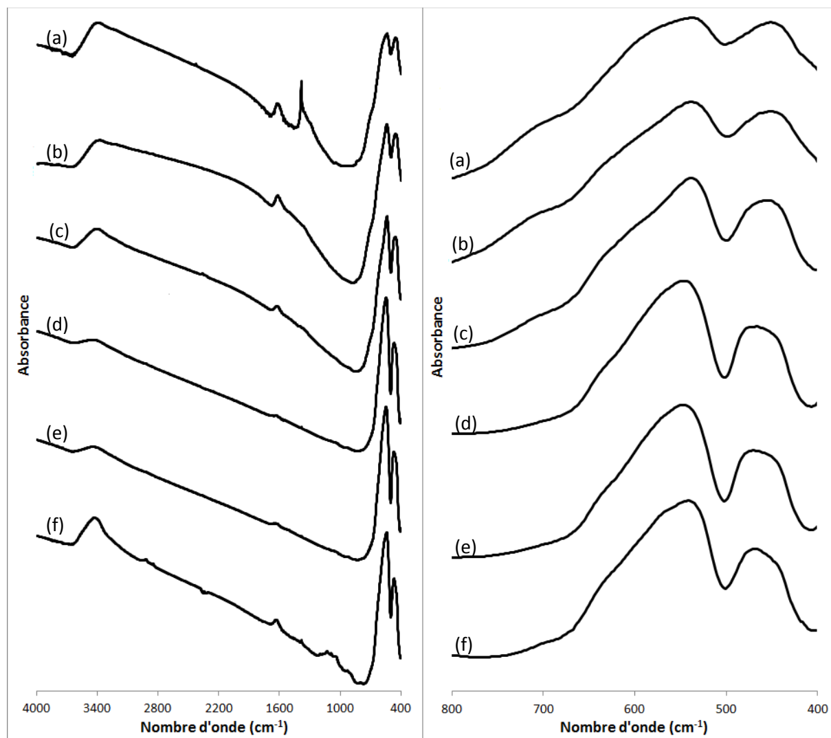
Figure 5.21 : Spectres infrarouge des produits obtenus au cours de la quatrième étape et de l'hématite de référence : (a) T = 200\text{ °C} , (b) T = 250\text{ °C} , (c) T = 300\text{ °C} , (d) T = 400\text{ °C} , (e) T = 500\text{ °C} et (f) hématite de référence.
