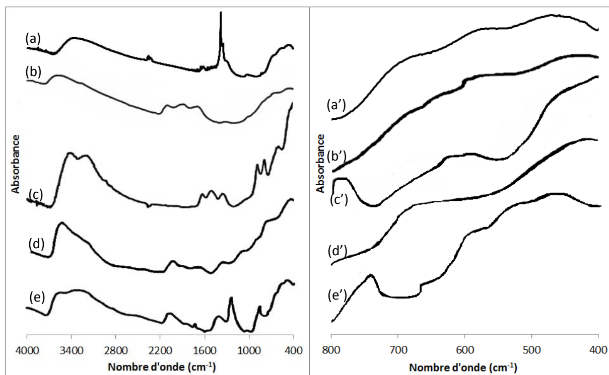
Figure 3.25 : Spectres infrarouge du produit du cyclone (a) et (a'), du \text{Fe}(\text{OH})_3 (b) et (b') (Lumme et Tummavuori, 1973) et des différentes formes du \text{FeOOH} : goethite (c) et (c') (Fan et al., 2006), ferroxhyte (d) et (d') (Carlson et Schwertmann, 1980) et lépidocrocite (e) et (e') (Gust, 1991).
