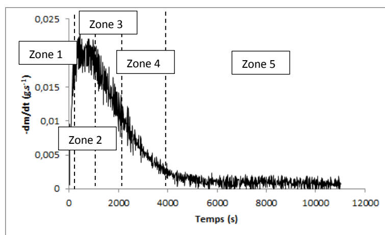
Figure 5.E.4 : Courbe de dérivée de la masse en fonction du temps - Solution de nitrate de fer nonahydraté ( T = 80\text{ °C} ).
