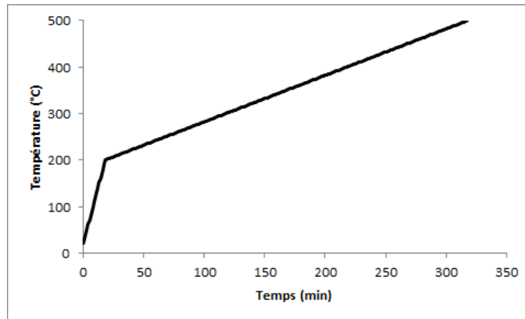
Figure 6.2 : Protocole opératoire de l'étude cinétique de la transformation de la ferrihydrite en hématite (exemple avec une vitesse de montée en température de 1\text{ °C.min}^{-1} entre 200 et 500 °C).
