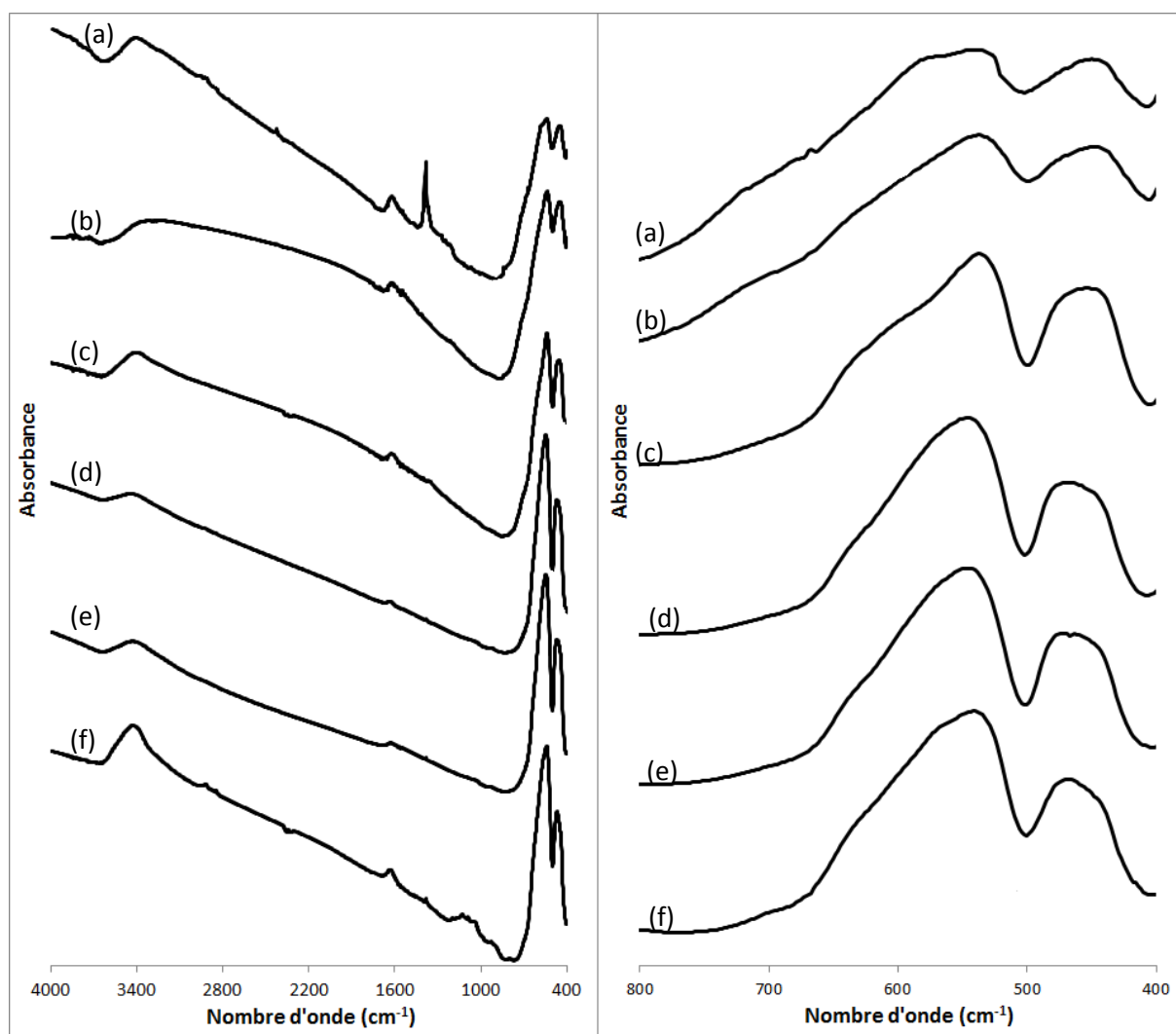
Figure 5.D.3 : Spectres infrarouge des produits obtenus au cours de la quatrième étape et de l'hématite de référence : (a) T = 200 °C, (b) T = 250 °C, (c) T = 300 °C, (d) T = 400 °C, (e) T = 500 °C et (f) hématite de référence.
