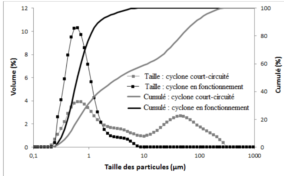
Figure 4.8 : Distributions de taille des particules issues du procédé pour les essais 11 et 12.
