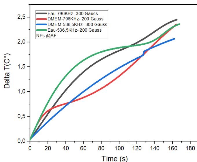
Figure V-8 : Températures des NPs @ AF (50nm) sous un champs magnétique alternative dans le DMEM et l'eau à 536,5 et 796 KHz.
