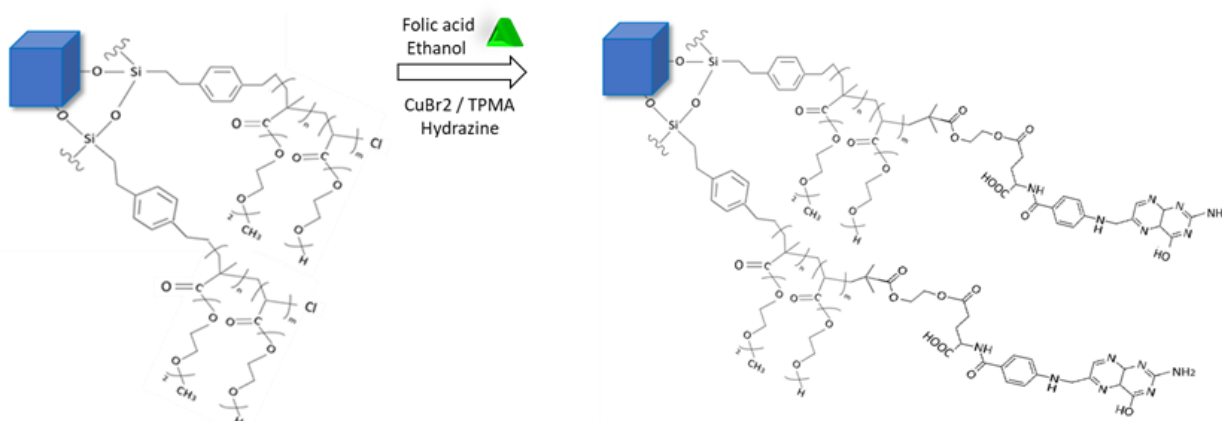
Figure V-2 : Modification des NPs@ P(MEO 2 MA 60 OEGMA 40 ) par l'acide folique.
