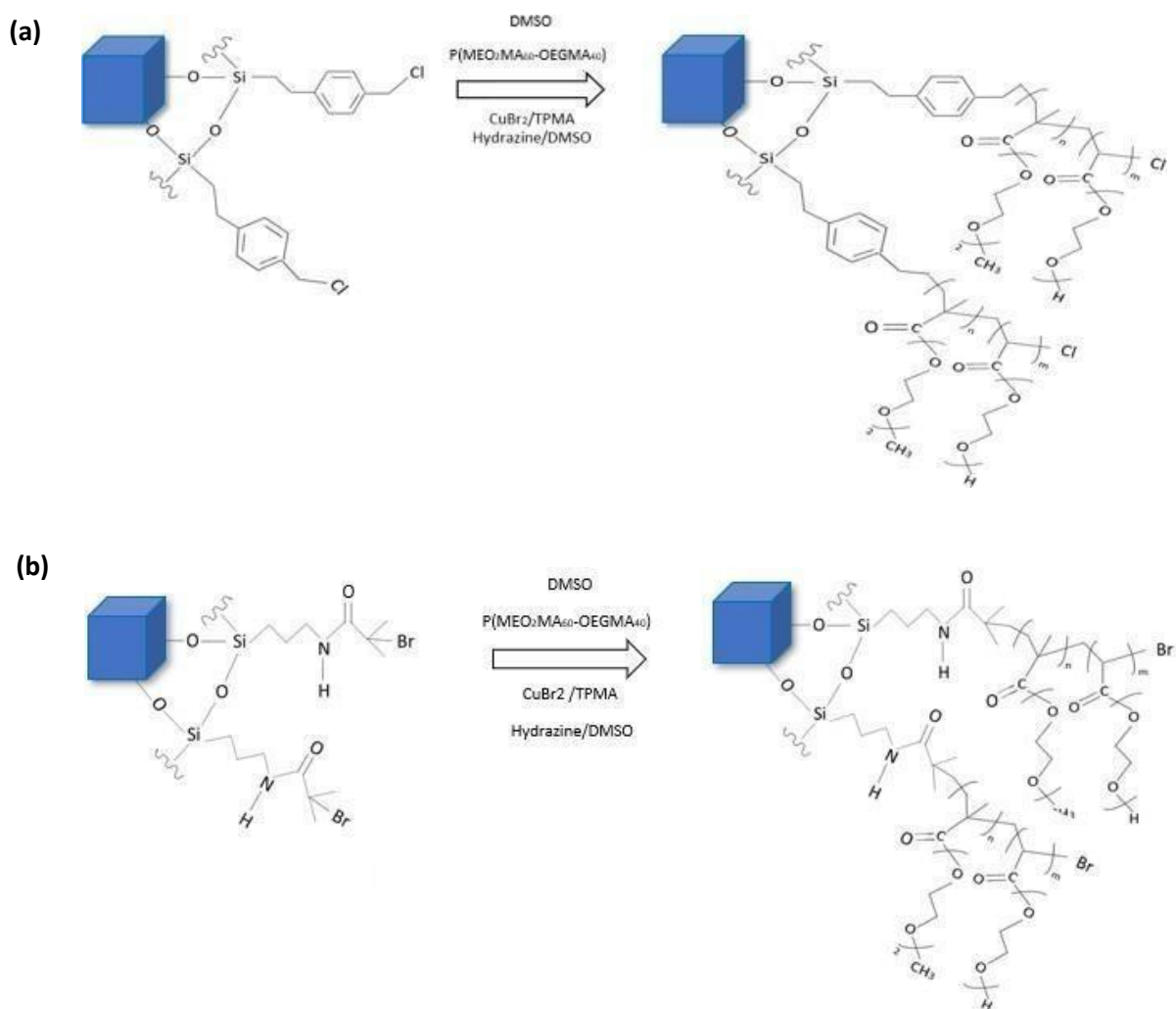
Figure III-4 : Schémas de la polymérisation des NPs @CMPETMS (a) et des NPs@APTMS-BIBB par le P(MEO 2 MA 60 OEGMA 40 ) (b).
