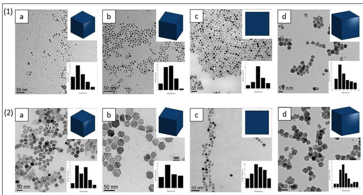
Figure II-6 : (1) Images MET (fond clair /bright field) des NPs Zn_{0.4}Fe_{2.6}O_4 : 5nm (a), 10nm (b), 18nm (c) et 45nm (d). (2) Images MET des NPs Zn_{0.4}Fe_{2.6}O_4@MnFe_2O_4 : 10nm (a), 15nm (b), 22nm (c) et 50nm (d).
