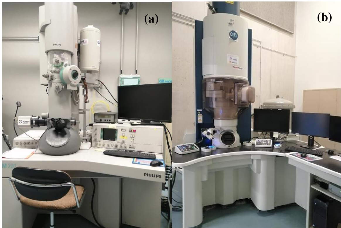
Figure 15 : (a) MET Philips CM200. (b) MET-HR JEOL JEM - ARM 200F.
