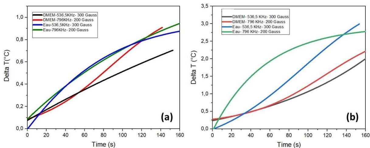
Figure III-18 : Températures des NPs @ P(MEO 2 MA 60 OEGMA 40 ) de 22nm (a) et des 50nm
