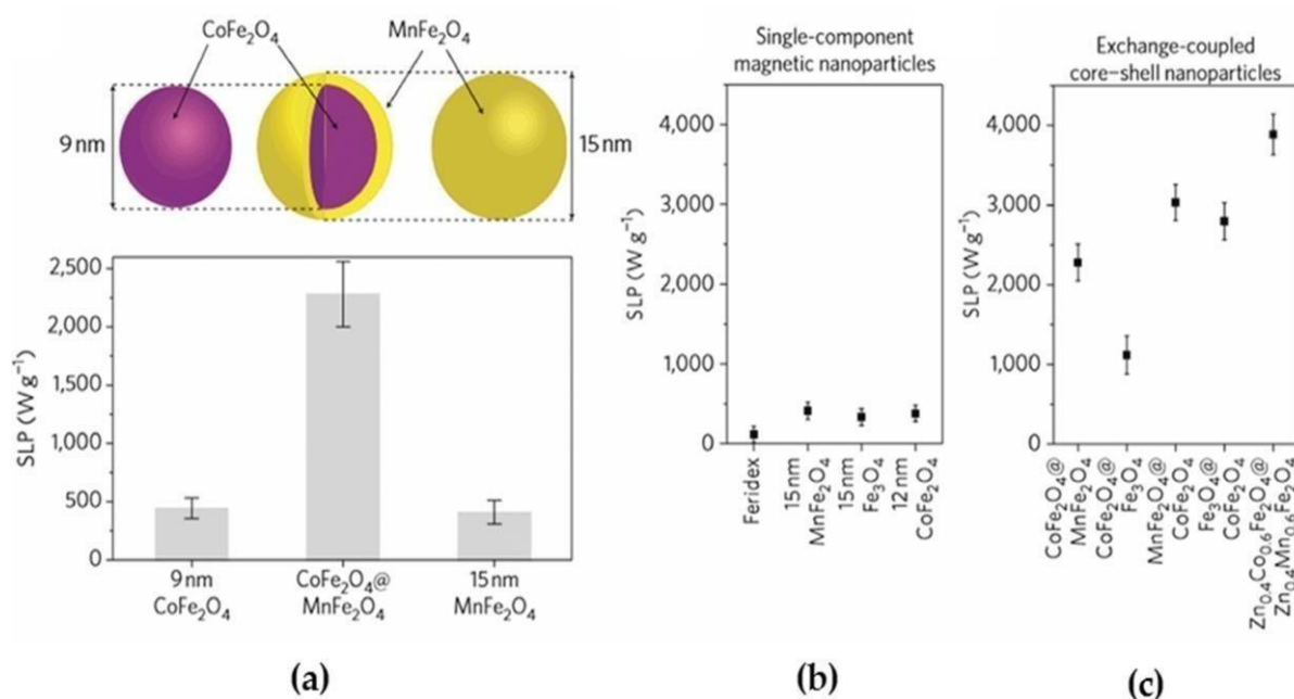
Figure I-15 : Nanoparticules \text{CoFe}_2\text{O}_4@15\text{ nm MnFe}_2\text{O}_4 et leurs valeurs de la SLP comparées à celles obtenues par les nanoparticules \text{CoFe}_2\text{O}_4 (cœur seul) et \text{MnFe}_2\text{O}_4 (coquille seule) (a). Valeurs de la SLP des nanoparticules \text{MnFe}_2\text{O}_4 , \text{Fe}_3\text{O}_4 , \text{CoFe}_2\text{O}_4 (b) et les cœur@coquille de \text{CoFe}_2\text{O}_4@15\text{ nm MnFe}_2\text{O}_4 , \text{CoFe}_2\text{O}_4@15\text{ nm Fe}_3\text{O}_4 , \text{MnFe}_2\text{O}_4@15\text{ nm CoFe}_2\text{O}_4 , \text{Fe}_3\text{O}_4@15\text{ nm CoFe}_2\text{O}_4 et \text{Zn}_{0.4}\text{Co}_{0.6}\text{Fe}_2\text{O}_4@15\text{ nm Zn}_{0.4}\text{Mn}_{0.6}\text{Fe}_2\text{O}_4 (c) 66 .
