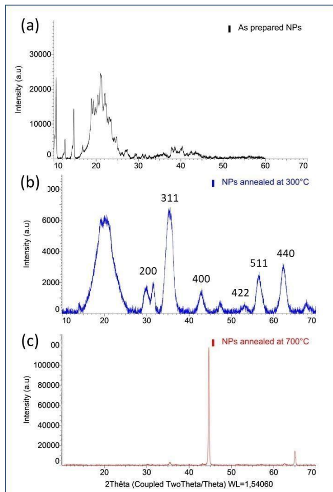
Figure II-4 : Diffractogrammes RX des NPs telles qu'elles sont préparées (a), après recuit à 300^\circ\text{C} (b) et à 700^\circ\text{C} (c).
