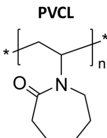
Figure I-22 : Structure chimique du Poly( N -vinylcaprolactame) (PVCL) 98,112 .
