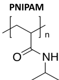
Figure I-21 : Structure chimique du Poly( N -isopropylacrylamide) (PNIPAM) 98 .
