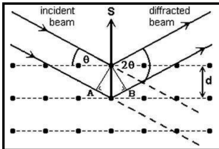
Figure 1 : Illustration schématique de la DRX lorsque la loi de Bragg est satisfaite 2 .
