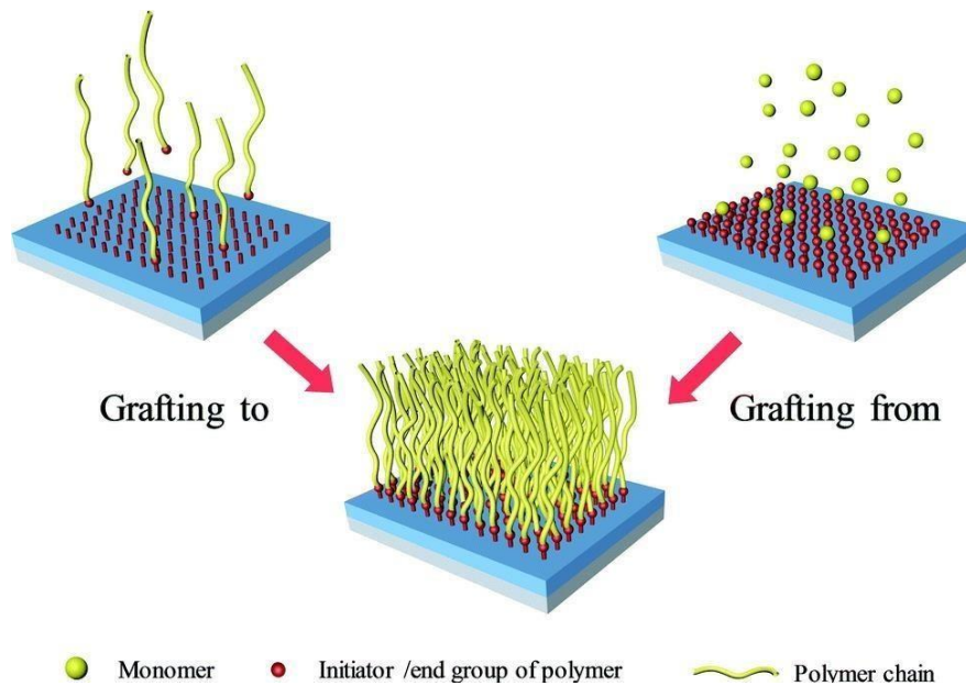
Figure I-26 : Schéma des deux méthodes de greffage du polymère « grafting to » et « grafting from » 131 .
