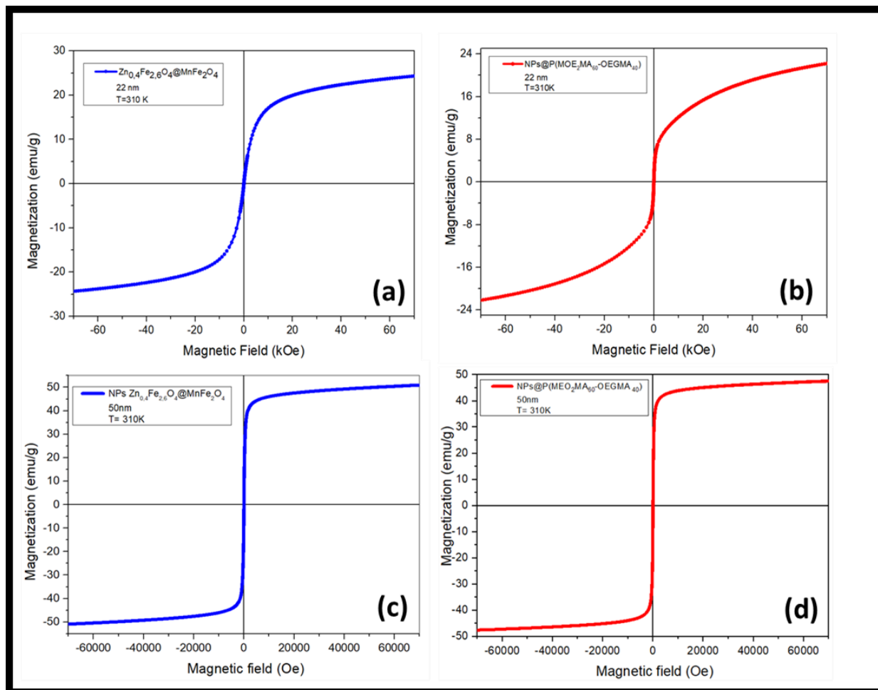
Figure III-12 : Valeurs de la magnétisation en fonction du champs magnétique des NPs Zn 0.4 Fe 2.6 O 4 @ MnFe 2 O 4 22nm (a) , des NPs@ P(MEO 2 MA 60 OEGMA 40 ) 22nm (b), des NPs Zn 0.4 Fe 2.6 O 4 @ MnFe 2 O 4 50nm(c) et des NPs@ P(MEO 2 MA 60 OEGMA 40 ) 50nm (d).
