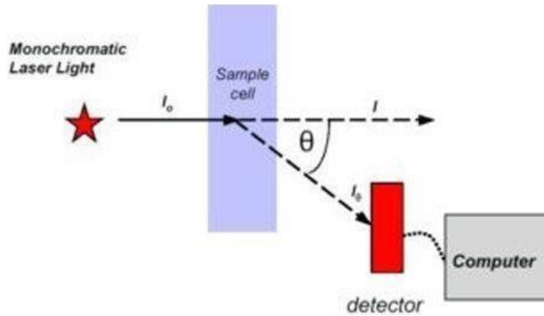
Figure 12 : Schéma représentatif de la DLS.
