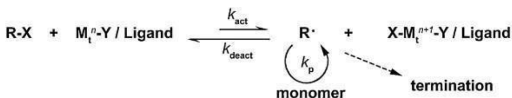
Figure I-27: Schéma du mécanisme ATRP proposé par Matyjaszewski et al. 142 .
