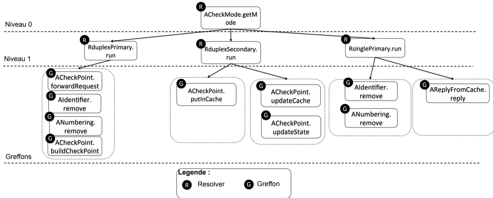
FIGURE 5.6 – Arborescence de résolveurs utilisée pour la résolution des interactions coté serveur.
