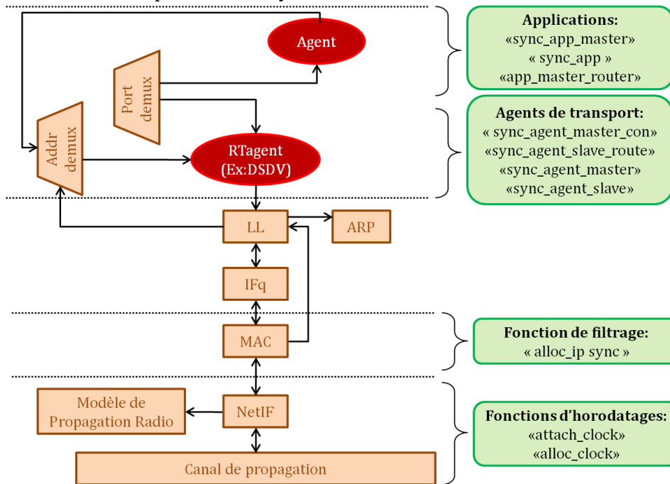
Figure III.10 Intégration de l'IEEE-1588 dans l'architecture du logiciel NS-2.
