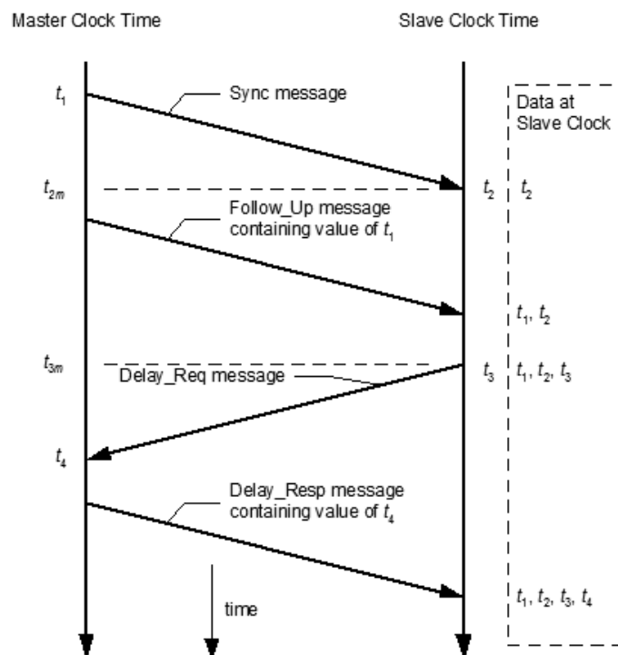
Figure V.10 Fonctionnement d'IEEE-1588 40 .
