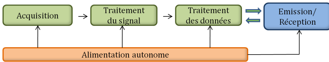
Figure I.2 Les principaux composants matériels d'un nœud capteur.
