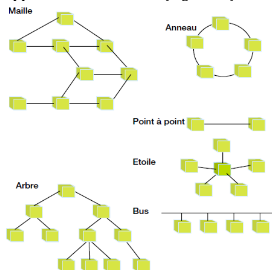
Figure I.9 Exemple de réseau bus de terrain 7 .
