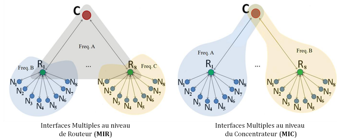
Figure V.5 Deux scénarios d'organisations du réseau avec des interfaces multiples.
