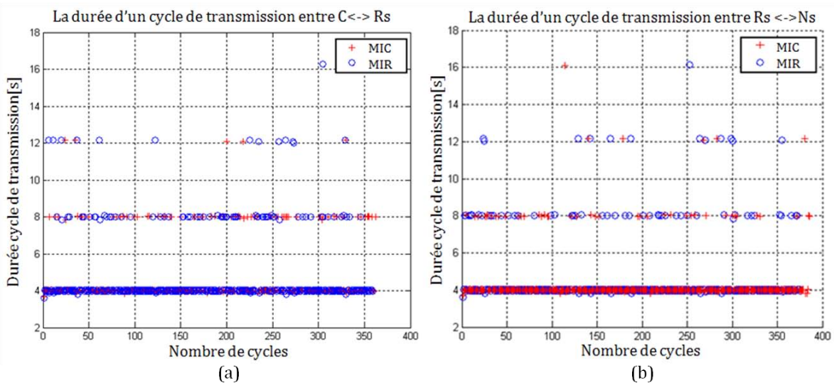
Figure V.7 Durée cycle de transmission entre C-Routers et R-Nœuds.
