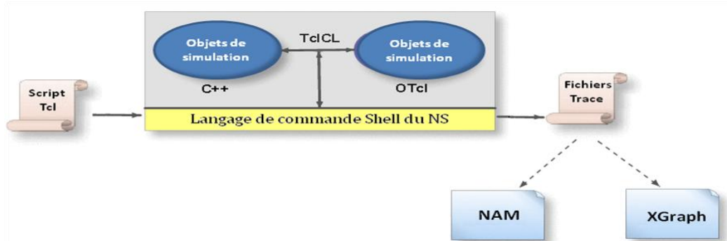
Figure I.15 L'architecture de base pour le simulateur NS-2.
