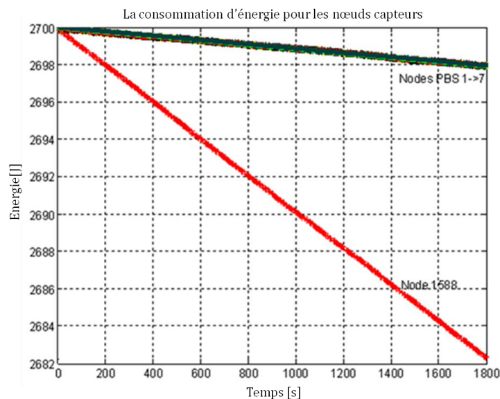
Figure V.26 La consommation d'énergie pour les nœuds du réseau.
