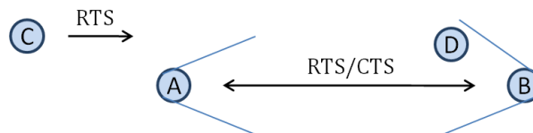
Figure IV.2 Le problème de nœuds cachés.
