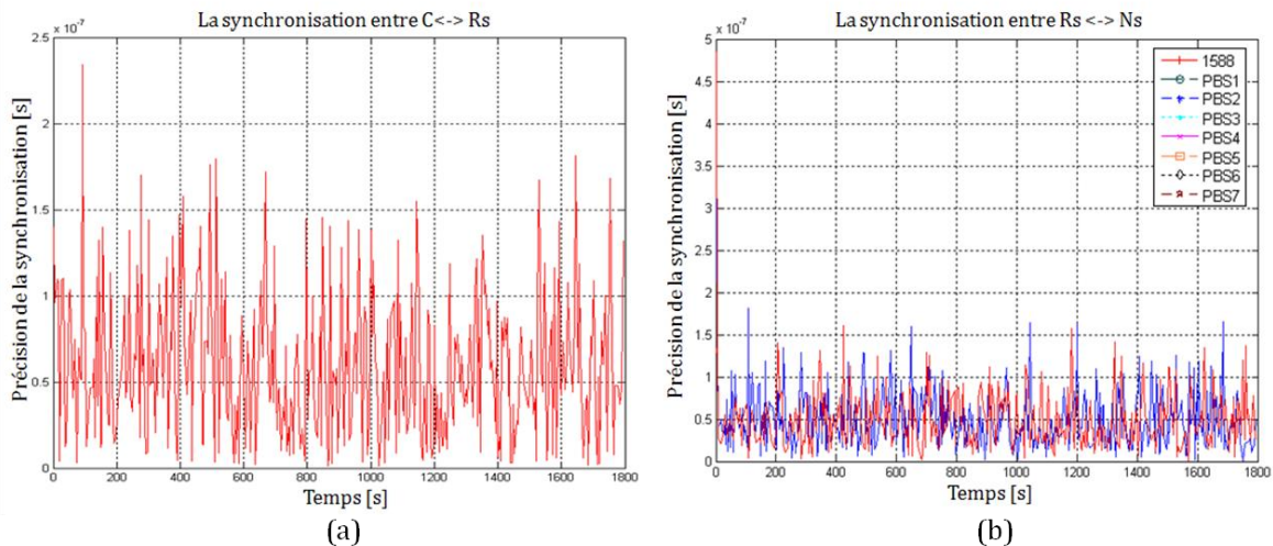
Figure V.27 Synchronisation du Niveau 1 et Niveau 2 avec Directional-TDMA MAC.
