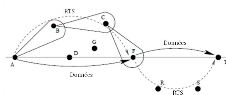
Figure IV.7 Le mécanisme de fonctionnement du MMAC protocole.
