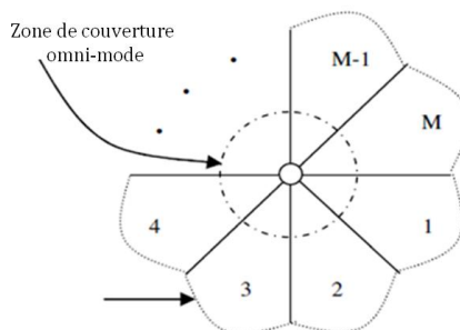
Figure IV.8 Le protocole DMAC Circulaire.
