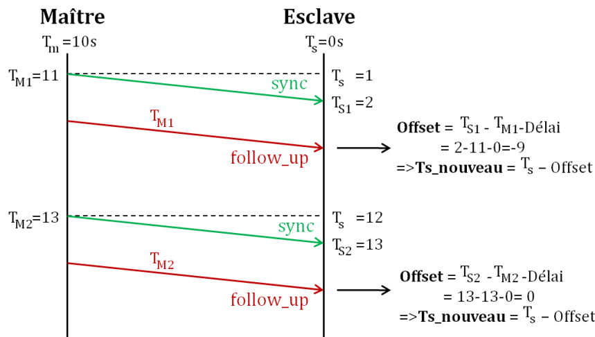
Figure III.1 La première phase de synchronisation de l'IEEE-1588.
