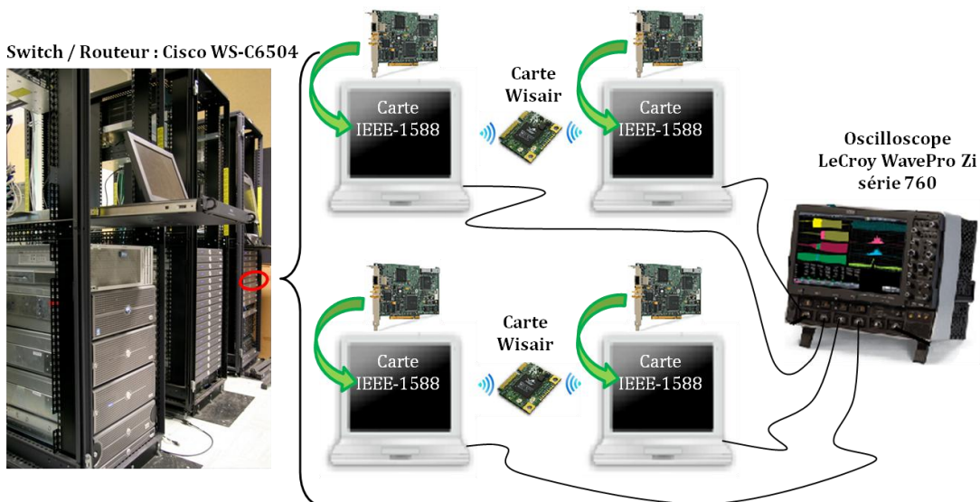
Figure V.9 Plate-forme d'expérimentation.
