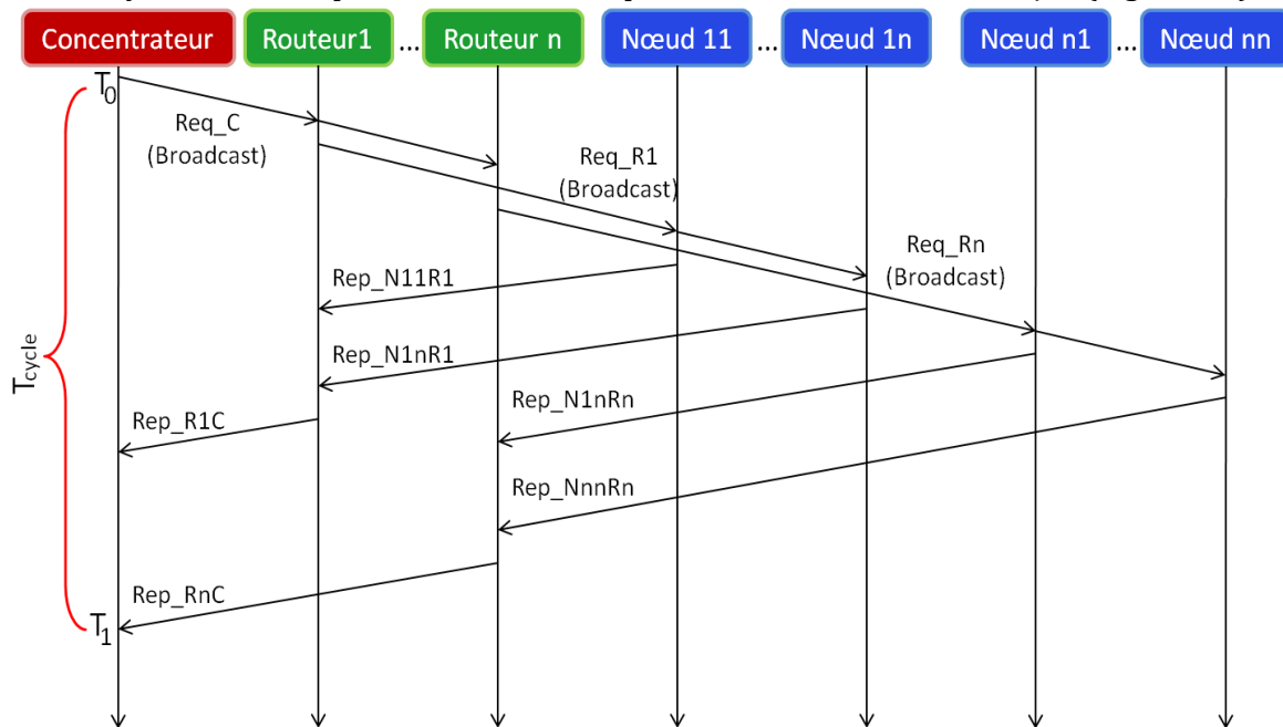
Figure V.2 Le temps d'un cycle de communication (cycle normal de données).
