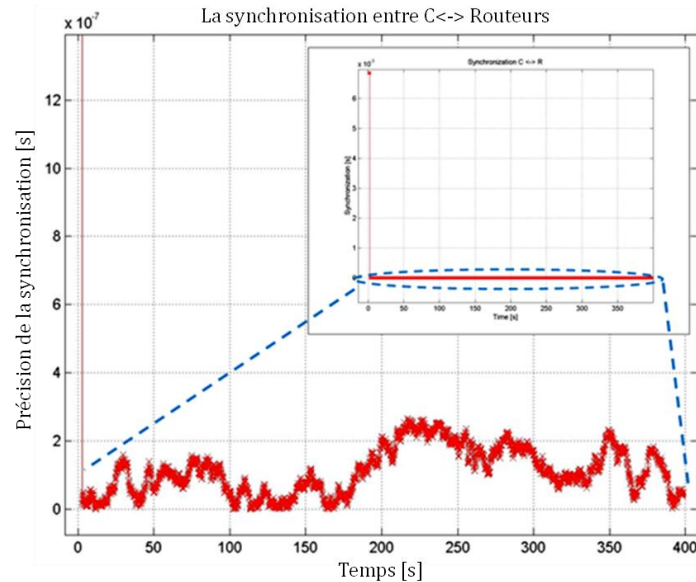
Figure V.24 La synchronisation entre C <-> Rs pour l'IEEE1588-PBS hybride.
