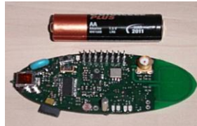
Figure I.4 Nœud capteur du projet EYES.
