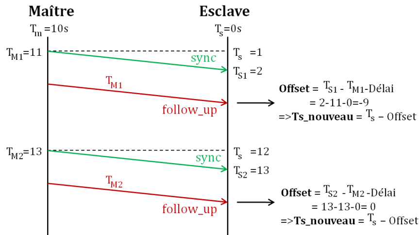
Figure III.1 La première phase de synchronisation de l'IEEE-1588.
