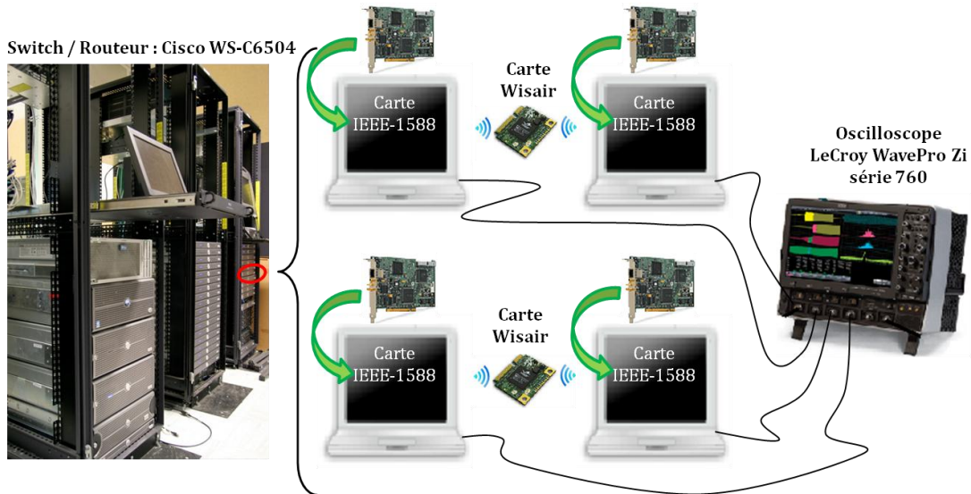
Figure V.9 Plate-forme d'expérimentation.
