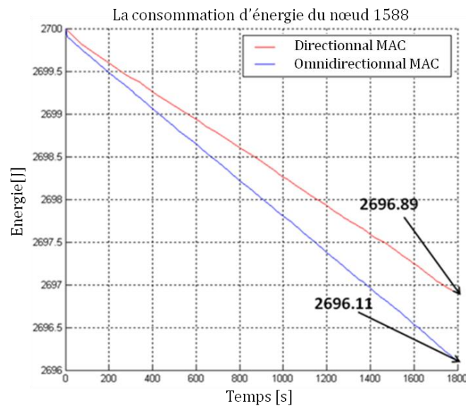
Figure V.29 Consommation en énergie des nœuds 1588.
