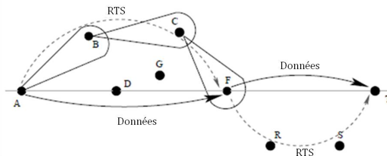
Figure IV.7 Le mécanisme de fonctionnement du MMAC protocole.
