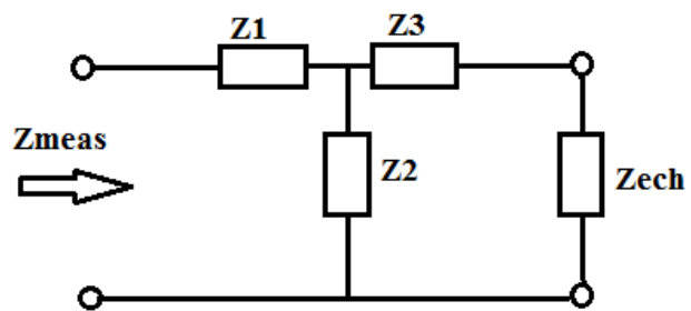
Figure 9 Circuit équivalent du système de mesure
