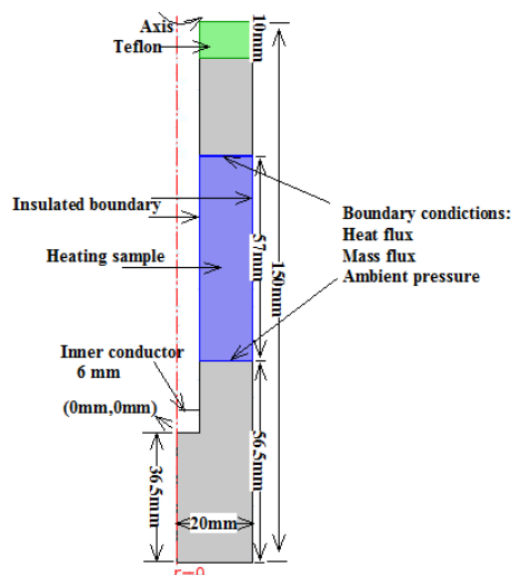
Figure 11 Le schéma de modèle 2D axisymétrique
