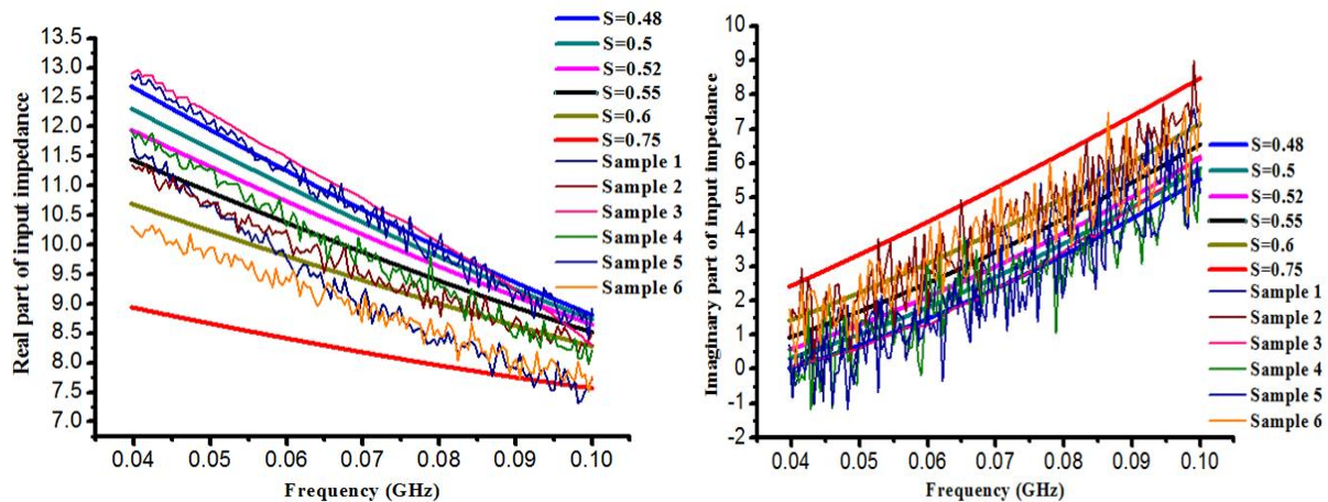
Figure 10 Comparaison des impédances d'entrées mesurées et simulées:
