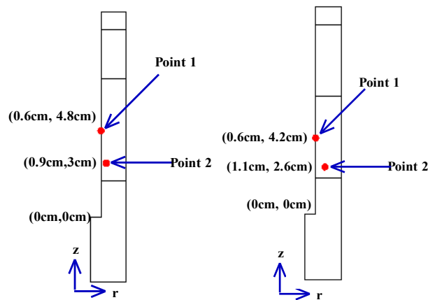
Figure 13 Positions des deux points pour mesurer la température : hauteur de l'échantillon est de 57mm (à gauche); la hauteur de l'échantillon est de 45mm (à droite)
