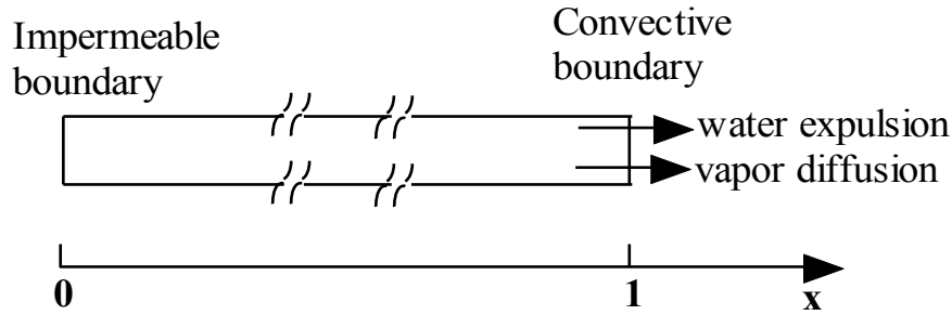
Figure 1 Schéma du modèle de brique 1D
