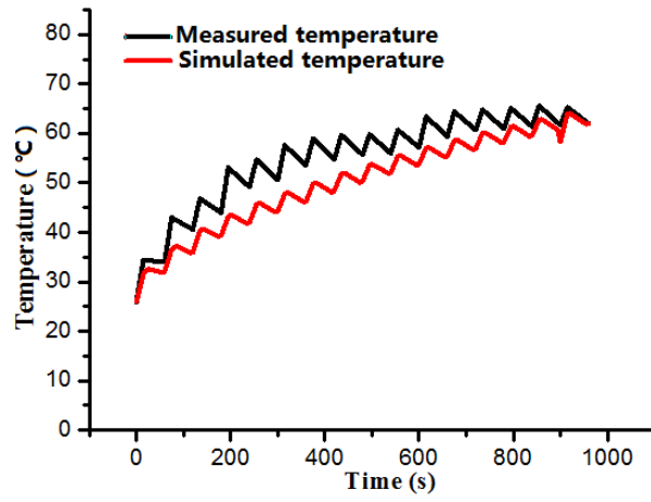
Figure 18 Changement de température du point 1 Figure 19 Changement de température du point 2
