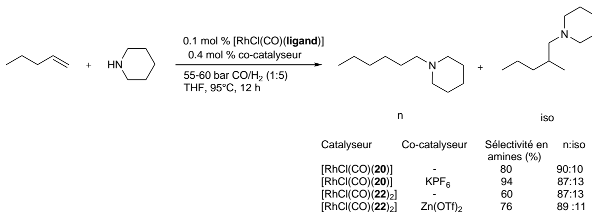
Schéma I. 10. Hydroaminométhylation du pent-1-ène avec piperidine, avec les ligands 20 et 22
