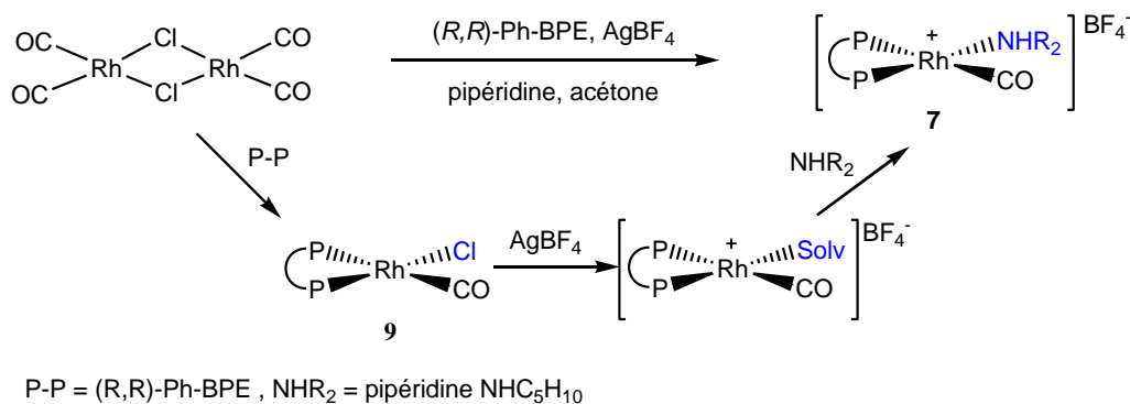
Schéma IV. 12. Synthèse du complexe [Rh(CO)(NHC_5H_{10})((R,R)\text{-Ph-BPE})]BF_4 7
