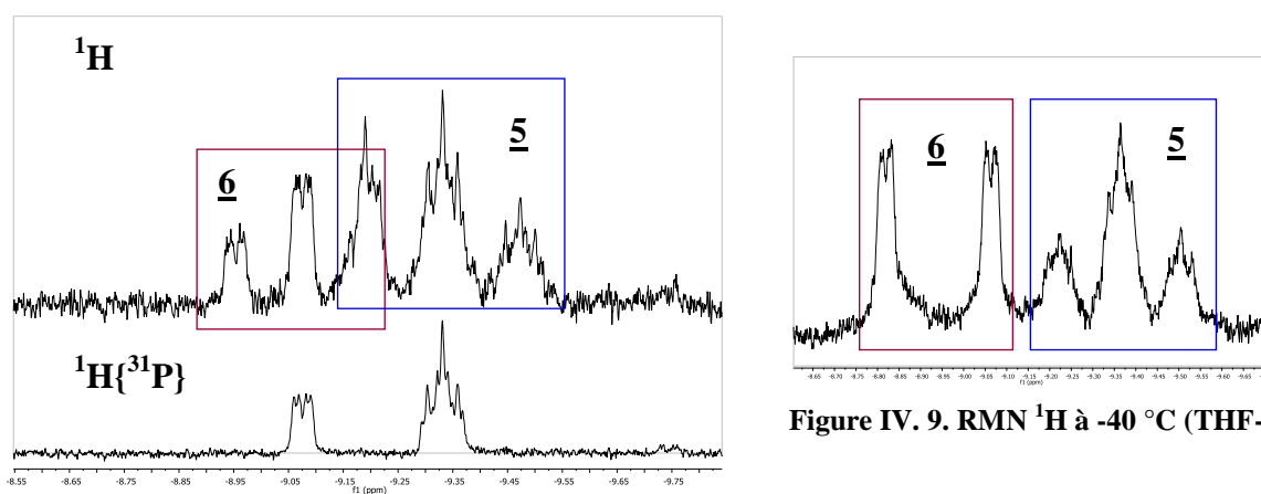
Figure IV. 10. Spectre RMN ^1\text{H} (haut) et ^1\text{H}\{^{31}\text{P}\} (bas) de la zone hydrure de l'espèce 6 (THF- d^8 , 25 °C).
