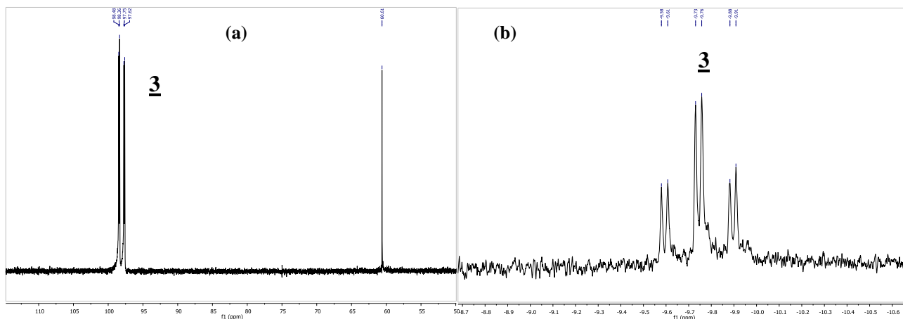
Figure IV. 29. Après 12 heures à 40°C, solution du système [\text{Rh}(\text{acac})(\text{CO})_2] / \text{Ph-BPE} en conditions d'HAM (a) spectre RMN ^{31}\text{P} (b) zone hydrure du spectre RMN ^1\text{H} ( \text{THF-d}^8 , spectre enregistré à 25 °C)
