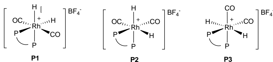
Schéma IV. 5. Structures possibles pour le complexe [\text{Rh}(\text{H})_2(\text{CO})_2((\text{R,R})\text{-Ph-BPE})]\text{BF}_4
