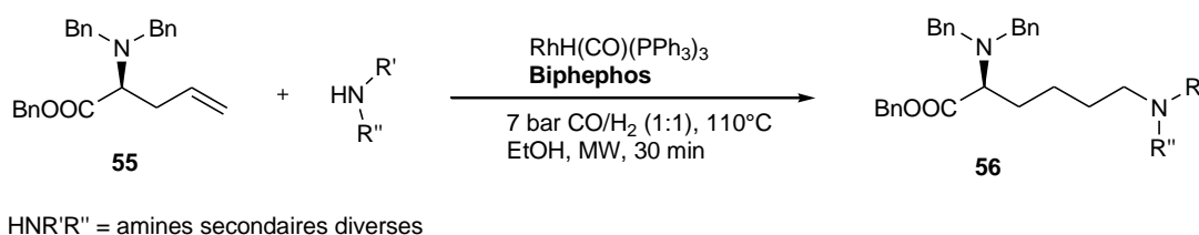
Schéma I. 26. Synthèse d' \alpha -aminoacides benzylés par hydroaminométhylation assistée aux micro-ondes
