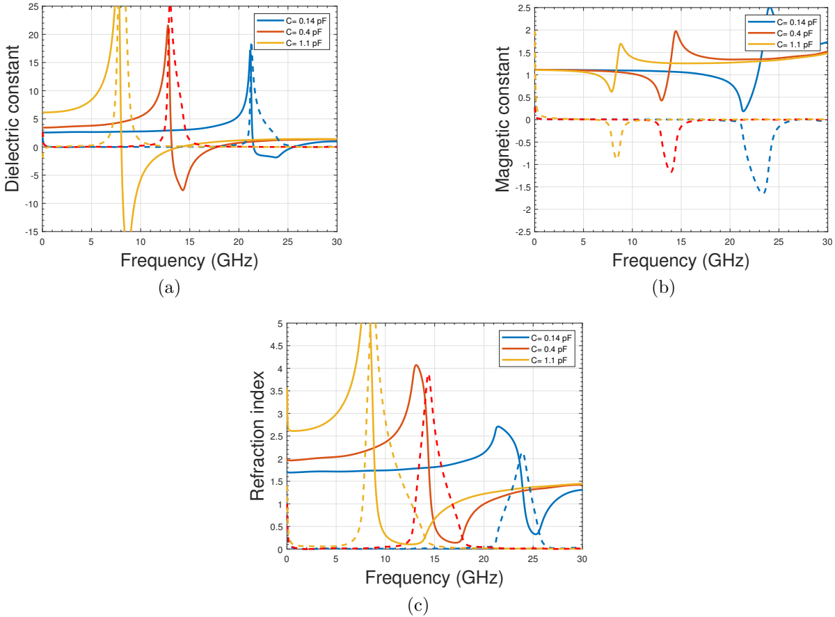
Figure 2.11 – UC parameters
