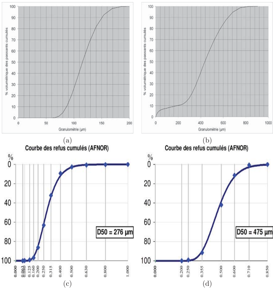
FIGURE 2.19 – Courbes granulométriques des sables (a) S110 ( D_{50} = 0,11 \text{ mm} ), (b) C412 ( D_{50} = 0,41 \text{ mm} ), (c) S276 ( D_{50} = 0,28 \text{ mm} ) et (d) S475 ( D_{50} = 0,48 \text{ mm} ). Les sables S110 et C412 ont été mesurés à l'aide d'un granulomètre laser, les courbes des sables S276 et S475 proviennent du fabricant.
