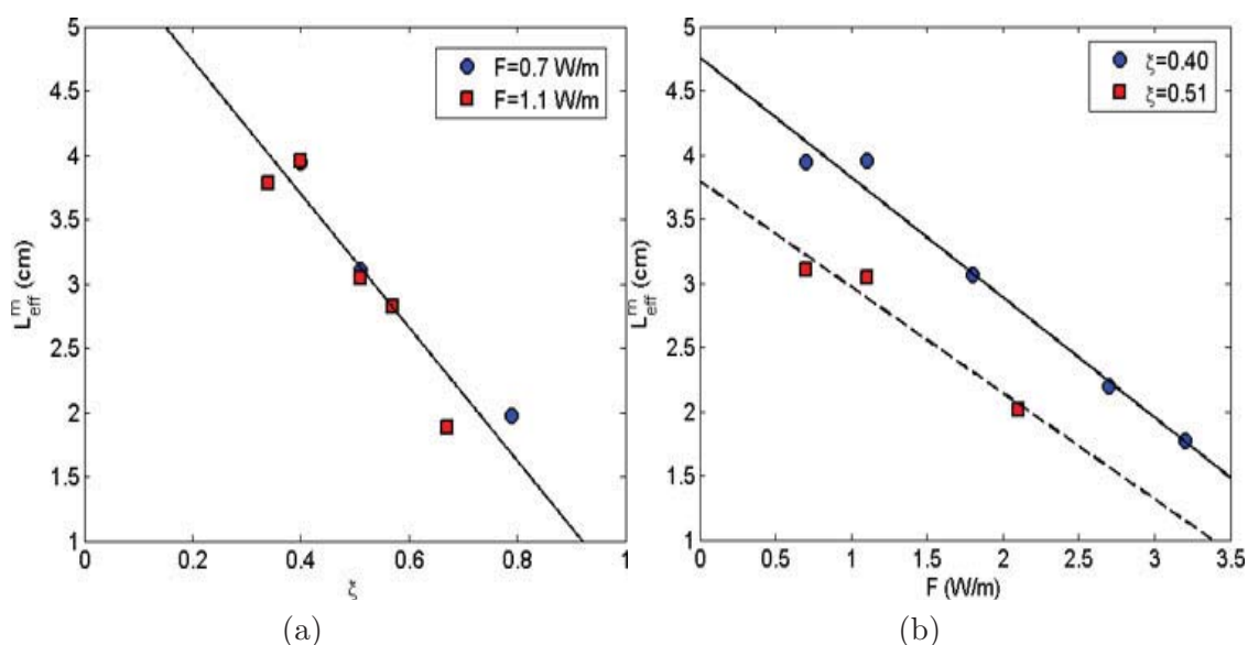
FIGURE 3.11 – Profondeur moyenne d’effondrement : (a) en fonction de \xi pour F = 0,7 W/m et F = 1,1 W/m, (b) en fonction de F pour \xi = 0,40 et \xi = 0,51 . (a) La droite (—) a pour équation L_{eff}^m = -5,2\xi + 5,8 . (b) La droite (—) a pour équation L_{eff}^m = -0,94F + 4,8 et la droite (- - -) a pour équation L_{eff}^m = -0,83F + 3,8 .
