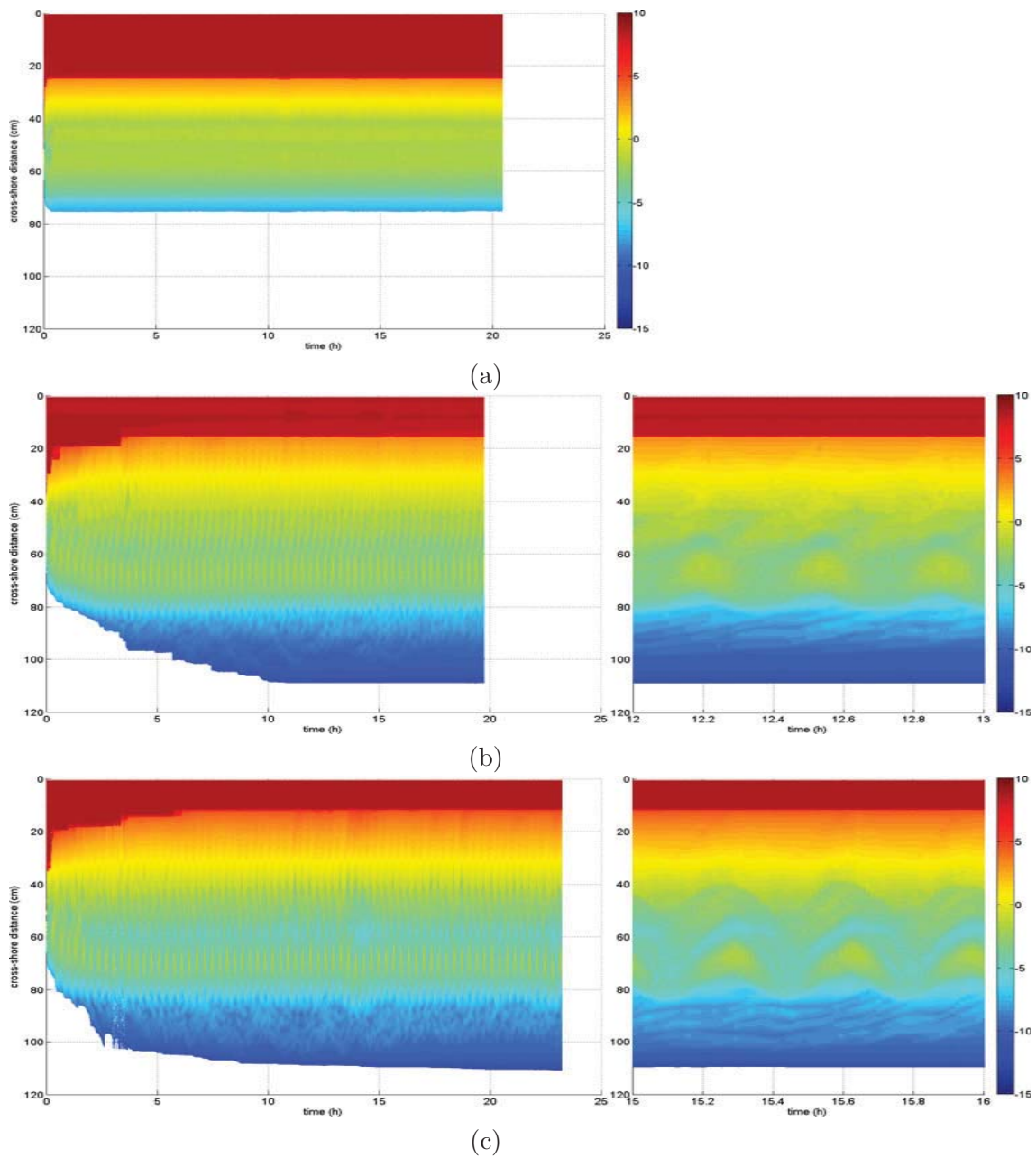
FIGURE 4.25 – Evolutions spatio-temporelles de la morphologie de la falaise et du fond de type T_3 . (a) sans marée et avec variation sinusoidale du niveau d'eau de période T_m = 20 \text{ min} et d'amplitude (b) A_m = 1 \text{ cm} et (c) A_m = 2 \text{ cm} .
