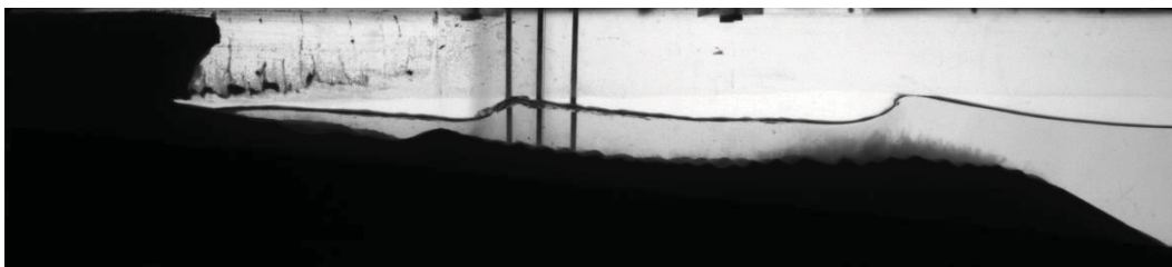
FIGURE 4.24 – Profil du fond et de la falaise pour une taille de grain de sable D_{50} = 0,11 mm.
