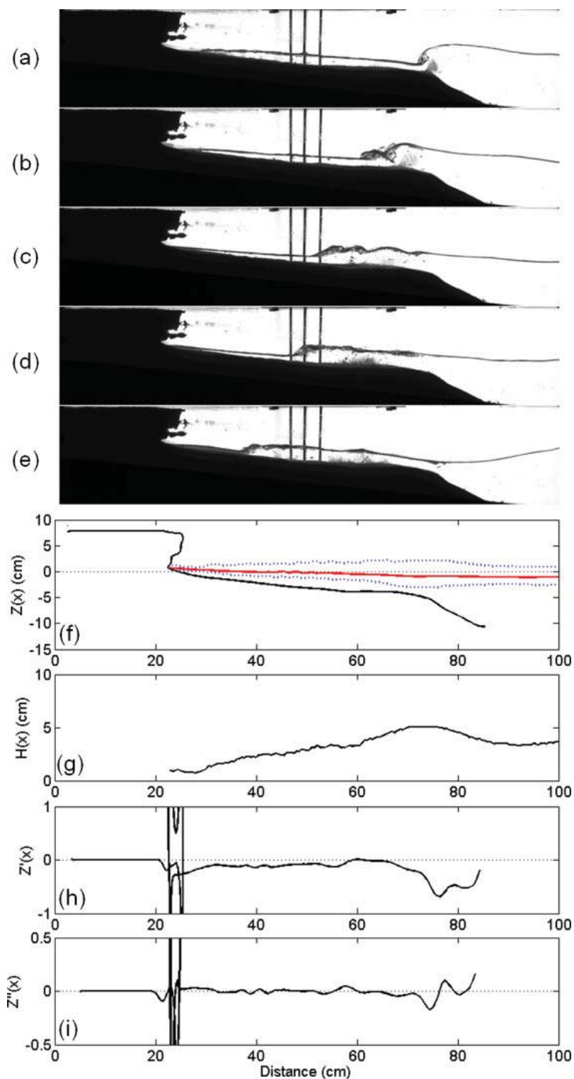
FIGURE 4.10 – Profil de fond de type T3 où la plateforme interne est à forte pente avec (F, \xi) = (0,9; 0,55) , x_C = 31,9 cm, x_R = 57,9 cm, x_M = 76,4 cm. (a)-(b)-(c)-(d)-(e) : Visualisation latérale. (f) : (—) Profils du fond Z(x) et (---) de la surface libre moyennés en temps, (...) enveloppe des vagues. (g) : Hauteur des vagues H(x) . Dérivées (h) première Z'(x) et (i) seconde Z''(x) du profil du fond Z(x) .
