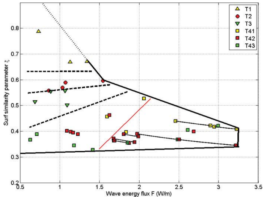
FIGURE 4.7 – Diagramme du type des fonds en fonction des paramètres de houle ( F; \xi ). Les frontières (---) délimitent les zones de morphologie différente. (—) limite entre les profils stationnaires et instationnaires pour le type T4. Les symboles reliés entre eux par une courbe pleine (—) représentent les cas instationnaires où les barres oscillent, les deux symboles correspondent aux forçages de houle pour les deux positions des barres.
