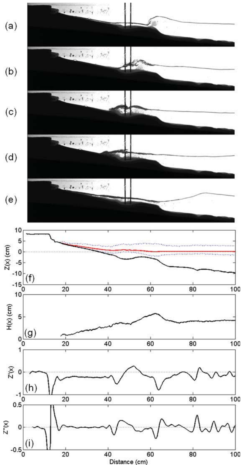
FIGURE 4.9 – Profil de fond de type T2 avec (F, \xi) = (1; 0, 57) , x_B = 17, 7 cm, x_C = 24, 2 cm, x_R = 42, 7 cm, x_M = 64, 7 cm. (a)-(b)-(c)-(d)-(e) : Visualisation latérale. (f) : (—) Profils du fond Z(x) et (—) de la surface libre moyennés en temps, (...) enveloppe des vagues. (g) : Hauteur des vagues H(x) . Dérivées (h) première Z'(x) et (i) seconde Z''(x) du profil du fond Z(x) .
