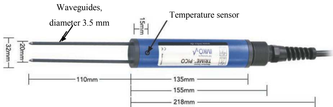
Fig. 5.12: TDR (Trime-Pico 32).
