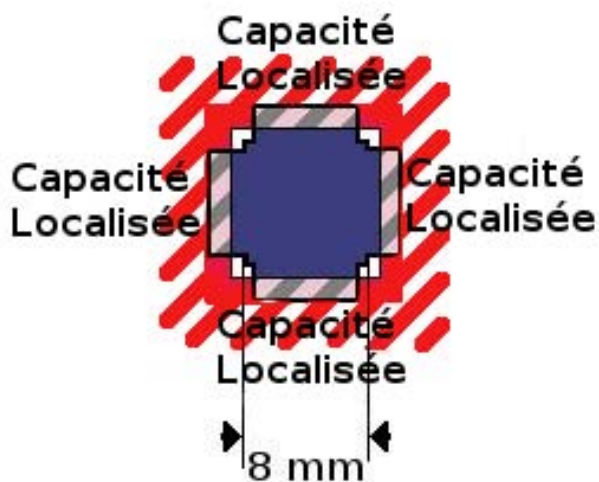
FIGURE 4.14 – Cellule-L1 avec des capacités localisées à l'intérieur de la cellule-L5
