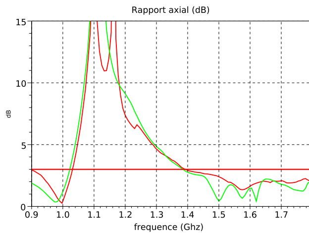
FIGURE 6.7 – Rapport axial mesuré pour le dipôle à 1GHz à 25mm au-dessus de la SHI en vert et en rouge le même dipôle à \lambda_1/4 d'un CEP
