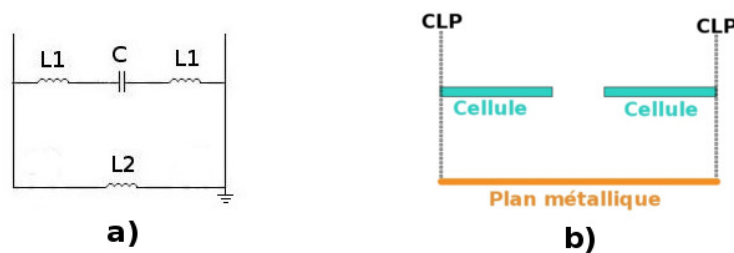
FIGURE 4.8 – a) CEE plus détaillé pour une cellule sans via miniaturisée et b) cellule équivalente en simulation sous HFSS vue en coupe
