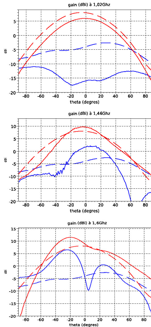
FIGURE 6.8 – Diagramme de rayonnement en gain mesuré pour le dipôle à 1GHz à 25mm au-dessus de la SHI en rouge le gain RHCP, et en bleu foncé le gain LHCP et respectivement pour les mêmes couleurs avec des tirets la même chose pour le même dipôle à \lambda_1/4 d'un CEP
