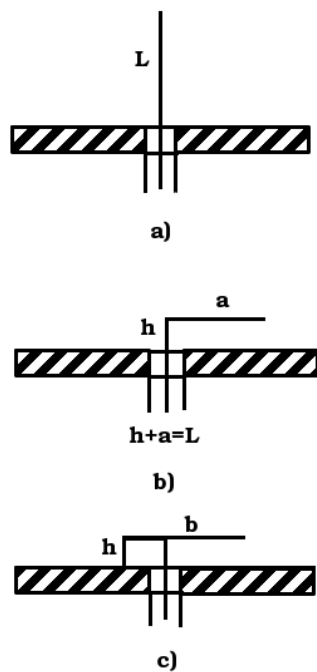
FIGURE 2.7 – Repliement d'un monopôle au-dessus d'un plan métallique a) monopôle b) monopôle replié (ILA) c) PIFA.
