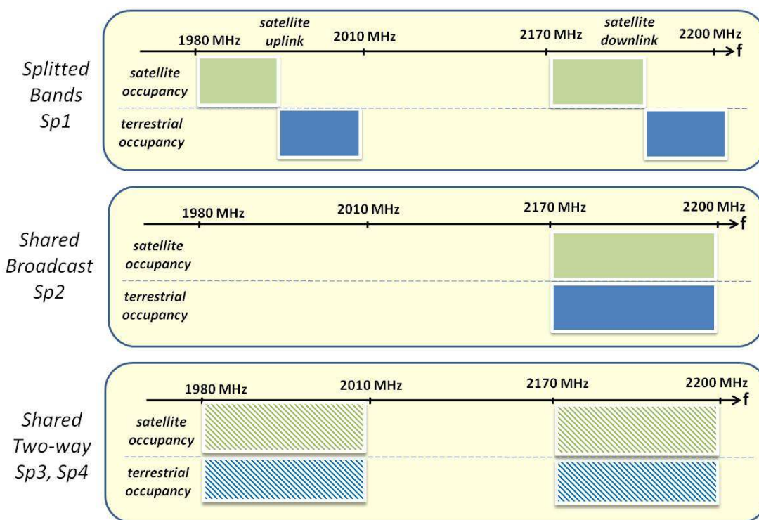
Figure 1-8 : Possibilités de répartition de fréquence entre systèmes satellite et terrestre (bande S).
