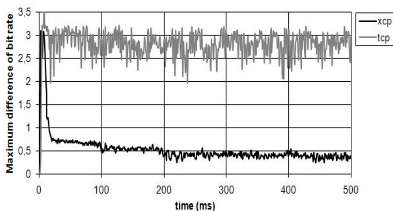
Figure 3-11: Ecart maximum entre les flux (XCP et TCP)
