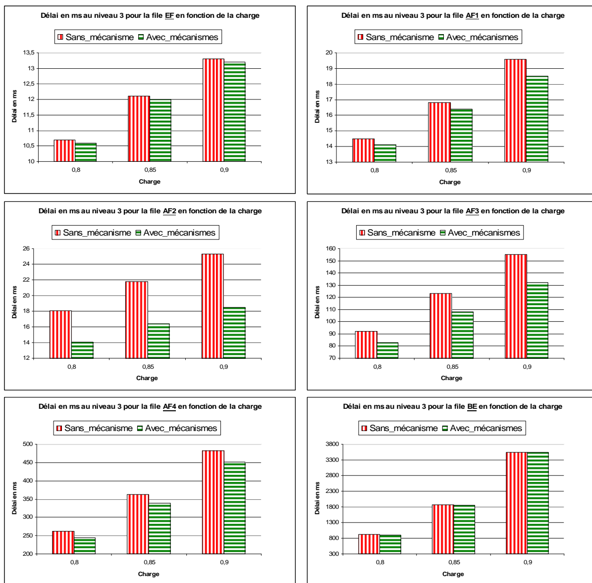
Figure 3-20: Délais dans les files de niveau 3
