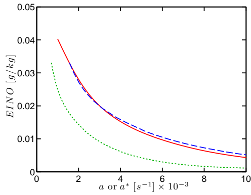
(c) Flame EINO.
