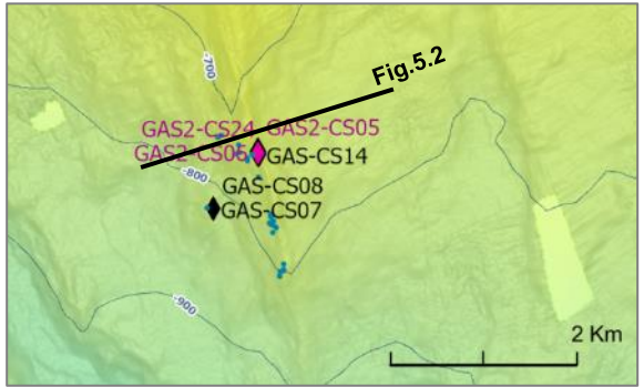
d- Zone de crête (zone à hydrates)
