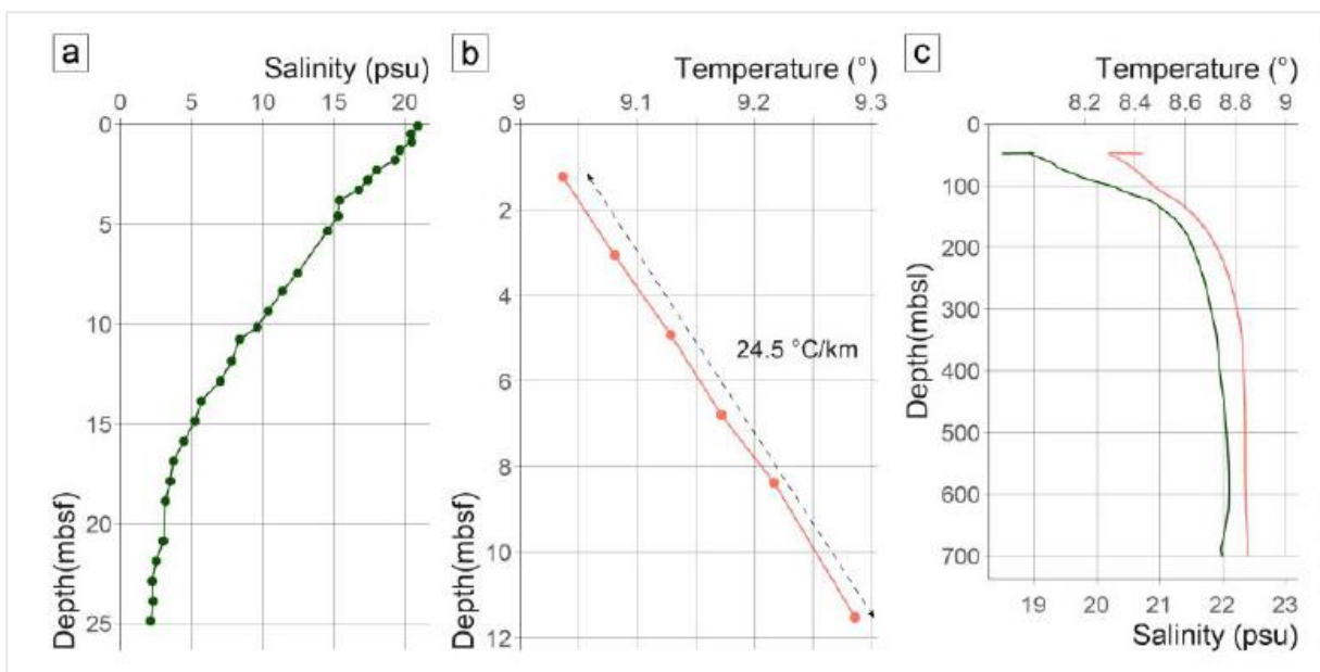
Figure 1.27: Profils des mesures réalisées in situ au cours de la campagne GHASS. (a) Profil de salinité dans les 25 premiers mètres de la colonne sédimentaire. (b) Gradient géothermique. (c) Evolution de la salinité et de la température dans la colonne d'eau (Riboulot et al., 2018).
