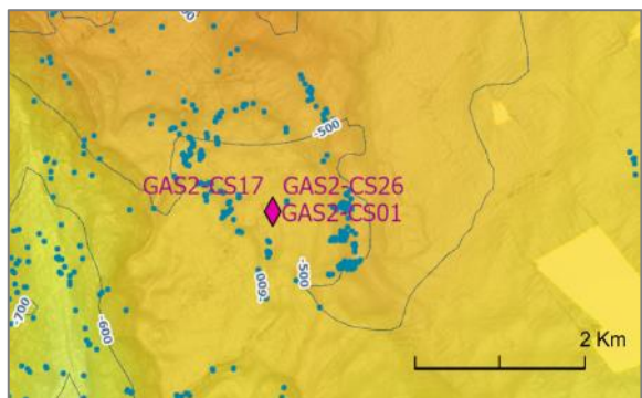
d- Zone de crête (zone à hydrates)
