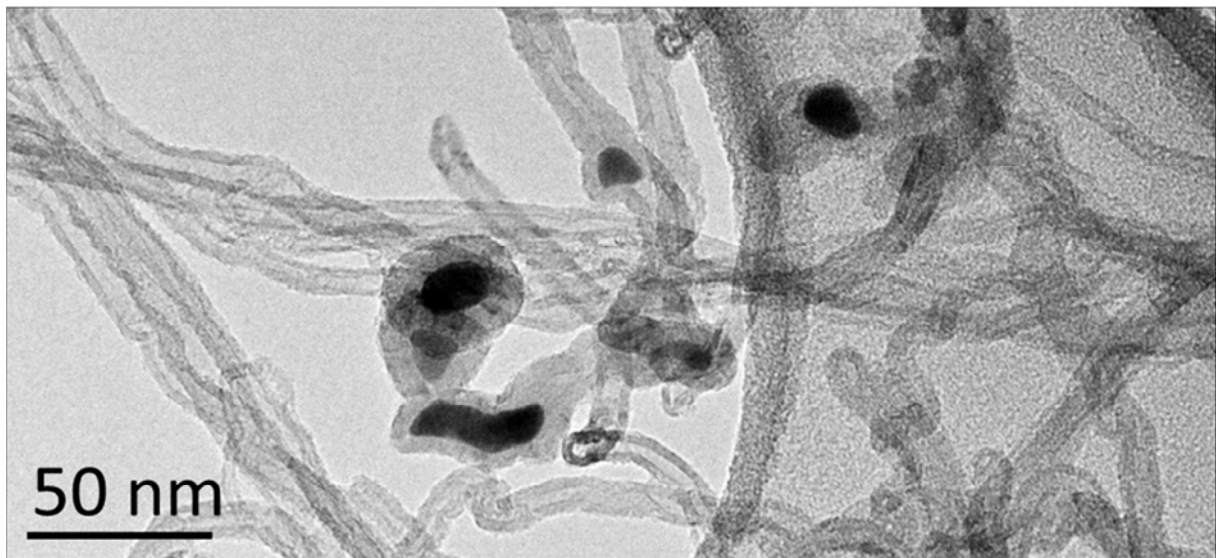
Figure 6 : Nanotubes de carbone multi-paroi (MWNTC) utilisés durant cette thèse. On peut remarquer sur la photo des nanoparticules métalliques issues de la synthèse (zones sombres) encapsulées dans des coques de carbone ou directement incluses dans les MWNTC. (Photo : L. Verneuil, EcoLab)
