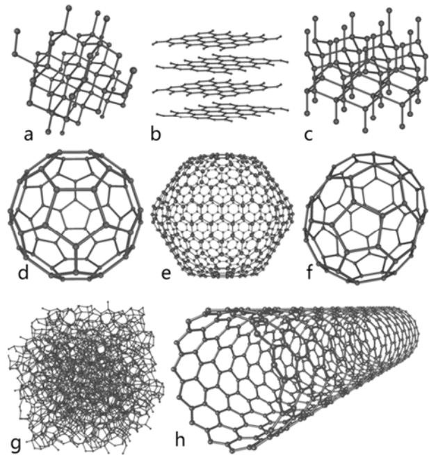
Figure 2 : Huit formes allotropiques du carbone présentes sur terre : (a) Diamant (hybridation sp^3 ), (b) Graphite (hybridation sp^2 ), (c) Lonsdaleite, Fullerènes (d) C60 (e) C540 (f) C70 (g) Carbone amorphe (h) Nanotube de carbone mono paroi. http://fr.wikipedia.org/wiki/Formes_allotropiques_du_carbone . Michael Ströck (mstroeck) 7 février 2006 (CC) BY-SA 3.0.
