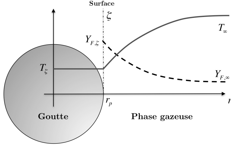
Figure 4.3 : Profil radial de la température T et de la fraction massique de carburant gazeux Y_F pour une goutte sphérique à température uniforme T_p = T_\xi (pas de stockage d'énergie à la surface).
