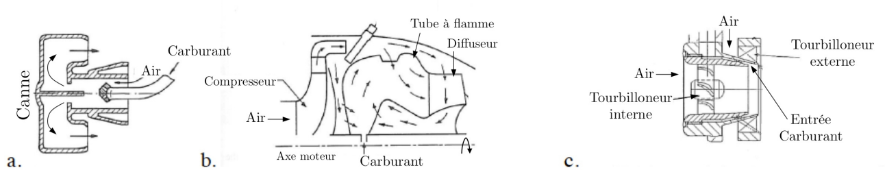
Figure 1.4 : Principaux types d'injecteurs utilisés dans les moteurs d'hélicoptères : à pré-vaporisation (a.), à roue centrifuge (b.), aéro-dynamique à préfilm (c.) (extraits de Lefebvre [126]).
