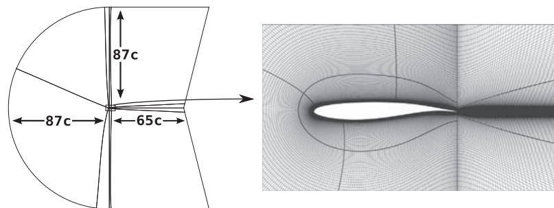
Fig. 4. Multiblock domain.
