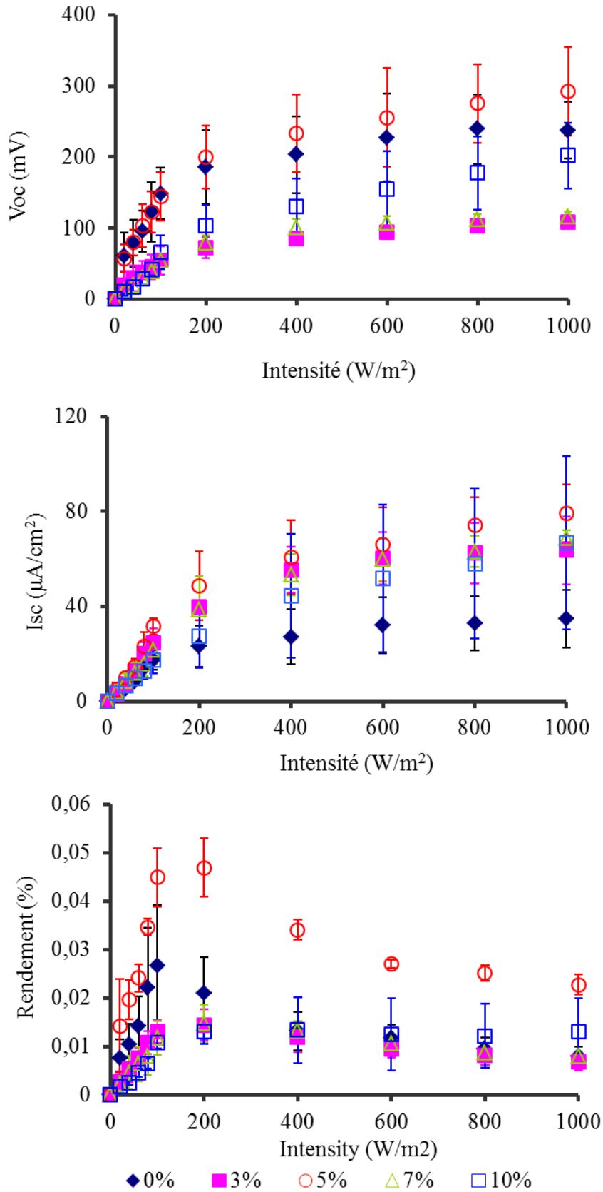
Figure 5.4: Les paramètres affectant les performances de la BSSC en utilisant les électrodes \text{TiO}_2 anatase-KCB2 avec les différentes concentrations de KCB2
