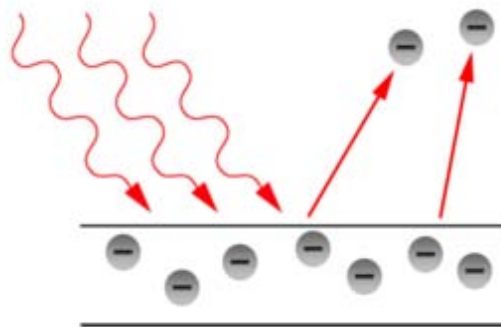
Figure 1.2: L'effet photovoltaïque, l'onde électromagnétique incidente éjecte les électrons du matériau
