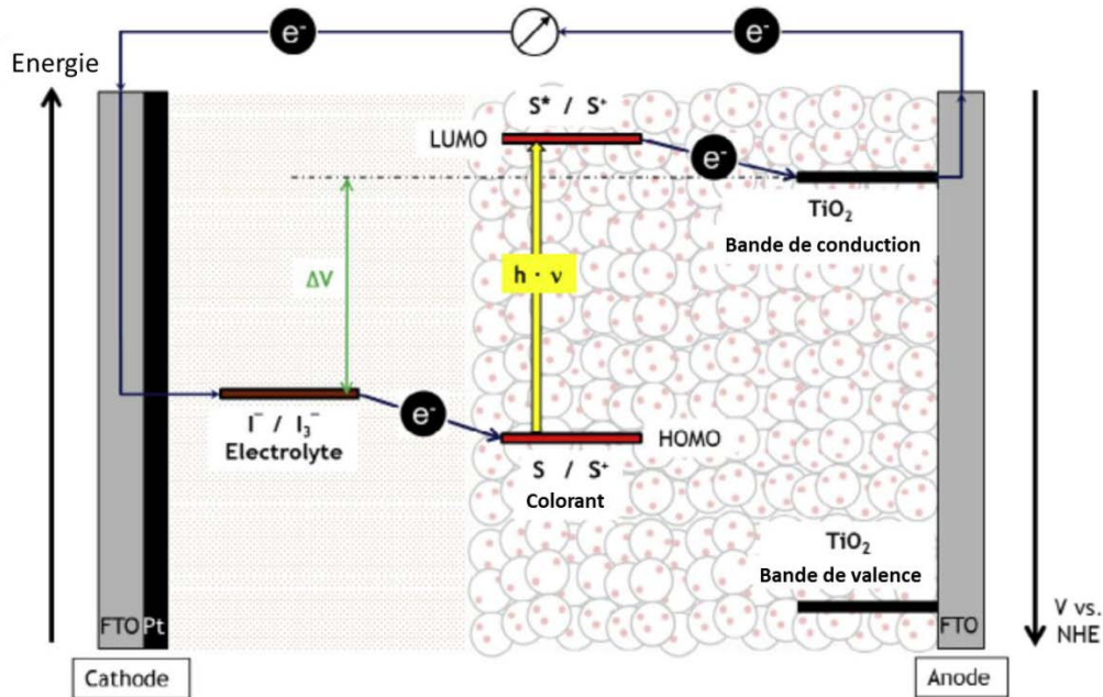
Figure 1.3: Principe de fonctionnement d'une CSSC [8]
