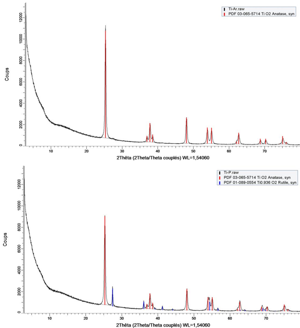
Figure 5.3: Les diagrammes de DRX de TiO 2 anatase et TiO 2 P25
