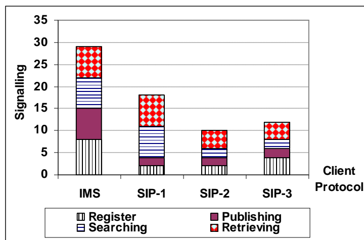
Figure 3.5.2-1: Poids de la signalisation côté client
