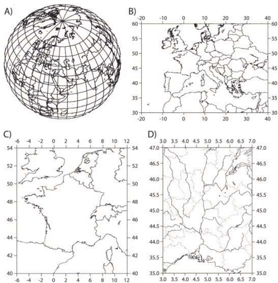
FIGURE 2.3 – Domaines MOCAGE de l'échelle globale à méso-échelle : (A) domaine "global" à 2° de résolution horizontale; (B) domaine "continental" à 1°; (C) domaine "régional" à 0.25°; et (D) domaine "zoom" à 0.08° (d'après Dufour et al. [2005]).
