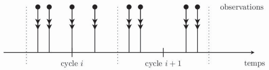
FIGURE 2.8 – Répartition des observations dans un 3D-FGAT d’après [Dajet, 2007]
