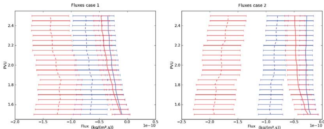
FIGURE 3.15 – Flux net d’ozone ( \text{kg m}^{-2} \text{s}^{-1} ) entre 1.5 PVU et 2.5 PVU à partir de MOCAGE sans assimilation (bleu) et des analyses MLS (rouge). La basse résolution ( 2^\circ ) et la haute résolution ( 0.2^\circ ) sont représentées par les lignes en tirets et pleines, respectivement. A gauche, Cas d’étude 1 : les flux sont estimés du 20 Juin 2009, 06 :00 UT au 24 Juin 2009, 18 :00 UT. A droite, Cas d’étude 2 : les flux sont estimés du 16 Juillet 2009, 06 :00 UT au 19 Juillet 2009, 18 :00 UT. Les barre d’erreur représentent la déviation standard divisée par la racine carrée du nombre de points de grille. Cela donne la limite inférieure de l’estimation de l’erreur car on ne tient pas compte de la corrélation entre les points de grille.
