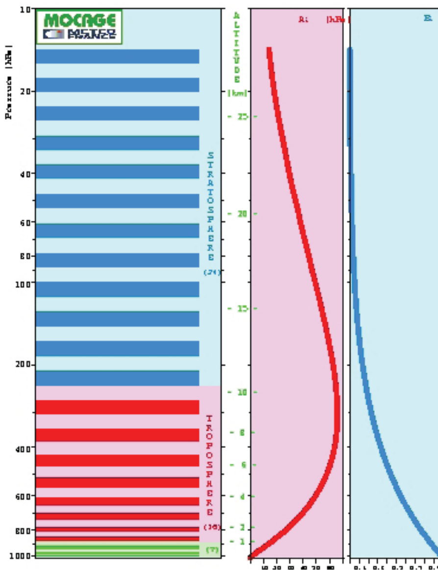
FIGURE 2.5 – Les 47 niveaux verticaux hybrides (\sigma, P) dans la version standard du modèle MOCAGE . A gauche le découpage de l’atmosphère en 47 couches, à droite les coefficients A_i et B_i permettant de calculer la pression de chaque niveau i suivant la formule A_i + B_i \cdot P_s , avec P_s la pression de surface.
