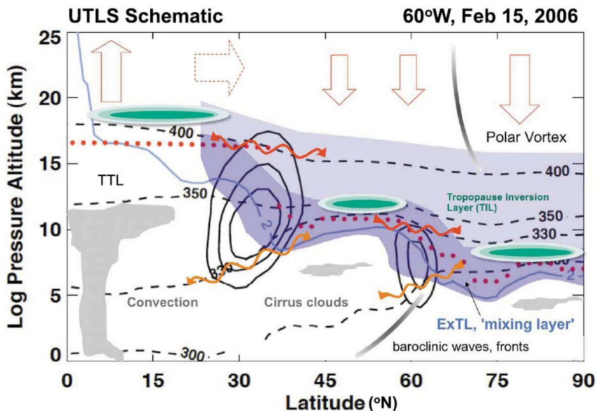
FIGURE 1.5 – Représentation schématique de l’UTLS extra-tropicale de l’hémisphère Nord sur la longitude 60°W le 15 Février 2006. Les contours de vents (lignes noires par intervalles de 10m.s -1 ), les surfaces de température potentielle (lignes noires en tirets), la tropopause thermique (points rouges), et la tropopause dynamiques (ligne bleu claire) sont représentés. La région en bleu clair représente l’UTLS extra-tropicale, en bleu foncé la couche de transition, en vert les maxima de stabilité verticale et en gris les nuages et les fronts. Les flèches rouge et oranges ondulés montrent les échanges quasi-isentropiques qui, respectivement franchissent ou non la tropopause. Les flèches rouges plus larges montrent la circulation stratosphérique moyenne de Brewer-Dobson (d’après Gettelman et al. [2011]).
