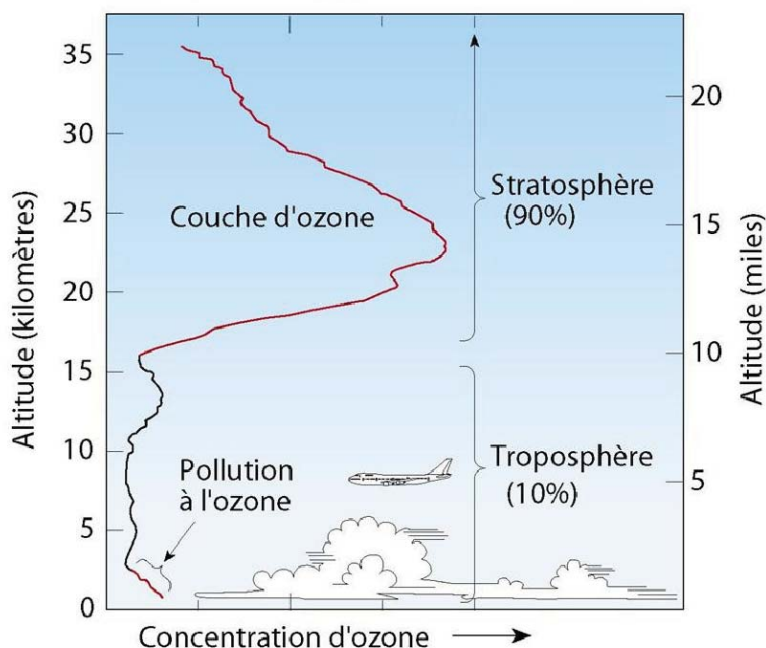
FIGURE 1.2 – Distribution verticale de l'ozone dans la troposphère et la stratosphère.
