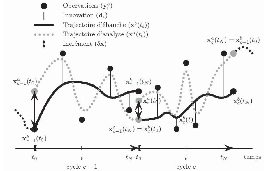
FIGURE 2.7 – Principe de la technique variationnelle du schéma 4D-VAR d’après [Dajet, 2007].
