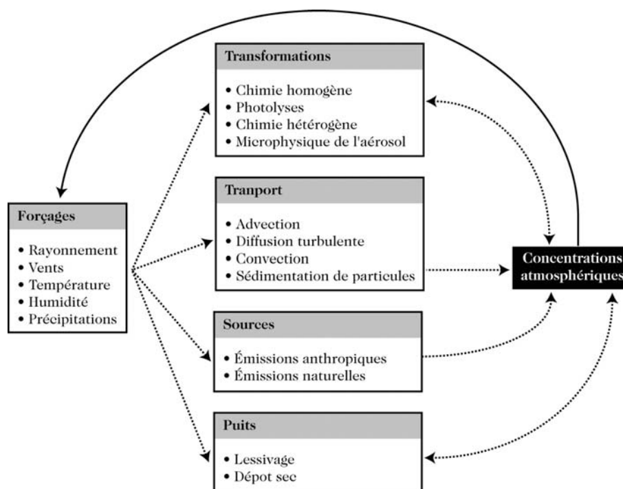
FIGURE 2.1 – Principaux processus physico-chimiques mis en jeu pour la modélisation numérique de la composition chimique de l’atmosphère d’après Delmas et al. [2005]
