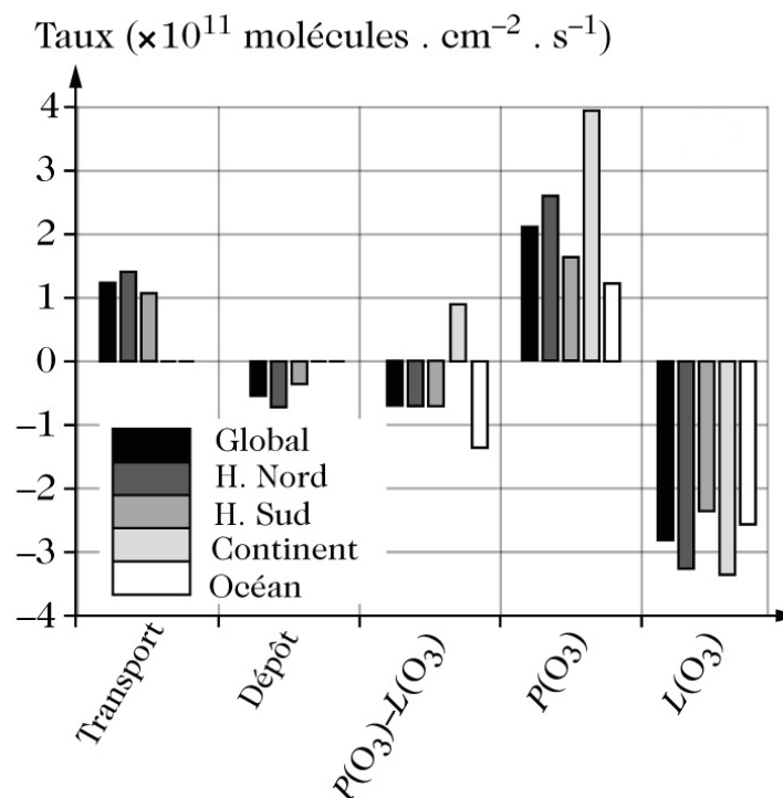
FIGURE 1.9 – Composantes du bilan de l'ozone troposphérique qui incluent le transport depuis la stratosphère et le transport inter-hémisphérique, le dépôt au sol et la production chimique nette P(\text{O}_3) - L(\text{O}_3) (production moins destruction). Figure d'après Delmas et al. [2005] et Crutzen et al. [1999].
