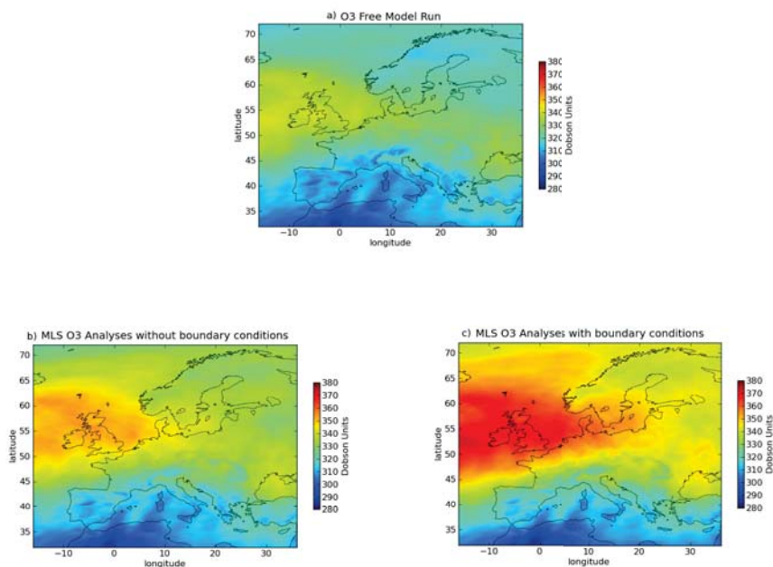
FIGURE 2.11 – Champs moyens de la colonne totale d'ozone (Unités Dobson) pour les Run 1 (a), Run 2 (b) et Run 3 (c) au dessus de l'Europe entre le 10 Juillet 2009 et le 25 Juillet 2009.
