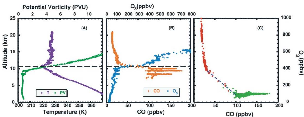
FIGURE 1.6 – Profils issus de mesures aéroportés montrant la region de transition dynamique et chimique au niveau de la tropopause. La tropopause thermique est représentée en pointillées (d'après Pan et al. [2004]).
