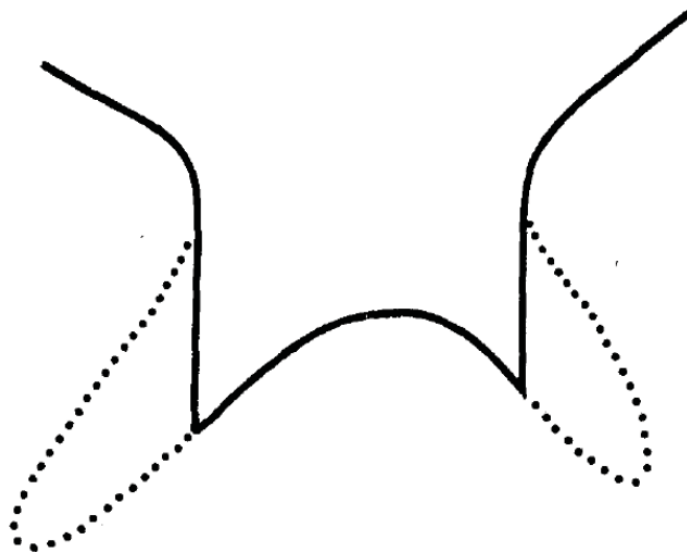
FIGURE 3.14 – Diagramme schématisant la méthode pour définir la tropopause (trait plein) dans le cas de multiples tropopauses (pointillés) sur la verticale. Cette condition tronque les foliations de tropopause à leur origine (d'après Wei [1987]).
