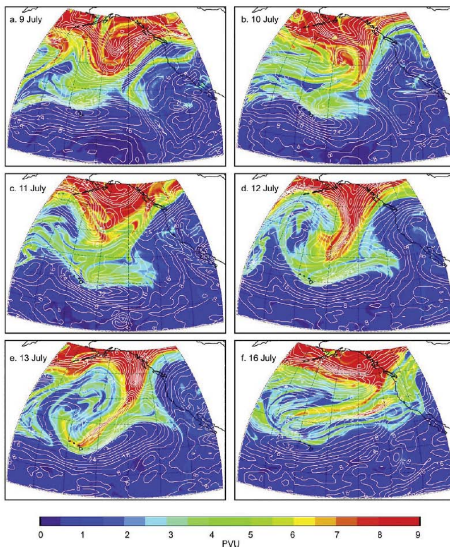
FIGURE 1.7 – Evolution de la PV sur 7 jours au dessus du pacifique nord sur le niveau isentropique 350 K. Au cours du déferlement des ondes de Rossby, les fortes valeurs de PV stratosphériques montrent s'étendent vers l'équateur sous formes de filaments (d'après Leblanc et al. [2004]).
