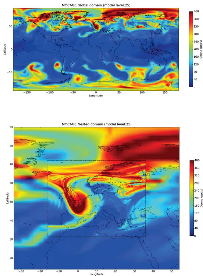
FIGURE 2.14 – Champs d’ozone au niveau modèle 25 (qui se situe entre 200 et 300 hPa) pour le domaine global (haut) et le domaine imbriqué (bas) le 17 juillet 2009 à 15 :00 UT. Les champs d’ozone montrent l’expérience du Run3, où les données MLS ont été assimilées dans le domaine global et dans le domaine imbriqué.
