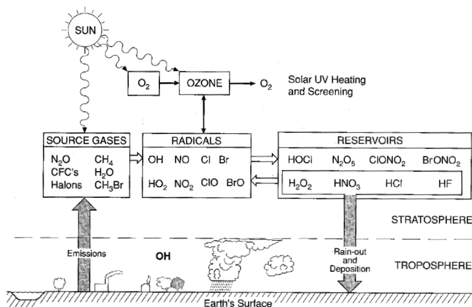
FIGURE 1.3 – Schéma de principe de la chimie de l'ozone stratosphérique (d'après Brasseur et al. [1999])
