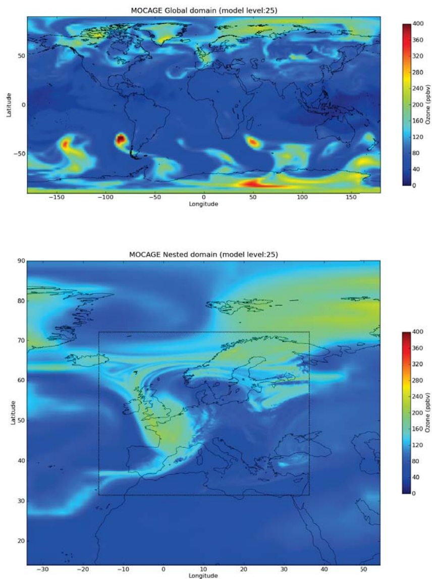
FIGURE 2.4 – Champs d’ozone au niveau modèle 25 (qui se situe entre 200 et 300 hPa) pour le domaine global (haut) et le domaine imbriqué (bas) le 17 juillet 2009 à 15 :00 UT. La concordance des champs entre le domaine global et le domaine imbriqué illustrent le “two-ways nesting”.
