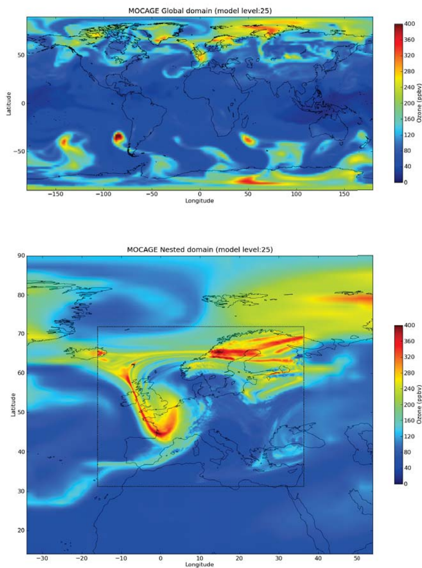
FIGURE 2.13 – Champs d’ozone au niveau modèle 25 (qui se situe entre 200 et 300 hPa) pour le domaine global (haut) et le domaine imbriqué (bas) le 17 juillet 2009 à 15 :00 UT. Les champs d’ozone montrent l’expérience du Run2, où les données MLS ont été assimilées seulement dans le domaine imbriqué.
