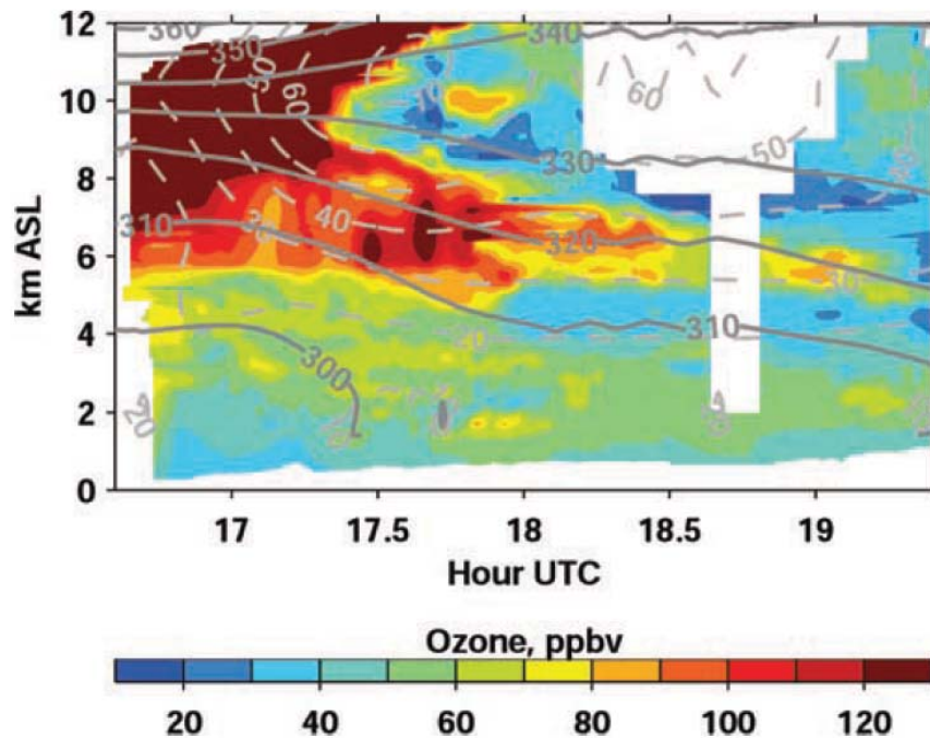
FIGURE 1.8 – Distribution verticale de l'ozone obtenue à partir d'un LiDAR aéroporté. Le vol traverse les États-Unis du nord vers le sud et montre un évènement STE. Les lignes grises en trait plein sont les températures potentielles (K), les lignes grises pointillées est la vitesse du vent en \text{m.s}^{-1} (d'après Wimmers et al. [2003]).
