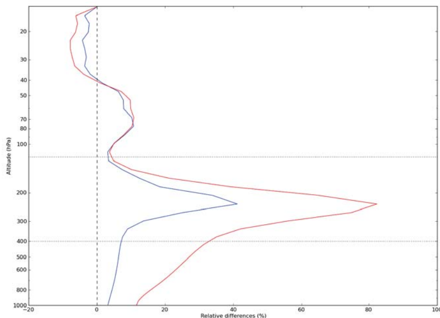
FIGURE 2.12 – Profil des différences relatives moyennées sur le domaine régional entre Run1 et Run2 (bleu) et entre Run1 et Run3 (rouge). Un maximum de différence est observé au niveau de l’UTLS entre 400 et 120 hPa.
