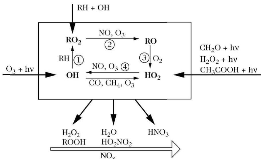
FIGURE 1.4 – Schéma des sources, des puits et des inter-conversions chimiques rapides des radicaux HO_x . Le cycle constitué par les réactions 1, 2, 3 et 4 produit ou détruit de l'ozone en fonction des concentrations de NO présentes dans l'atmosphère (d'après Delmas et al. [2005]).
