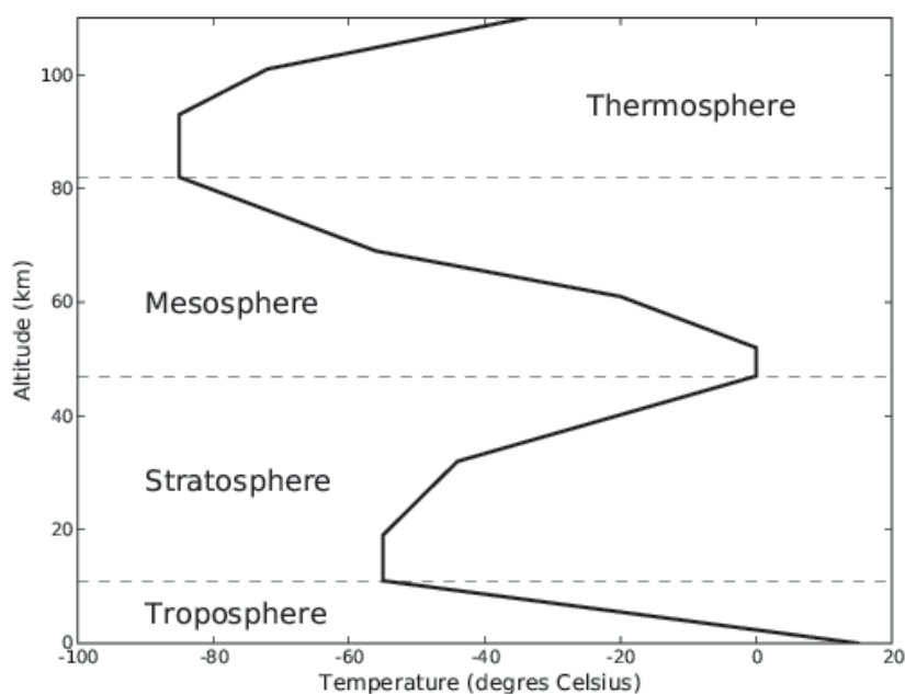
FIGURE 1.1 – Profil de température dans l'atmosphère en °C.
