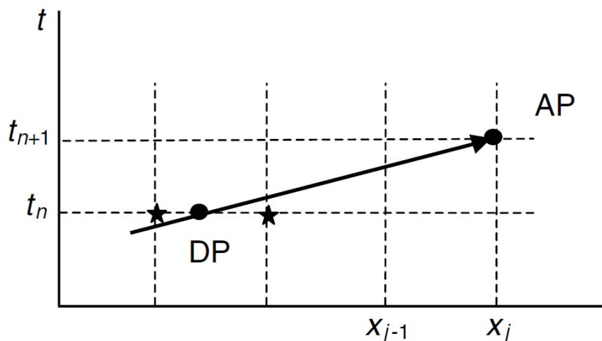
FIGURE 2.2 – Diagramme schématisant le schéma semi-lagrangien. AP (arrival point) représente le point d’arrivée au nouveau pas de temps. DP (departure point) représente le point de départ au précédent pas de temps. La flèche représente l’advection depuis DP jusqu’à AP (d’après Kalnay [2003]).
