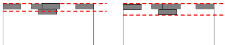
Figure III-20 : Schématisation de la quantification de l'endommagement induit par des phénomènes de corrosion de l'alliage 2050-T34, PT dans une solution NaCl 0,7M (a) profondeur moyenne atteinte par la corrosion intragranulaire (b) profondeur maximale atteinte par la corrosion intragranulaire.
