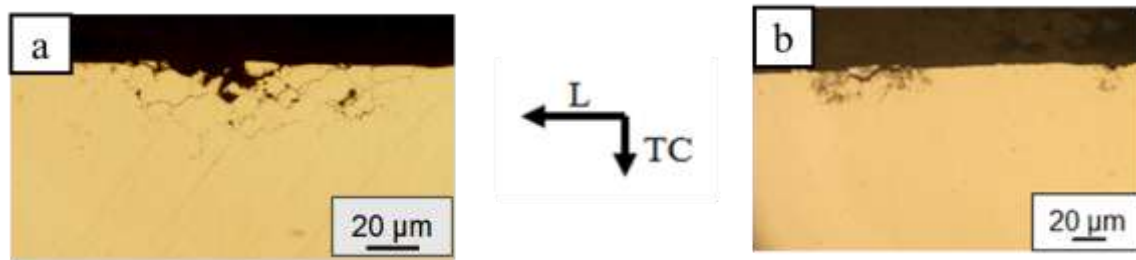
Figure V- 5: Observation en coupe du plan L-TC (a) du Noyau soudé T34 OPT et (b) du Noyau soudé T34 OPT post traité après 3 jours d'immersion dans une solution de NaCl 0,7 M à 25 °C.
