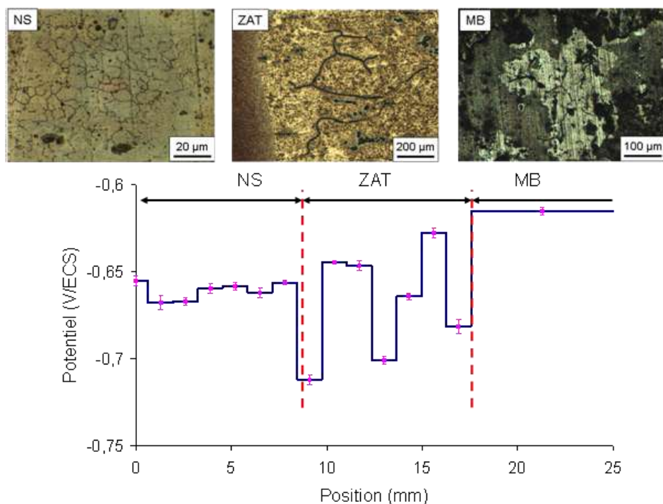
Figure IV-24 : En haut : observations des échantillons après les mesures de potentiel libre (OCP) réalisées dans une solution NaCl 0,7 M à 25 °C. En bas : évolution du potentiel libre dans le joint soudé T34 OPT à 1,5 mm sous la surface supérieure.
