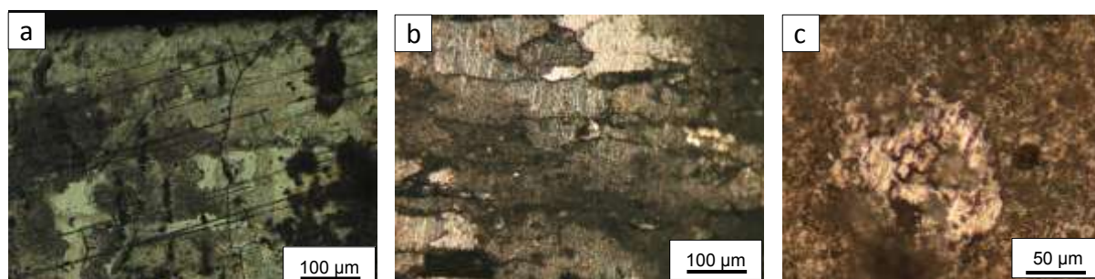
Figure IV-47: Observations au microscope optique dans le plan L-TL (a) du métal de base, (b) de la ZAT et (c) du noyau soudé du joint soudé T34 OPT après un essai de corrosion sous contrainte réalisé sur le joint soudé complet durant 3 jours dans une solution à 0,7 M de NaCl thermostatée à 25 °C.
