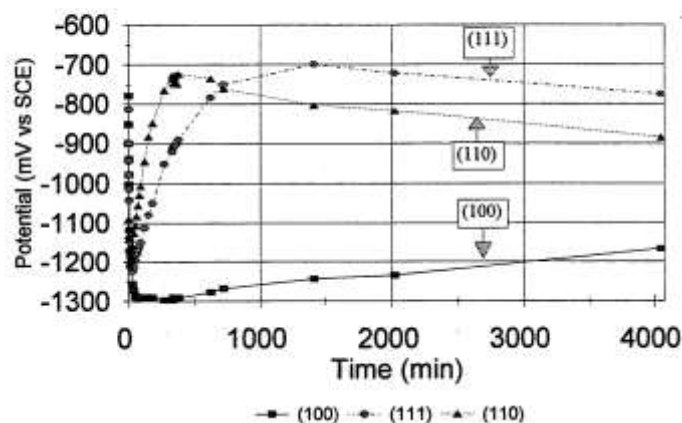
Figure V- 11: évolution de l'OCP d'un monocristal d'aluminium en fonction de l'orientation cristallographique des grains exposés à l'électrolyte pour une solution de NaCl à 3,5 % [124].
