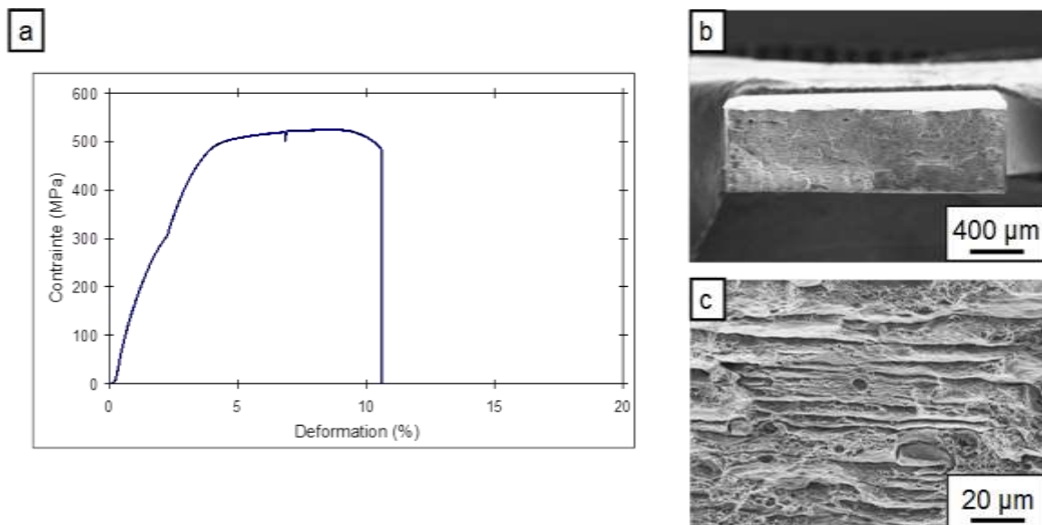
Figure III-17 : (a) Courbe de traction conventionnelle pour un échantillon de l'alliage 2050-T34, PT sollicité suivant la direction L (b) Micrographie MEB représentant la section rompue de l'éprouvette après l'essai de traction (c) Micrographie MEB d'une zone du faciès de rupture à fort grandissement.
