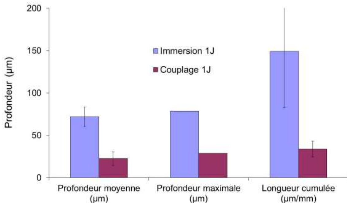
Figure IV-39 : Quantification de l'endommagement du métal de base du joint soudé T34 OPT après un jour d'immersion dans une solution NaCl 0,7 M. Le métal de base est soit immergé individuellement dans l'électrolyte soit couplé avec le noyau soudé du joint T34 OPT.
