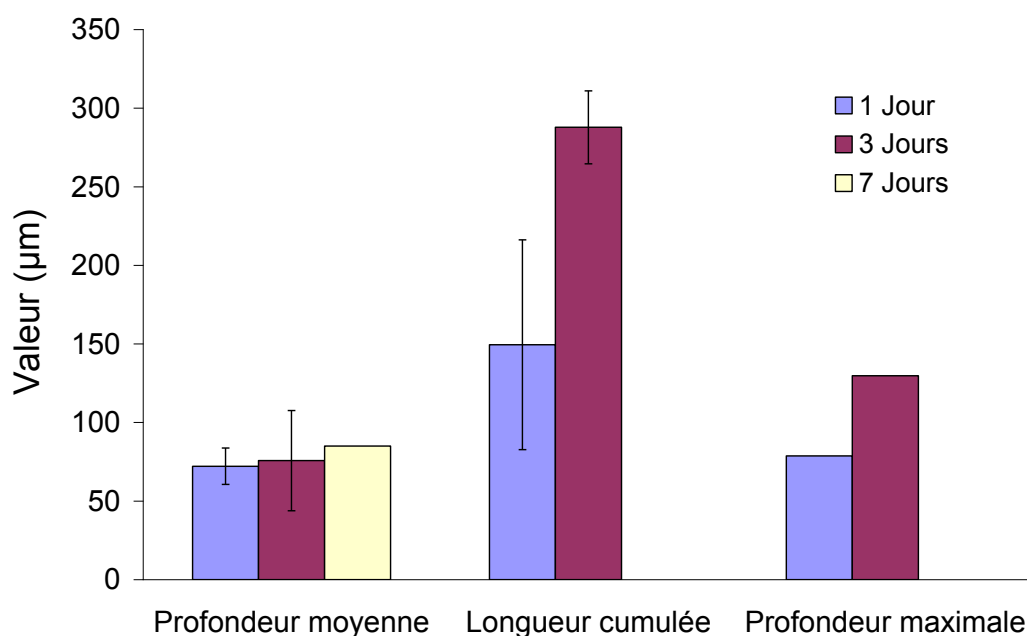
Figure III-8 : Grandeurs caractéristiques associées à l'endommagement en corrosion intergranulaire de l'alliage 2050-T34 prélevé au centre de la tôle après 1 jour, 3 jours et 7 jours d'immersion dans une solution NaCl 0,7 M thermostaatée à 25°C.
