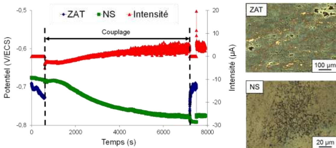
Figure IV-36 : Mesure du courant de couplage galvanique entre le NS et la ZAT du joint soudé T34 OPT prélevés à mi- épaisseur dans une solution NaCl 1M à 22 °C -Micrographies des électrodes de NS et de ZAT à l'issue de l'essai de couplage.
