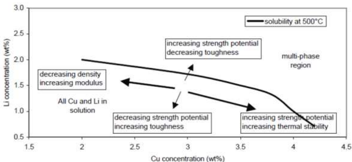
Figure I-10 : Influence de l'ajout de cuivre et de lithium sur les propriétés mécaniques des alliages Al-Cu-Li [31].
