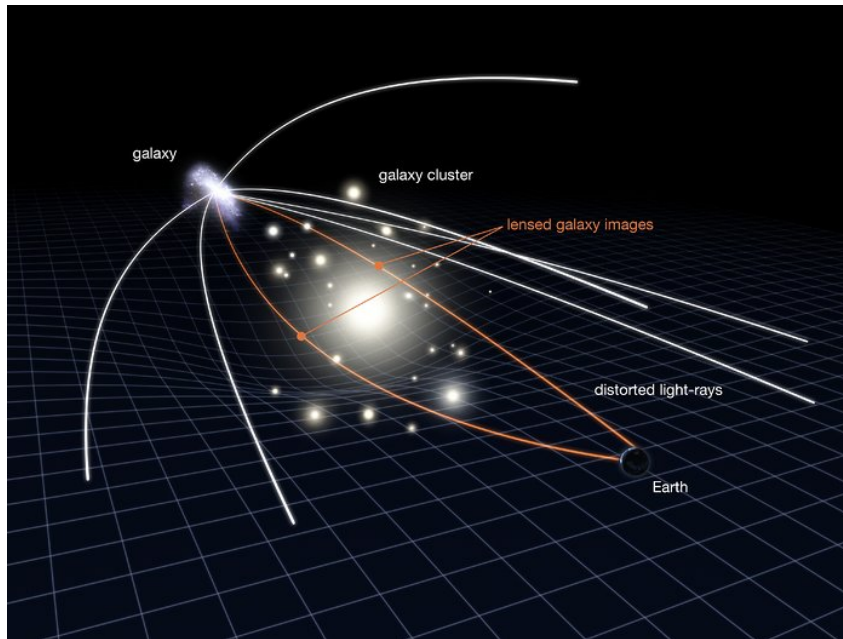
Figure 1.3. Illustration of gravitational lensing (Image: NASA, ESA & L. Calçada).
